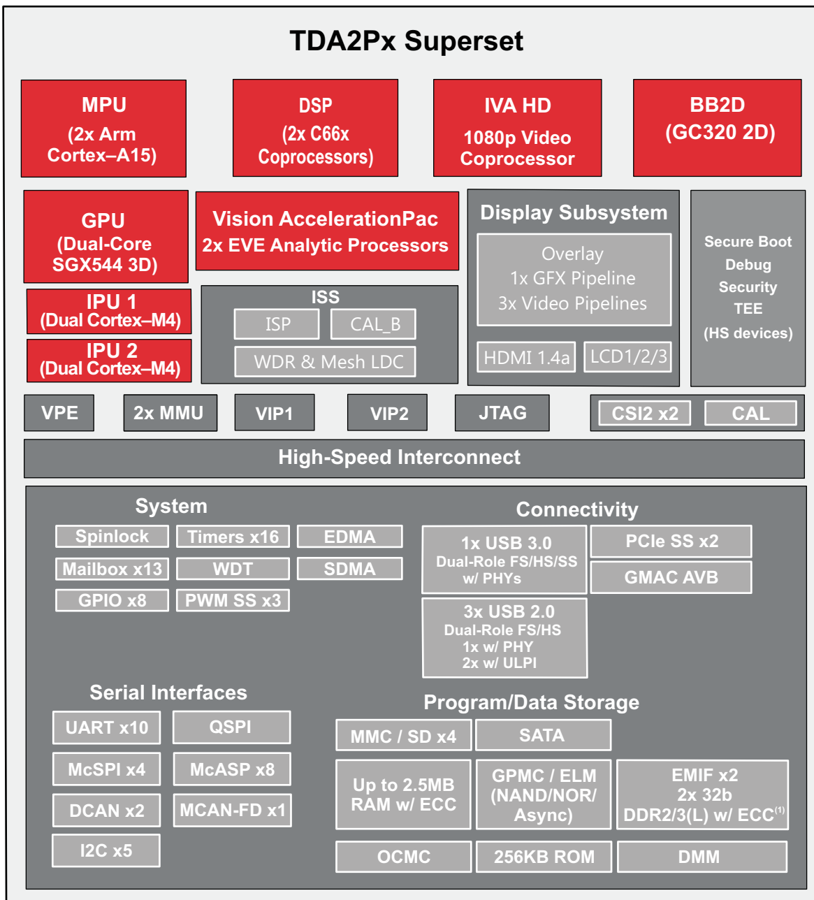
图 1-1. TDA2Px 方框图
