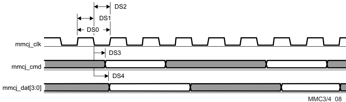
图 7-76. MMC/SD/SDIOj in - Default Speed - Transmitter Mode
