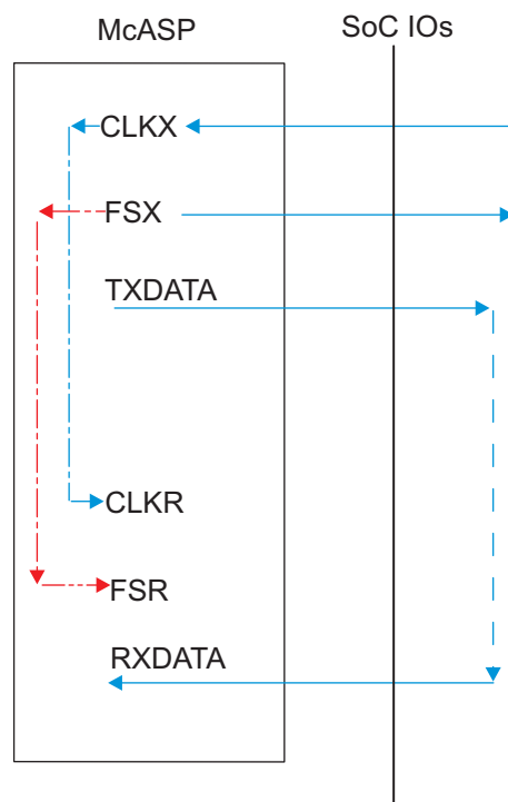
图 7-41. McASP1-8 CI-FO- – SYNC Mode
