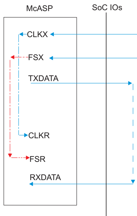
图 7-42. McASP1-8 CI-FI- – SYNC Mode
