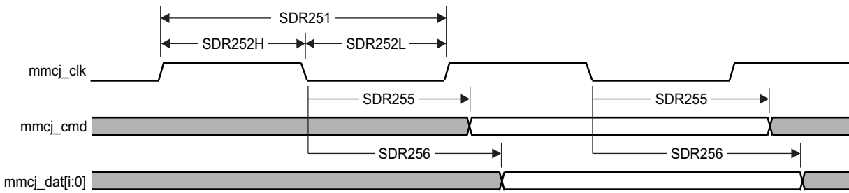
图 7-82. MMC/SD/SDIOj in - SDR25 - Transmitter Mode
