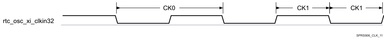
图 6-13. rtc_osc_xi_clkin32 Input Clock
