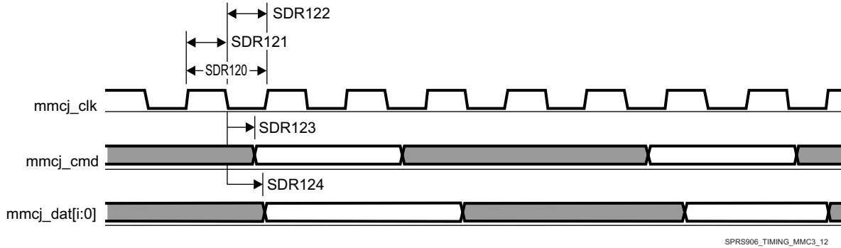
图 7-80. MMC/SD/SDIOj in - SDR12 - Transmitter Mode
