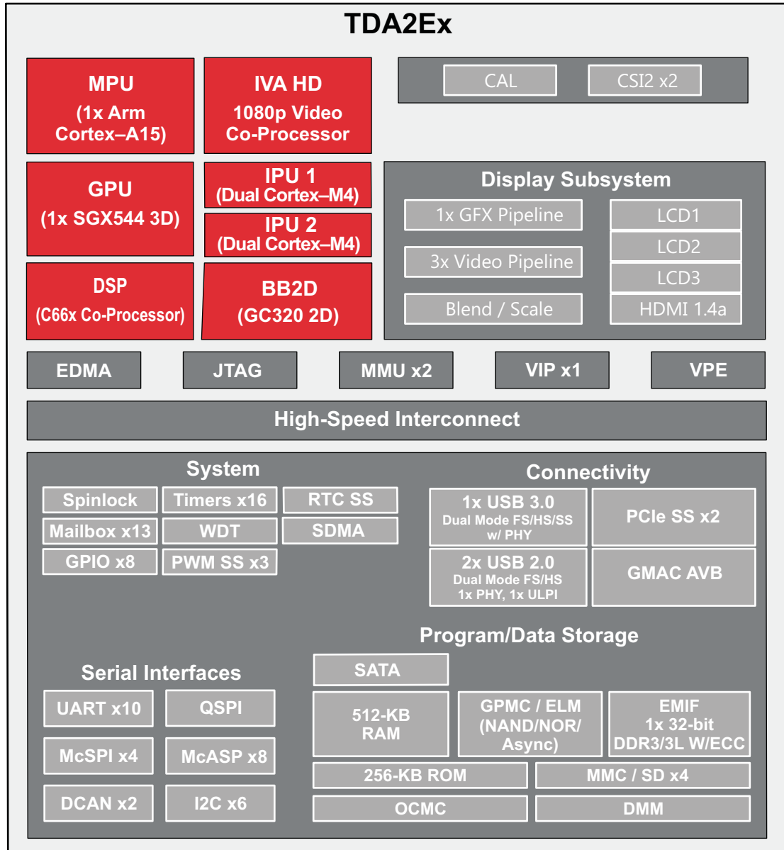
图 1-1. TDA2Ex 框图
