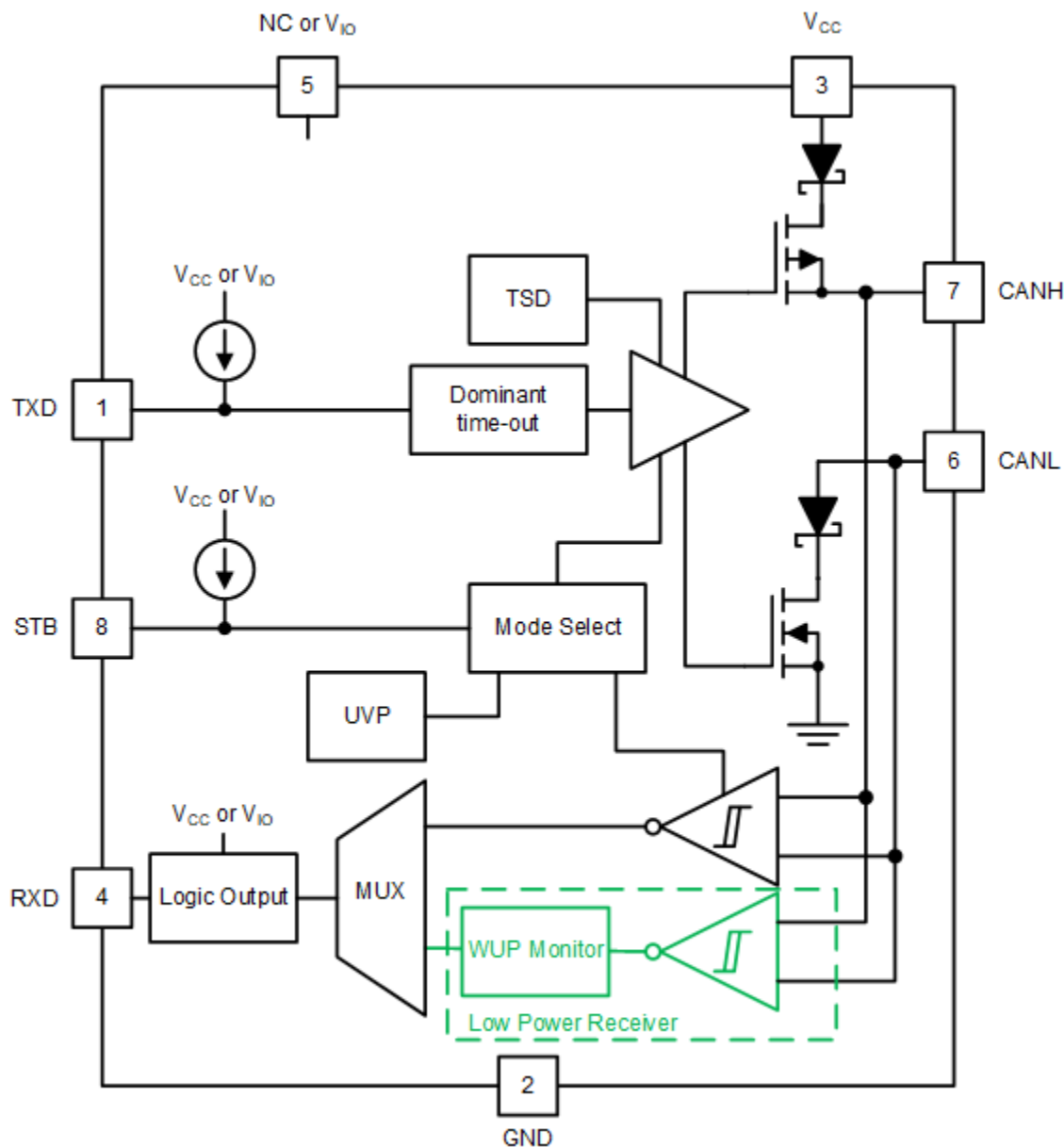
图 7-1. 方框图
