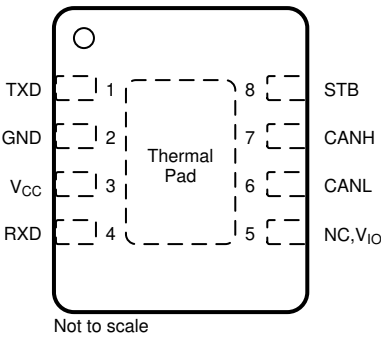
图 4-3. DRB 封装，8 引脚 VSON (顶视图)
