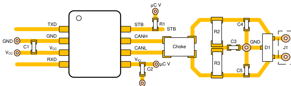
图 8-6. 布局示例
