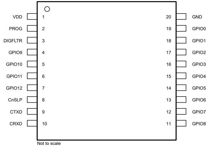
图 4-1. DGQ 20-PIN ( 顶视图 )
