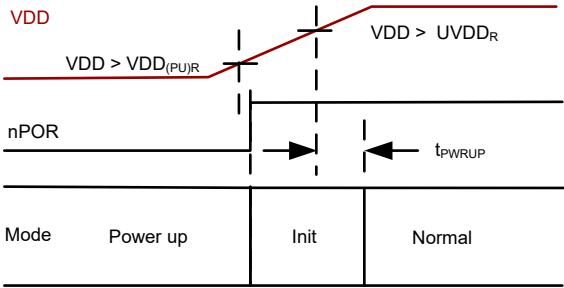
图 6-1. 上电时序
