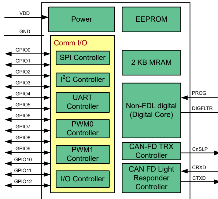
图 7-1. 高级方框图
