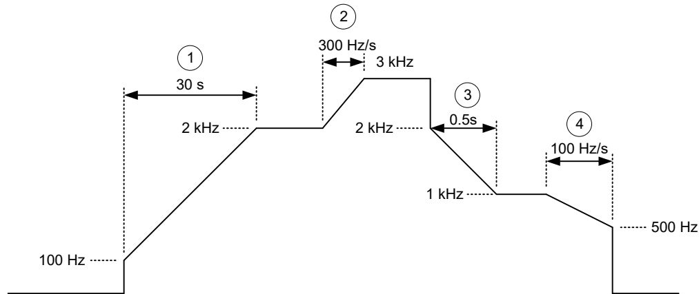
图 7-17. PWM 开关频率斜坡示例
