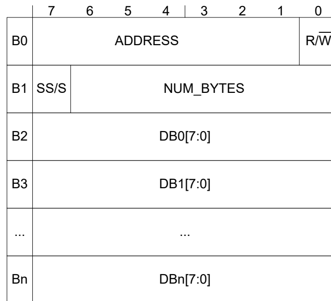
图 7-117. I2C 发送 FIFO
