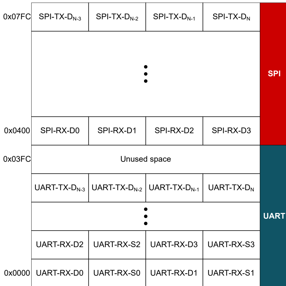
图 7-6. MRAM 布局示例 ( SPI 和 UART 启用 , 各占 50% )
