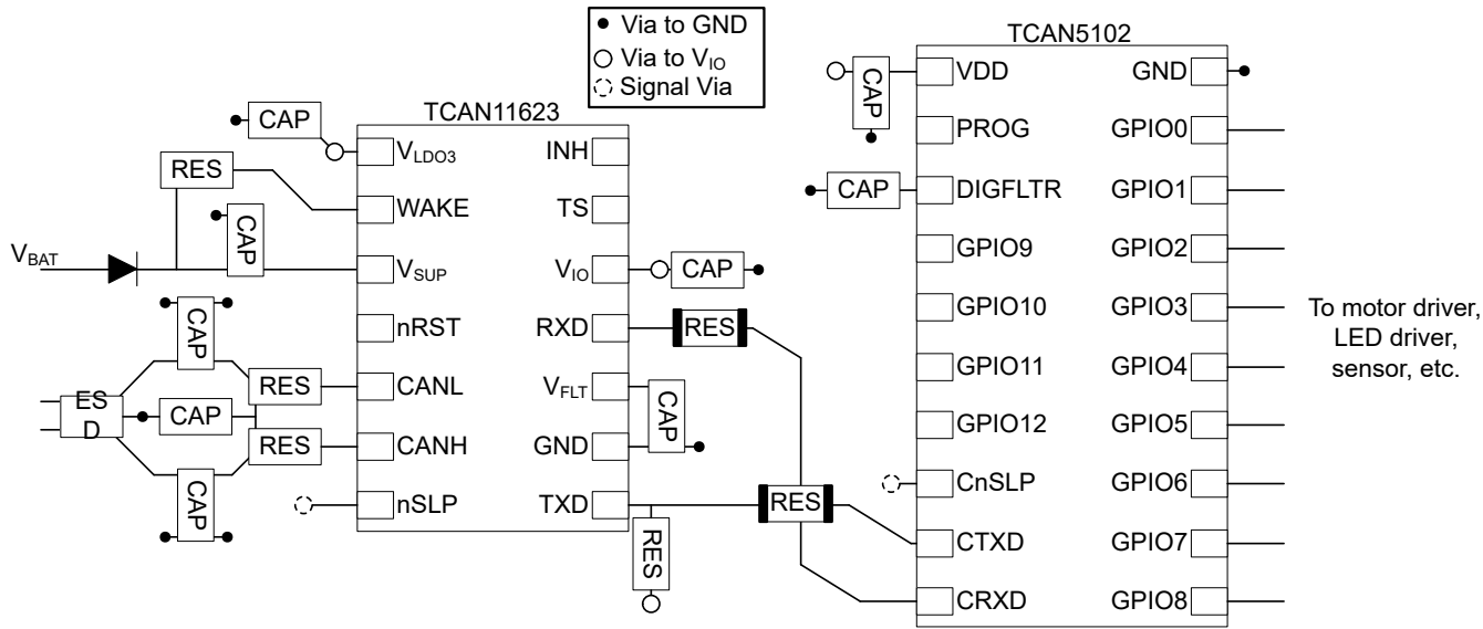
图 8-2. 布局示例
