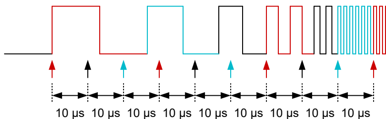
图 7-10. 开关频率斜坡更新
