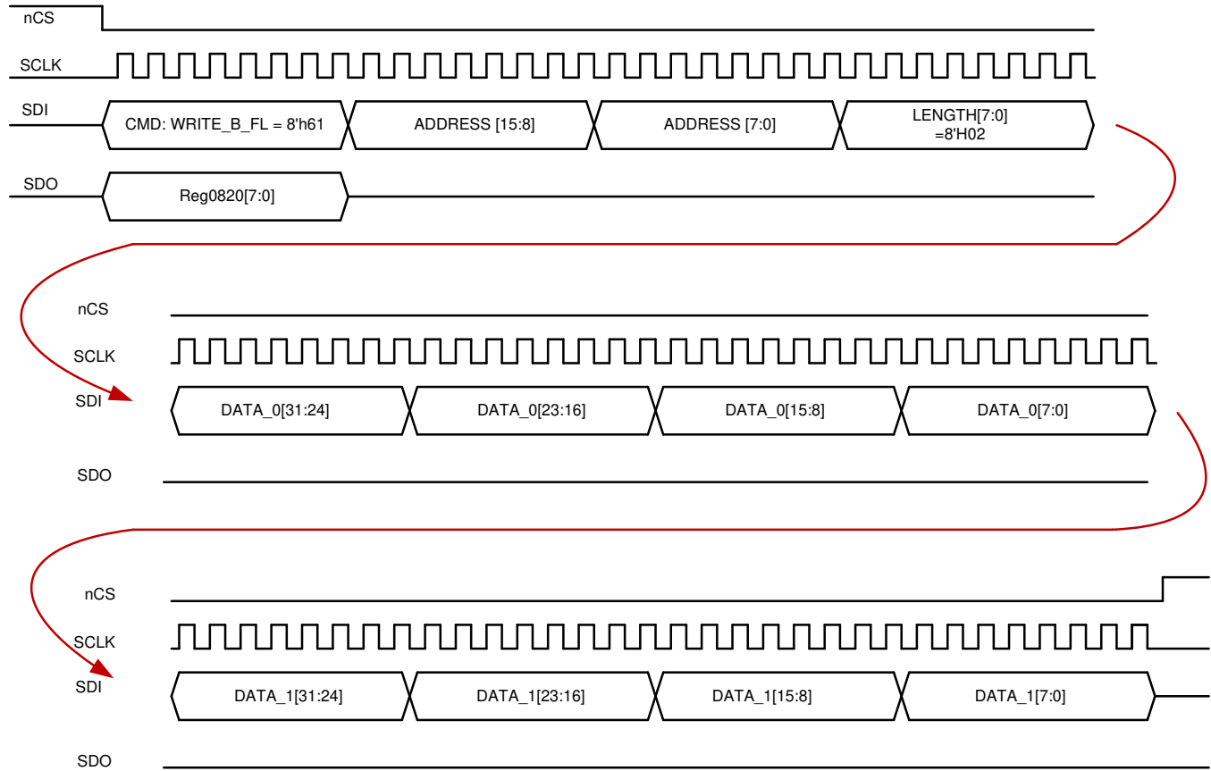
图 34. Write
