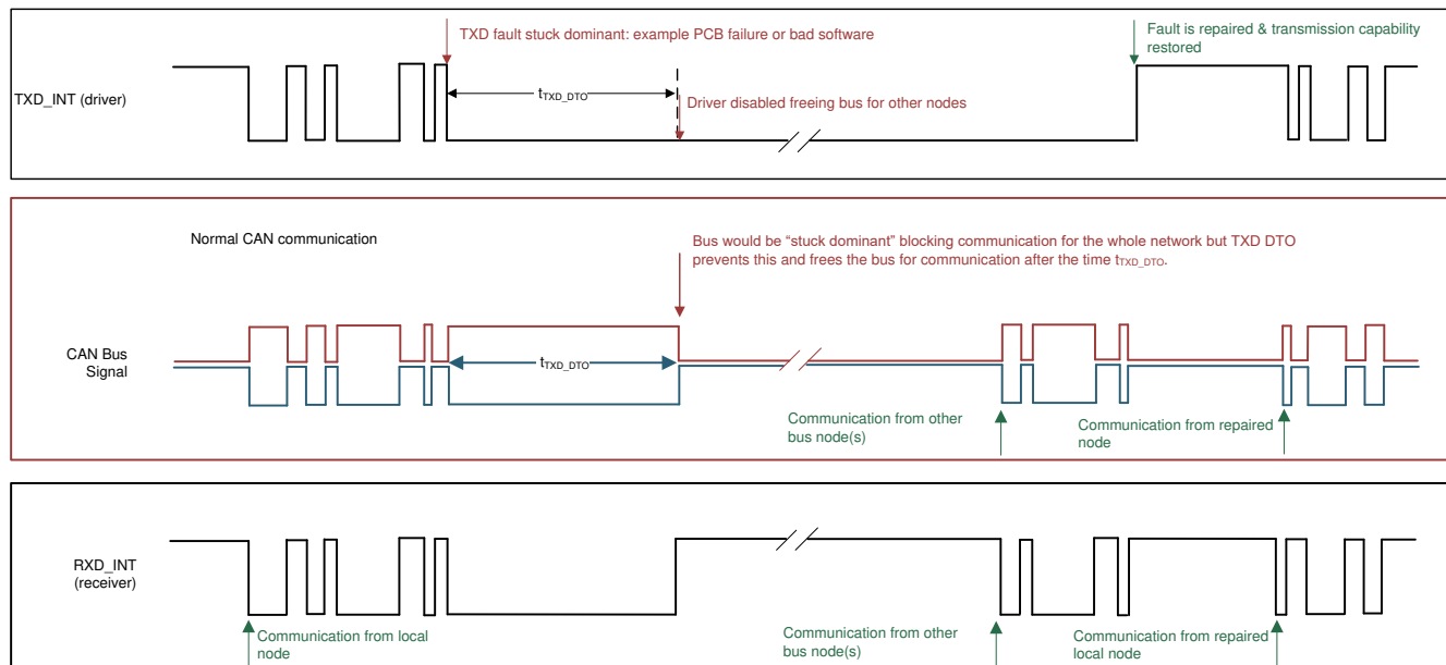
图 8-7. Example timing diagram with TXD_INT DTO
