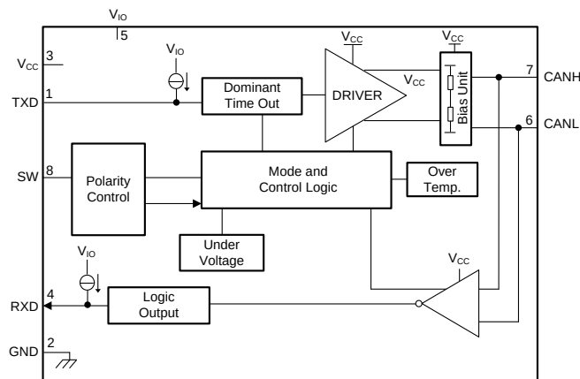
功能框图
