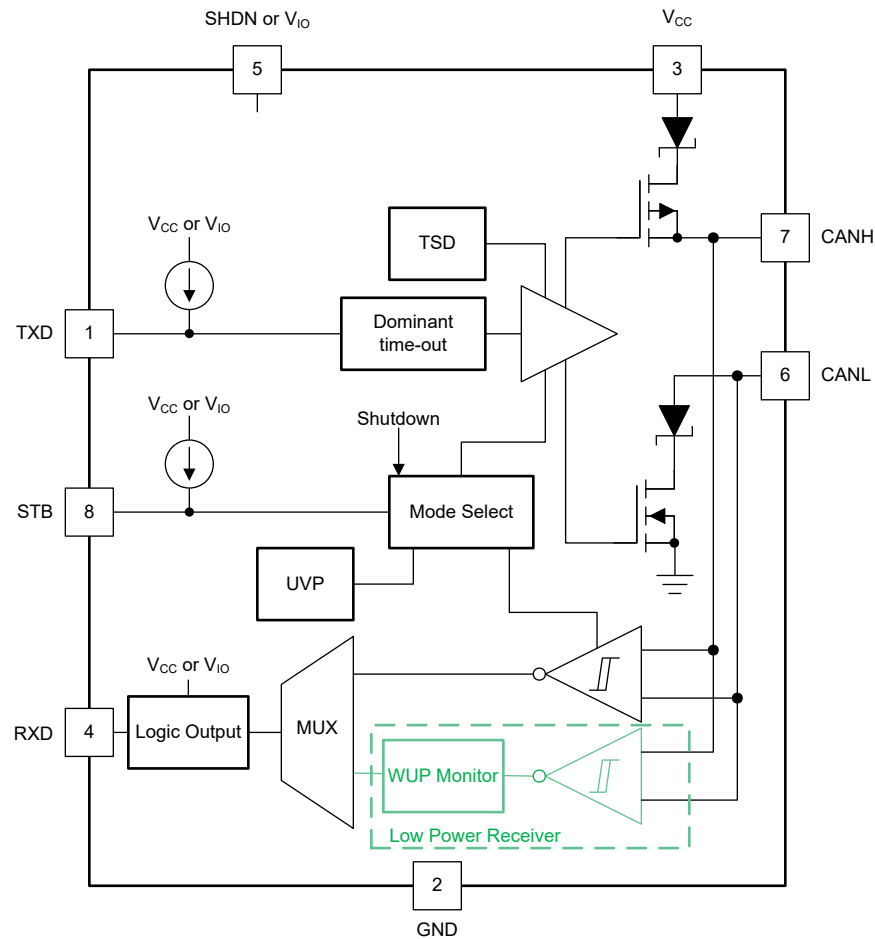
图 8-1. Block Diagram
