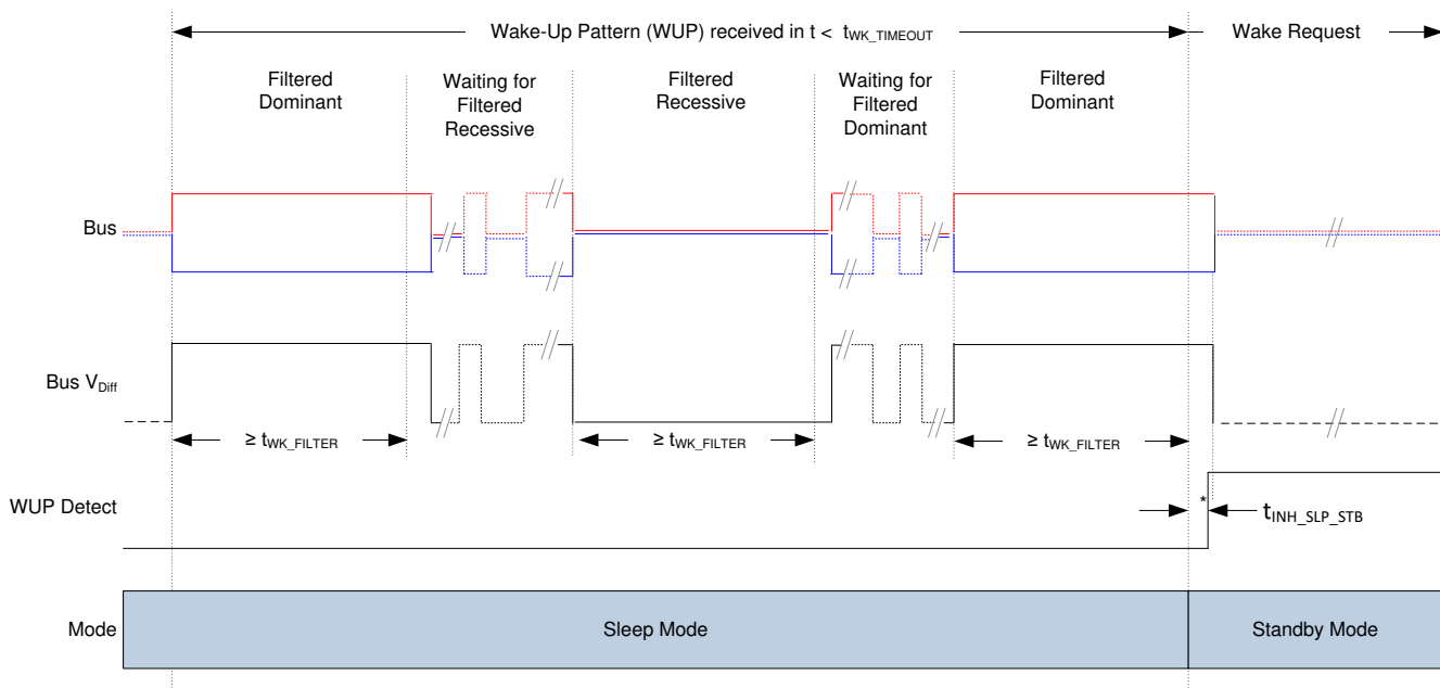
图 7-6. 唤醒模式 (WUP)
