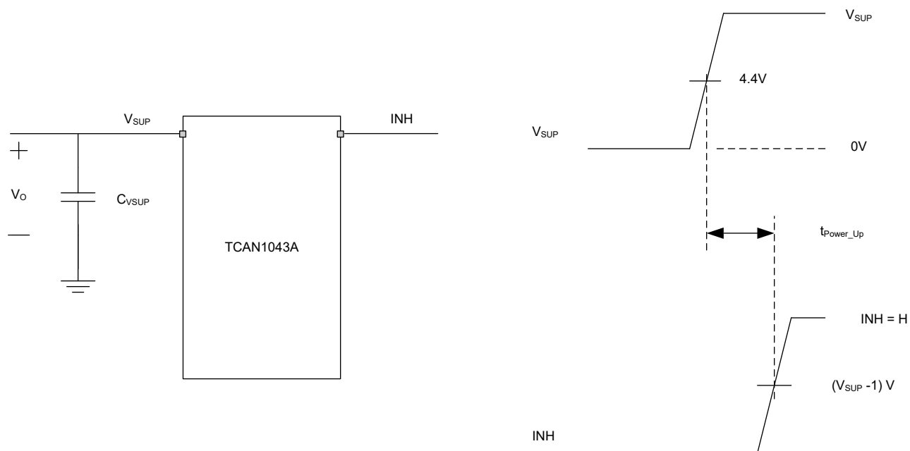
图 6-12. 上电时序
