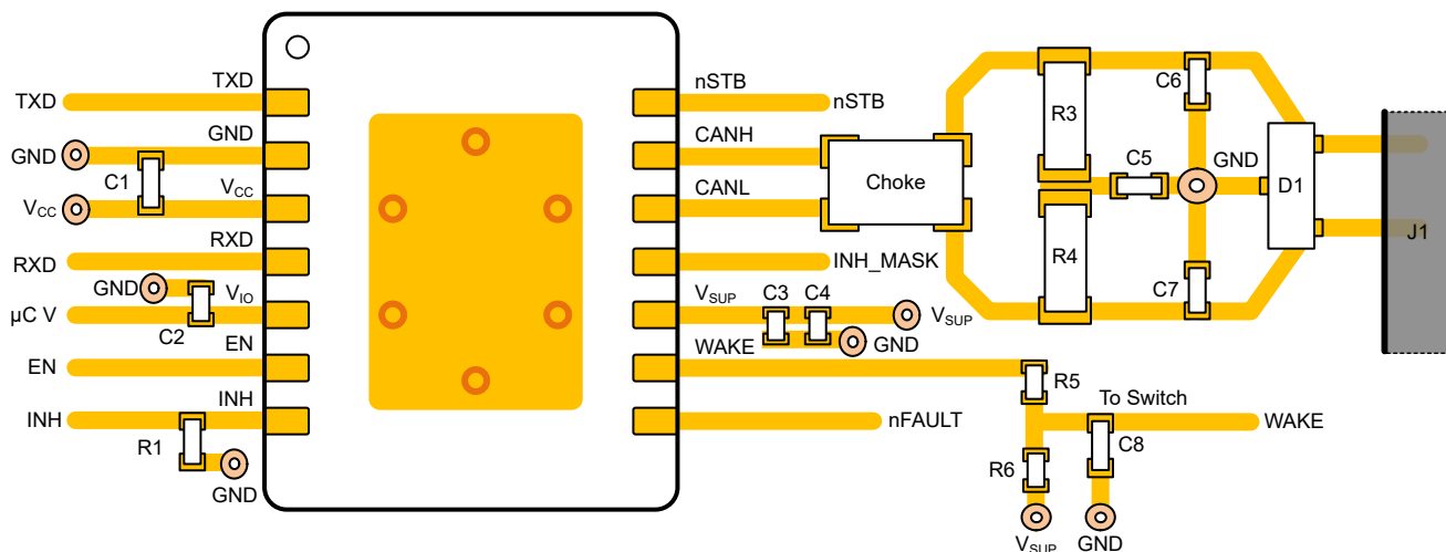
图 8-5. 示例布局
