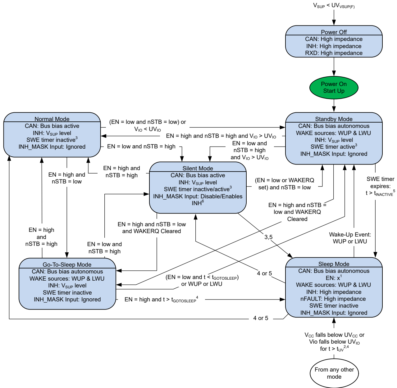
图 7-4. TCAN1473A-Q1 状态机
