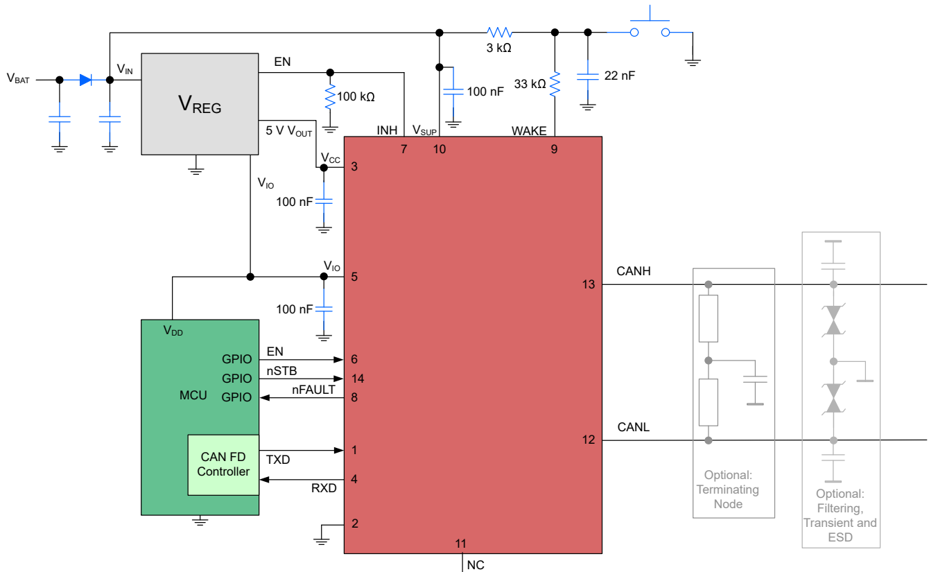
图 8-1. 典型应用
