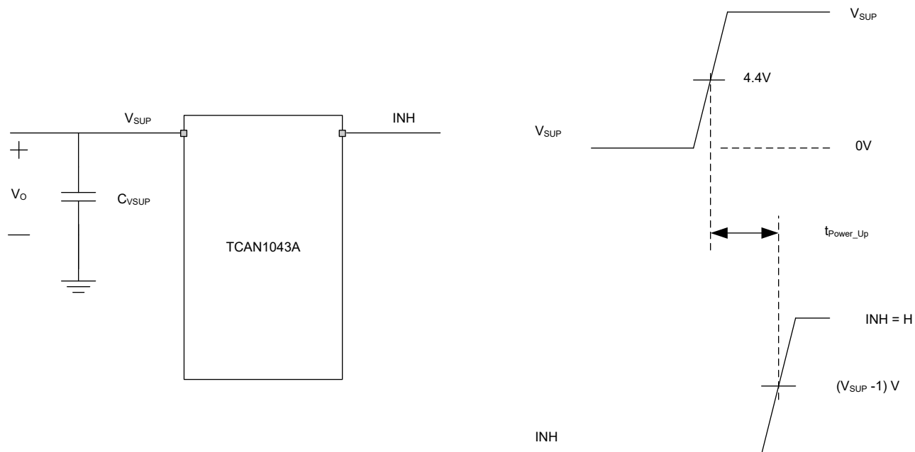
图 6-10. 上电时序
