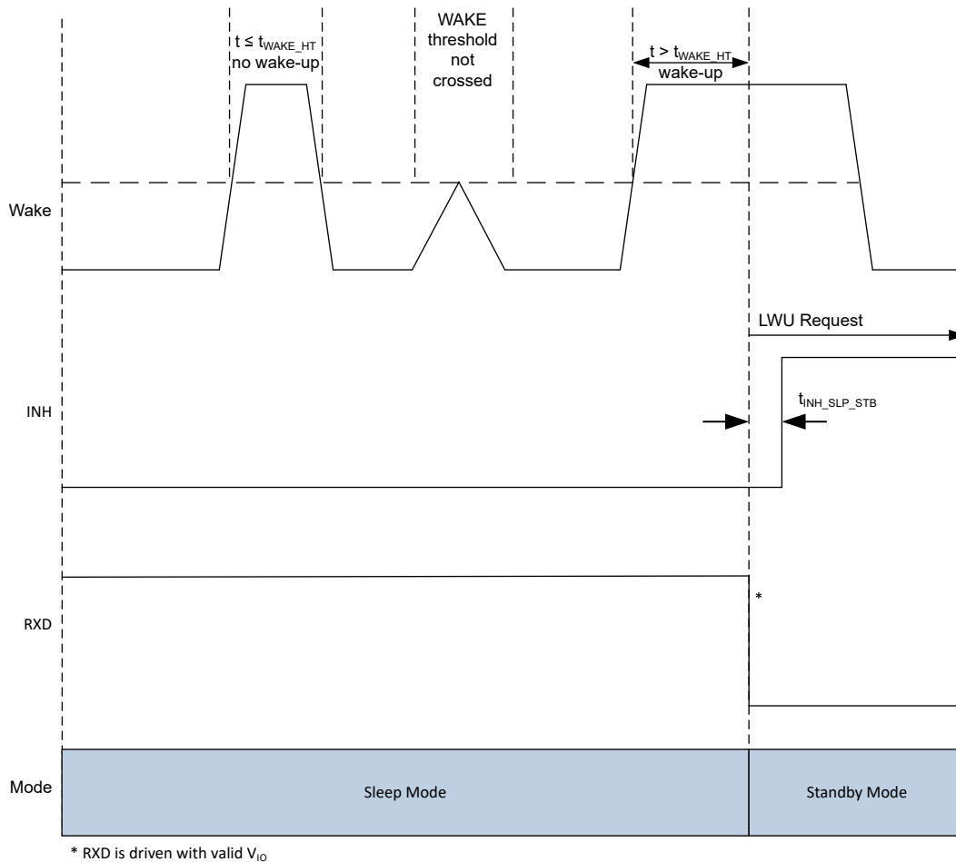
图 7-9. LWU 请求上升沿
