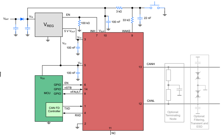
简化版应用原理图
