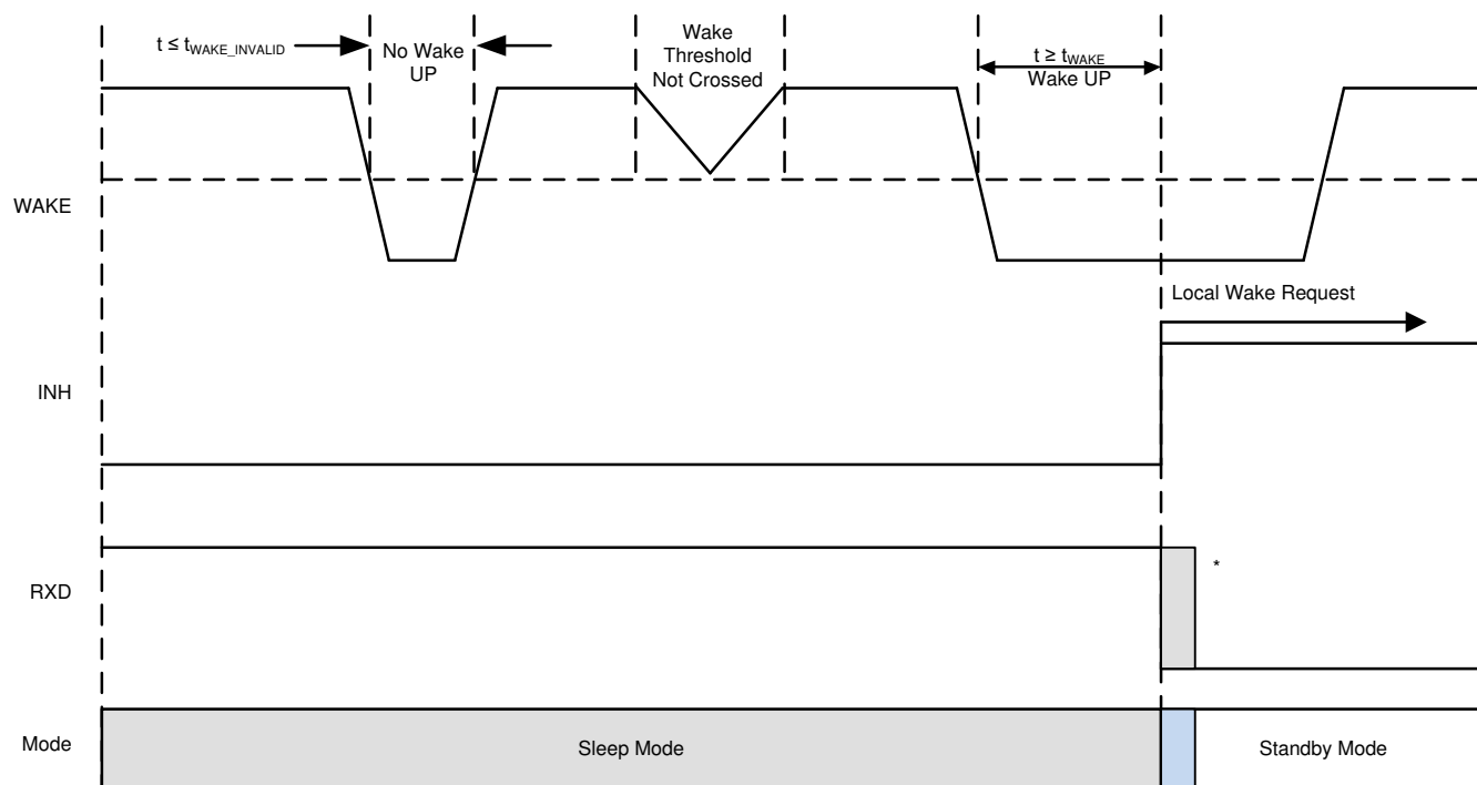
图 8-16. Local Wake Up - Falling Edge
