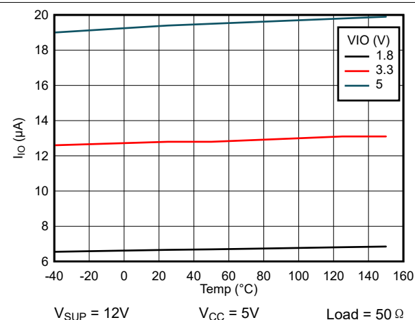
图 6-6. Normal Mode Dominant: I_{IO} vs Temperature
