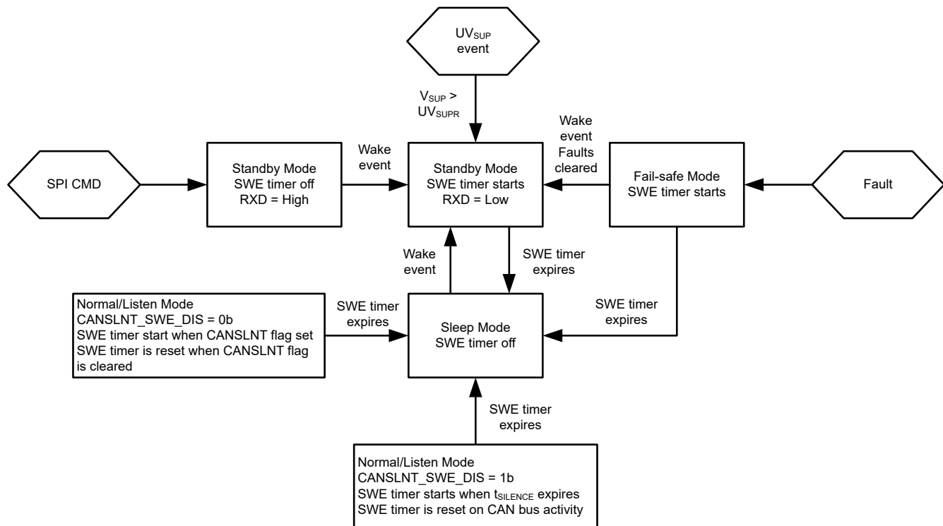
图 8-23. Sleep Wake Error (SWE) Timer if Enabled
