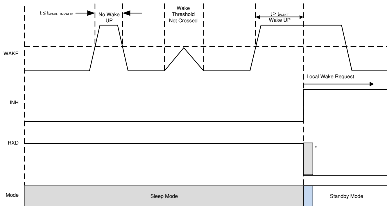
图 8-15. Local Wake Up - Rising Edge
