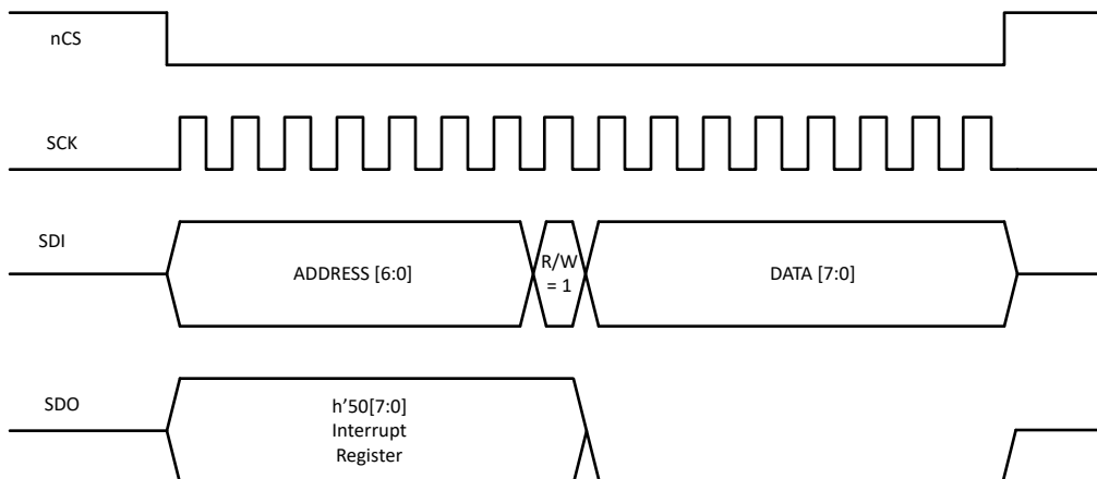
图 8-41. SPI Write
