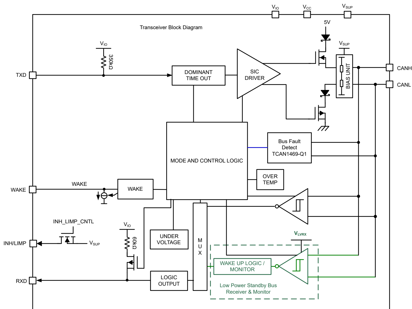
图 8-4. TCAN1469-Q1 CAN Transceiver Block Diagram
