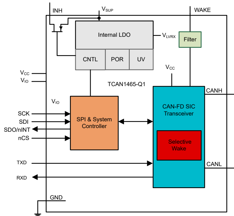
图 8-1. TCAN1465-Q1 Functional Block Diagram
