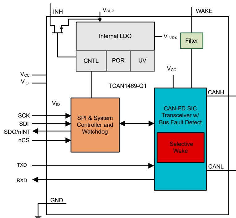
图 8-2. TCAN1469-Q1 Functional Block Diagram
