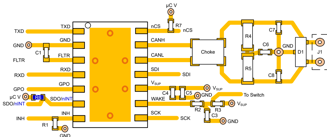
图 9-10. Example Layout
