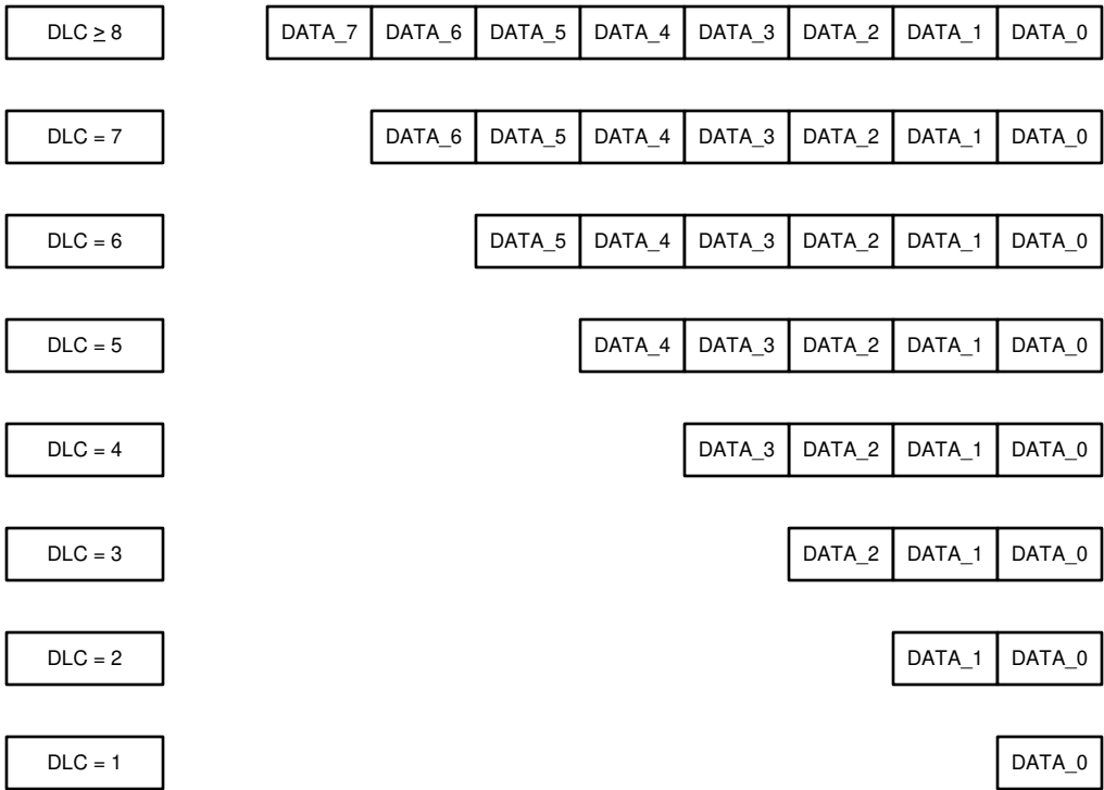
图 8-21. Data register mask values for different DLC values
