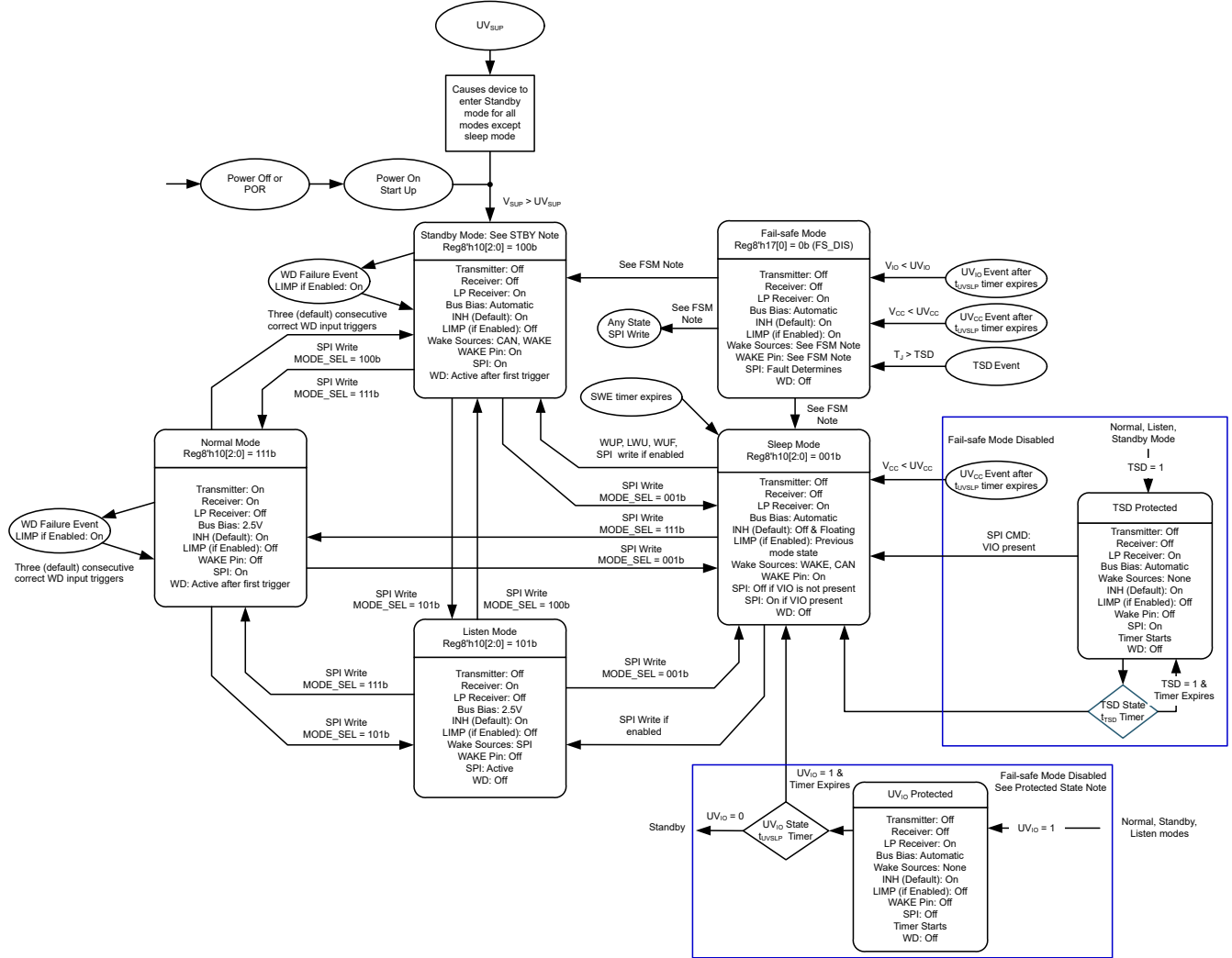
图 8-11. TCAN1469-Q1 Device State Diagram
