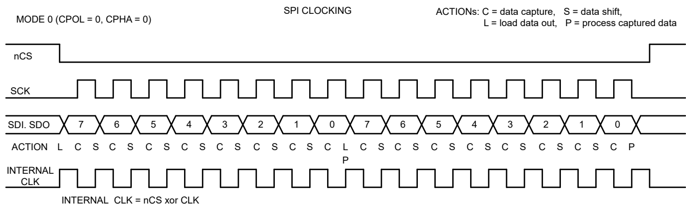
图 8-40. SPI Clcking
