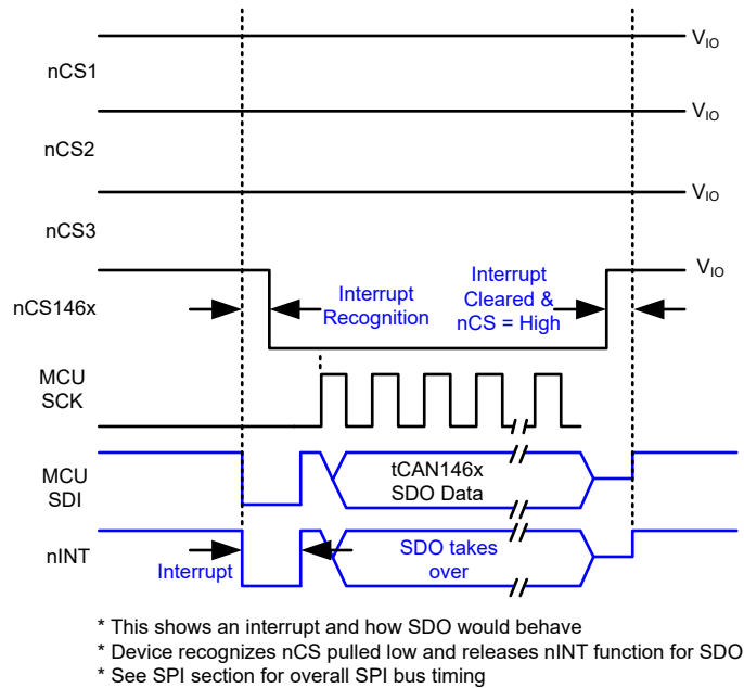
图 8-7. nINT Timing Diagram
