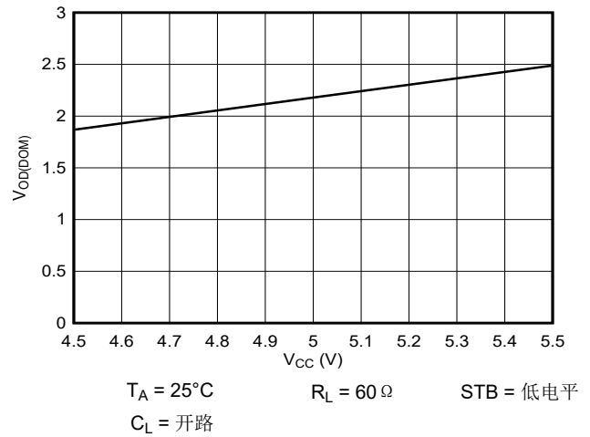
图 6-2. V_{OD(DOM)} 与 V_{CC} 间的关系
