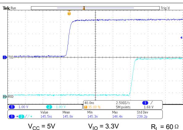
图 9-5. t_{\text{PROP(LOOP2)}}
