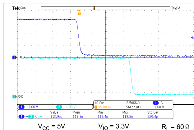
图 9-4. t_{\text{PROP(LOOP1)}}
