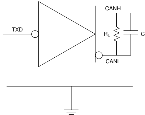
图 7-1. I_{CC} 测试电路
