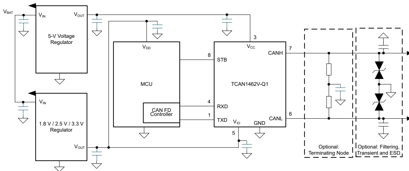
图 9-6. 使用 1.8V、2.5V、3.3V IO 连接的典型收发器应用
