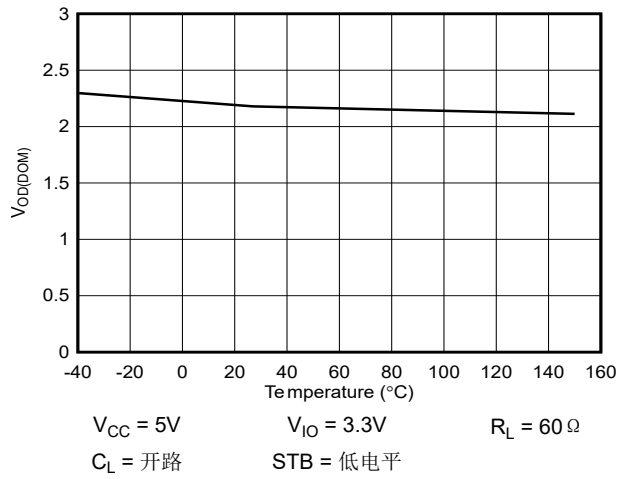
图 6-1. V_{OD(DOM)} 过热
