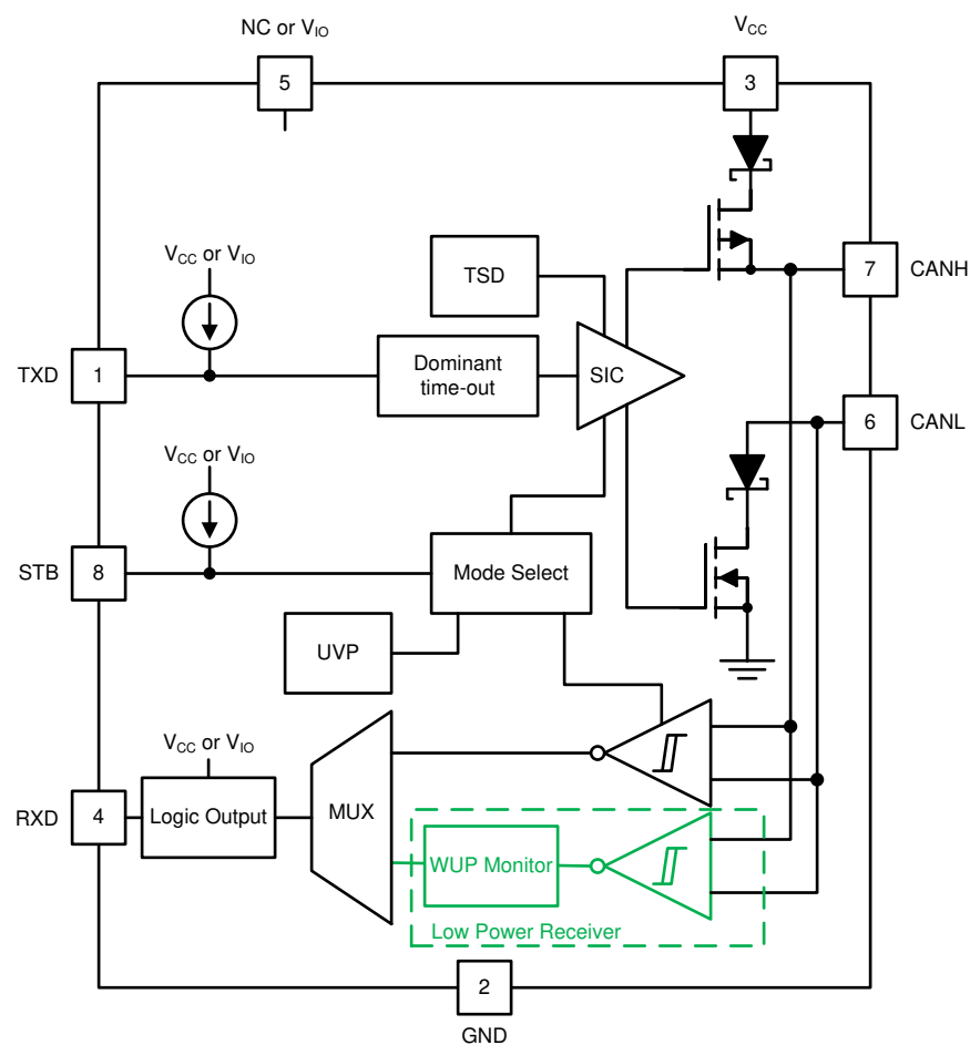
图 8-3. 方框图
