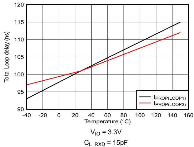
图 6-5. 总环路延迟 t_{PROP(LOOP1)} 和 t_{PROP(LOOP2)} 与温度间的关系
