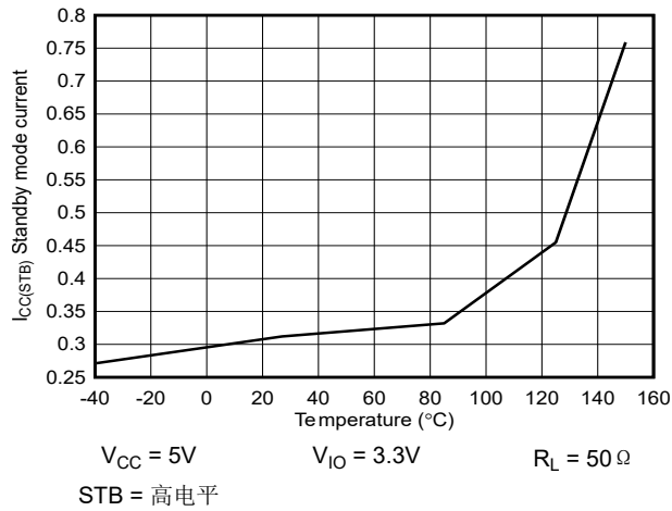
图 6-3. I_{CC(standby)} 与温度间的关系
