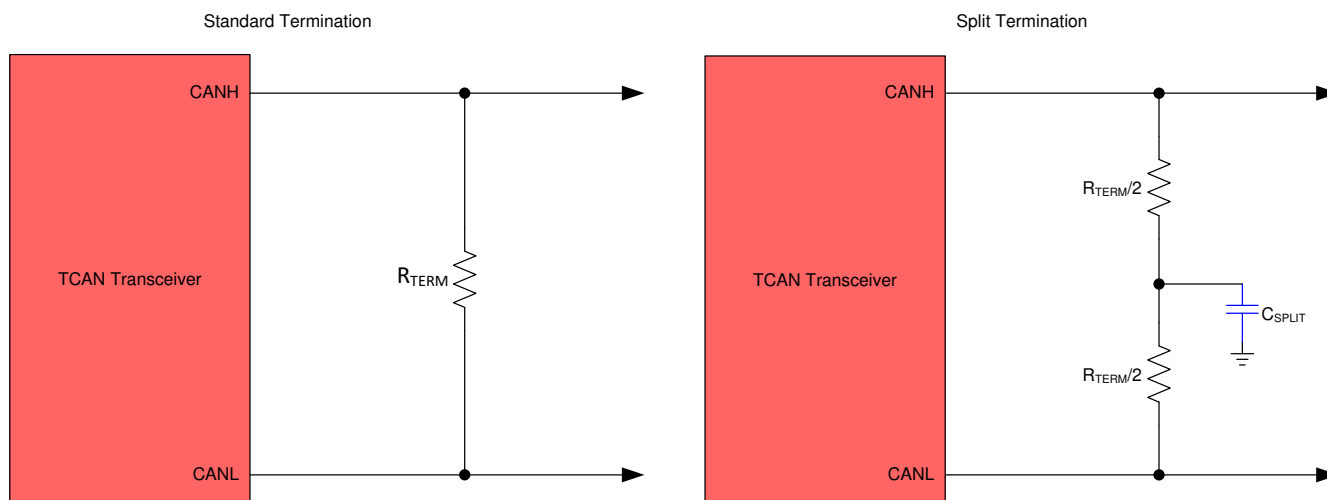
图 9-2. CAN 总线终端概念
