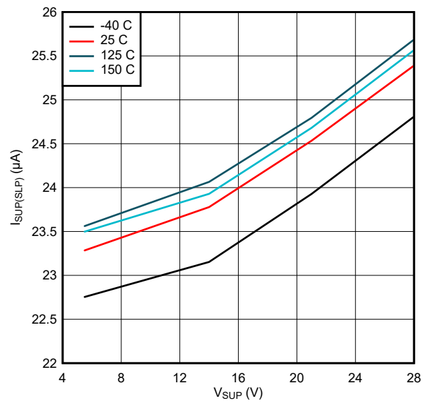
图 7-2. I_{SUP} over V_{SUP} Sleep Mode
