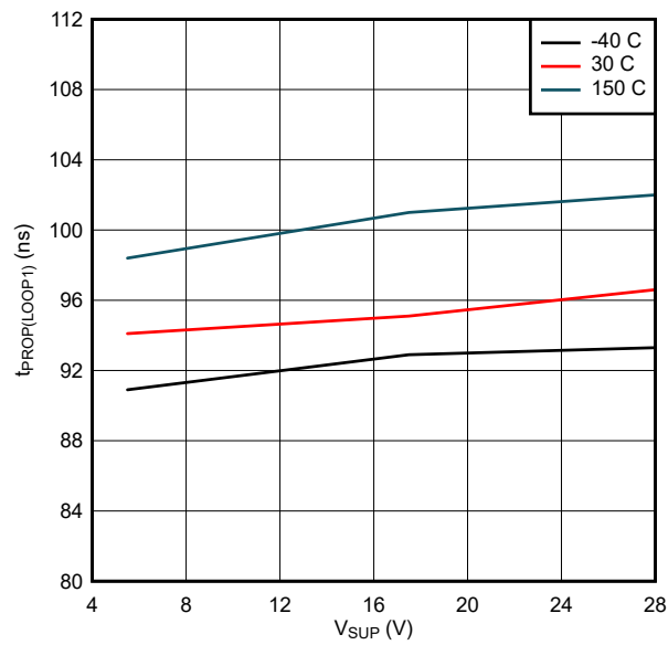
图 7-1. t_{PROP(LOOP1)} over V_{SUP}
