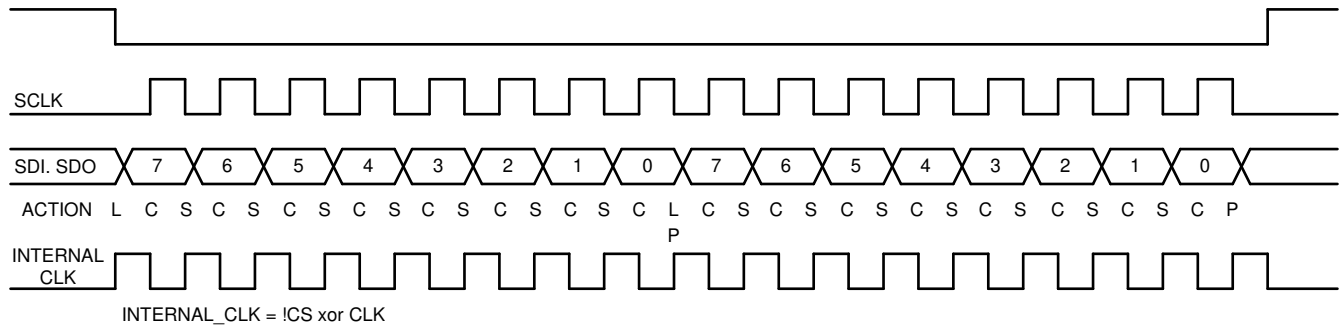
图 9-21. SPI Clocking
