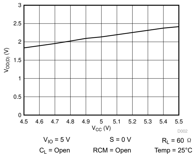
图 6-2. V_{OD(D)} over V_{CC}
