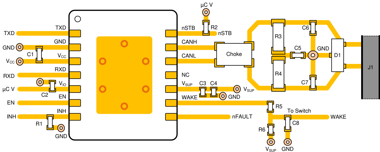
图 8-4. 示例布局
