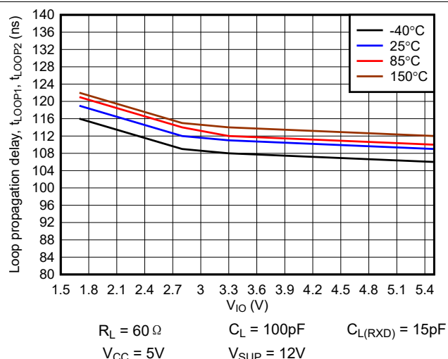
图 5-4. 环路传播延迟与 V_{IO} 和温度间的关系
