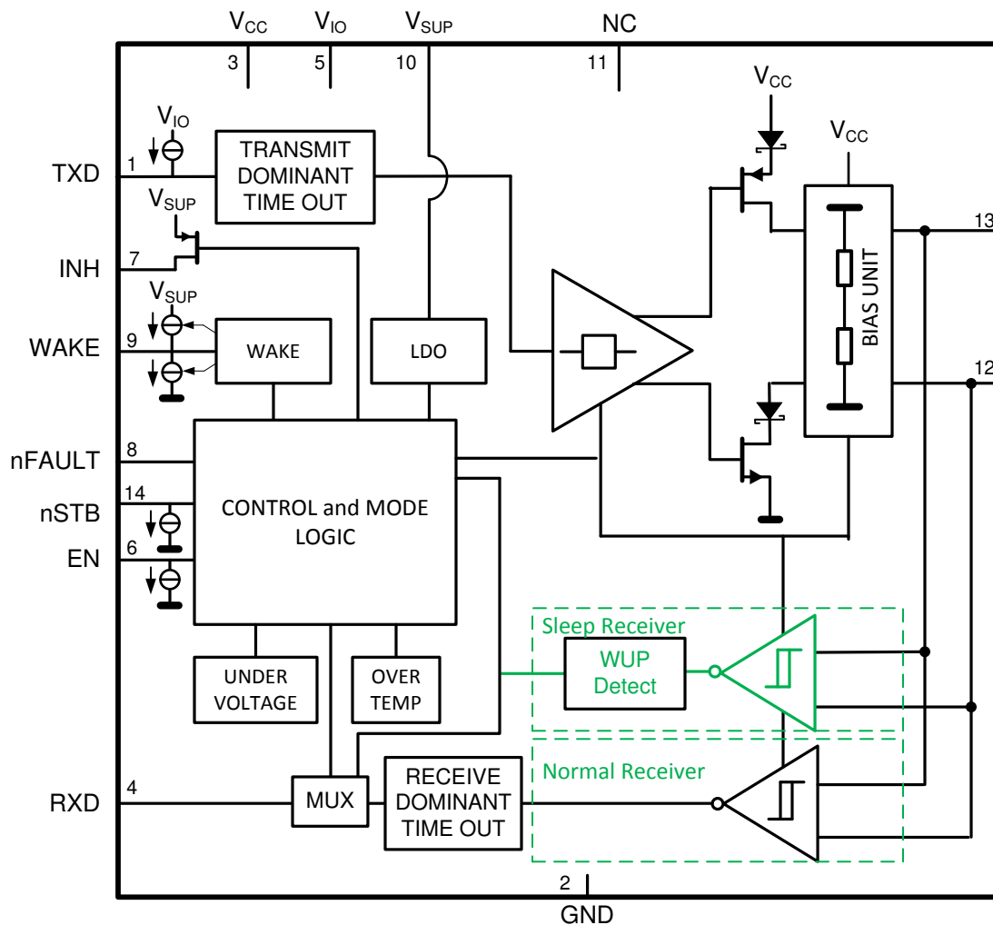
功能方框图
