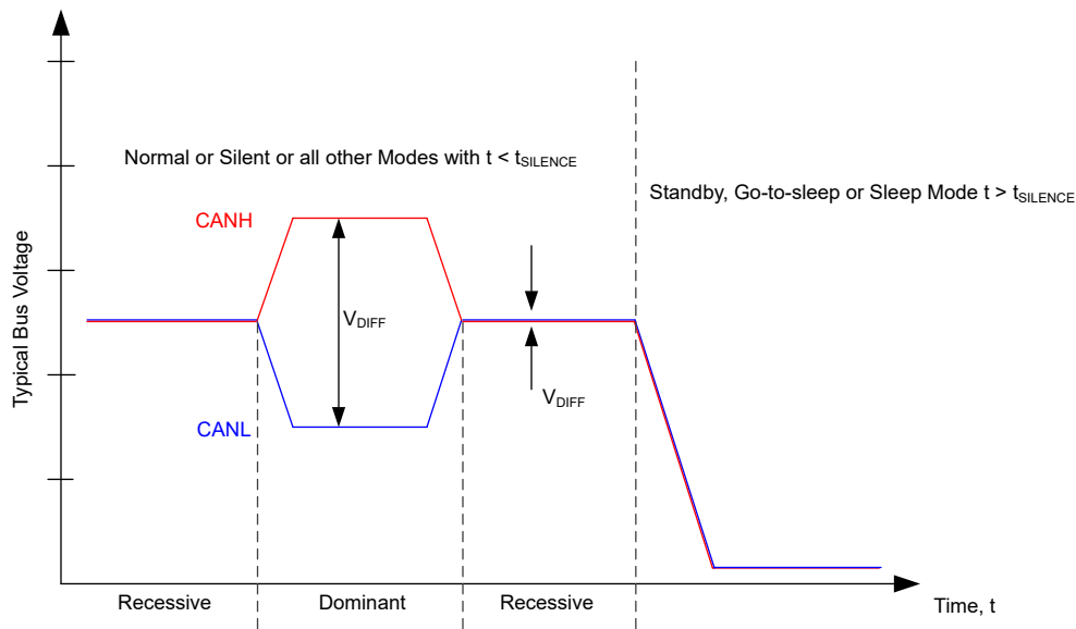
图 8-11. Bus States
