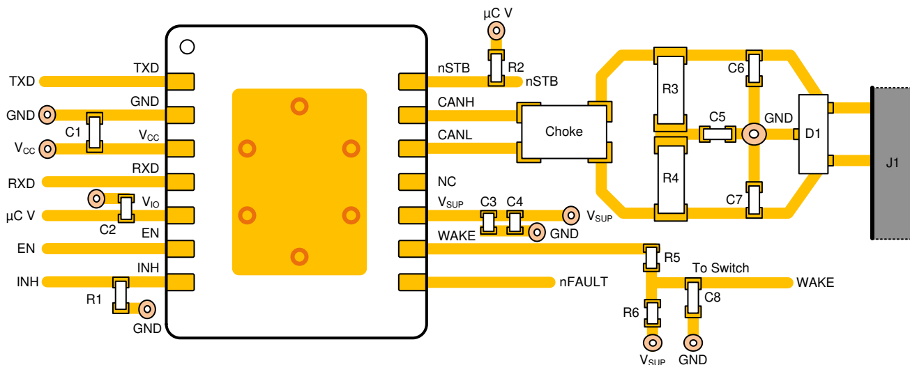
图 11-1. Example Layout
