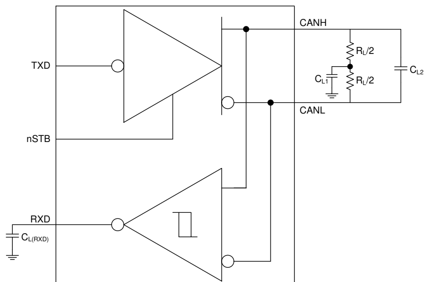
图 7-2. Test Circuit
