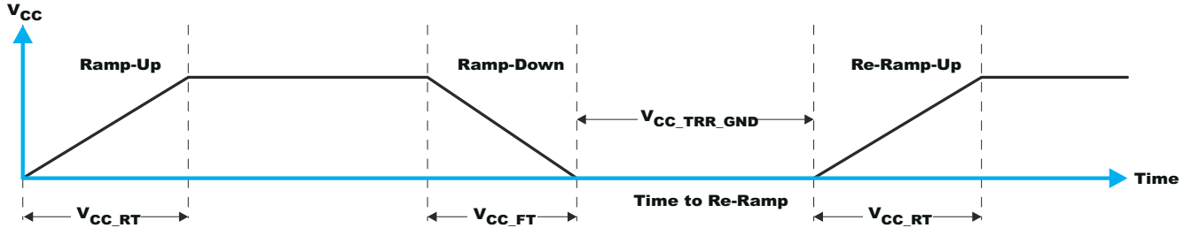
图 8-6. 将 V 降至 0.2V 或 0V 以下，然后上升
