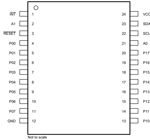
图 4-1. PW (TSSOP) 封装，24 引脚（俯视图）
