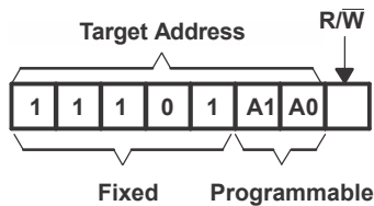
图 7-7. TCAL9539R 地址
