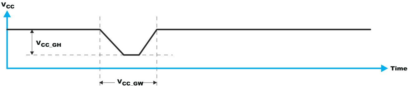
图 8-8. 干扰宽度和干扰高度
