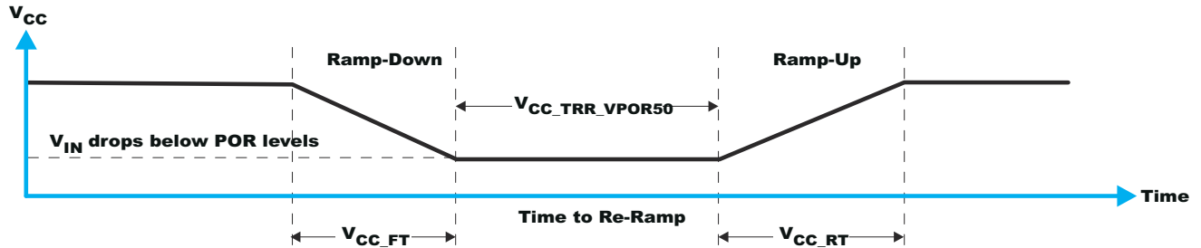
图 8-7. 将 V 降至低于 POR 阈值，然后重新上升
