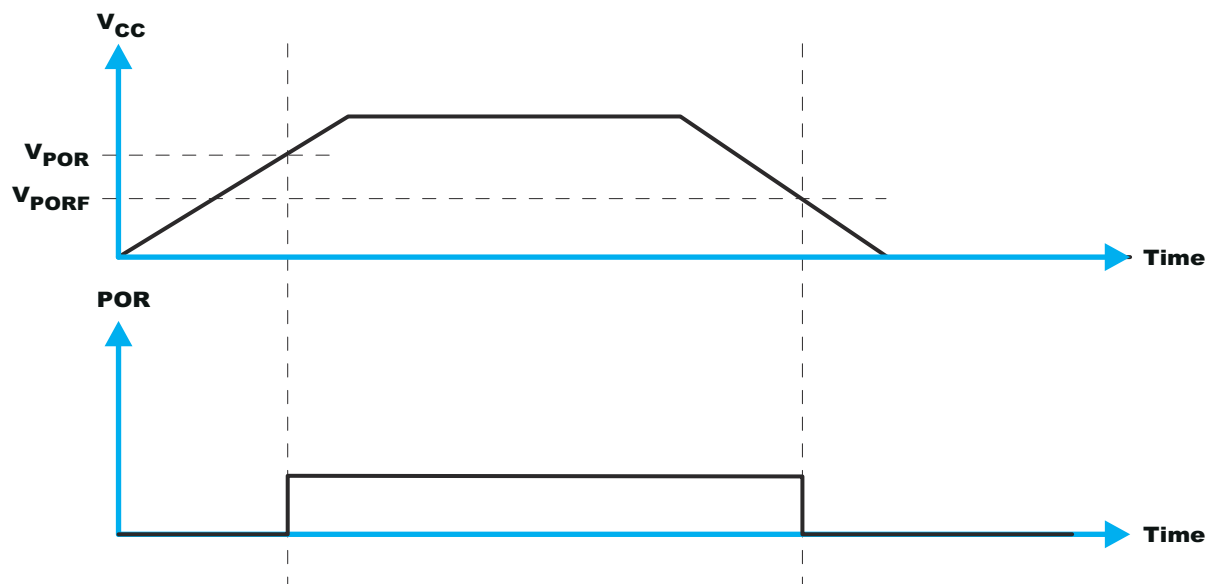
图 8-9. V_{POR}
