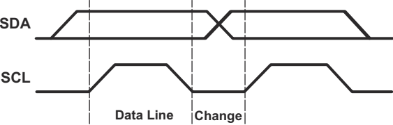
图 7-5. 位传输
