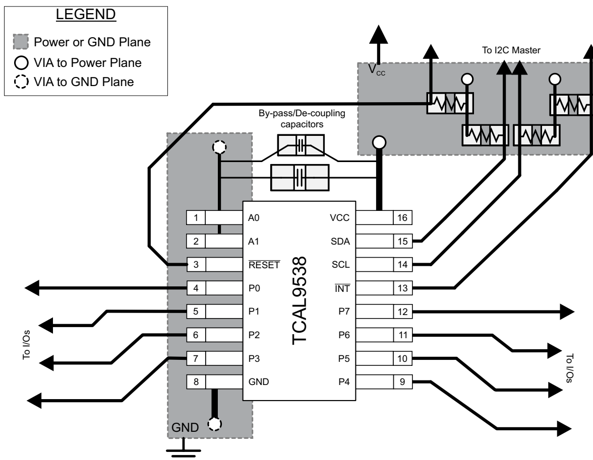
图 8-9. TCAL9538 布局
