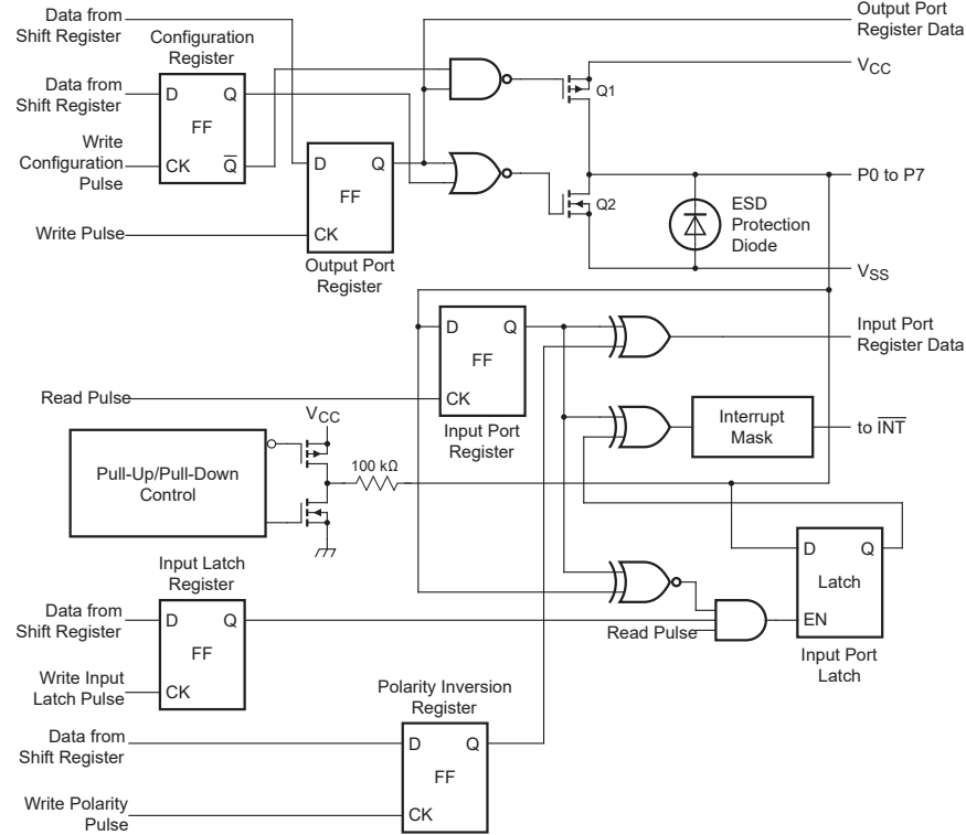
图 7-2. P0 至 P7 的简化原理图
