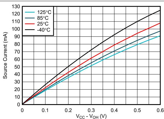
图 5-15. I/O 拉电流与输出高电压的关系， V_{CC} = 1.8\text{V}
