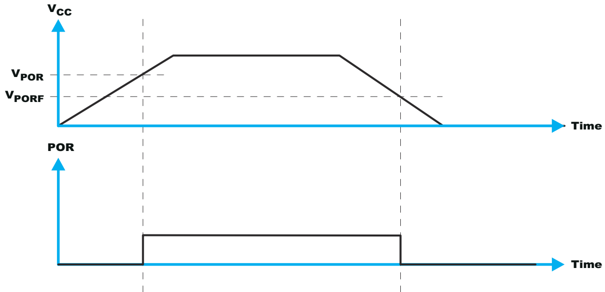
图 8-8. V_{POR}
