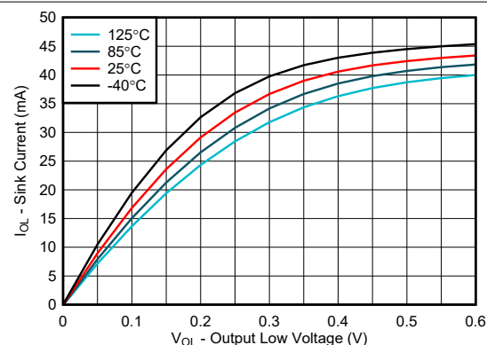
图 5-6. I/O 灌电流与输出低电压的关系, V_{CC} = 1.08V
