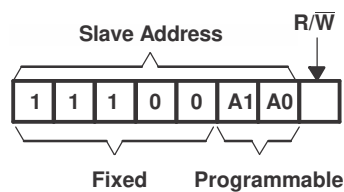
图 7-7. TCAL9538 地址
