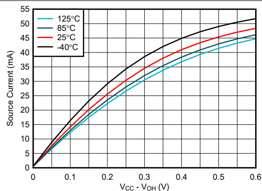
图 5-14. I/O 拉电流与输出高电压的关系， V_{CC} = 1.2\text{V}
