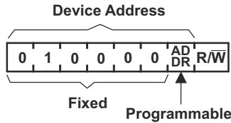
图 7-7. TCAL6416R 地址
