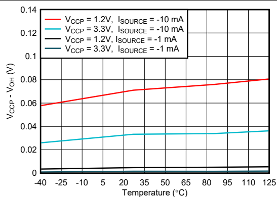
图 5-19. I/O 高电压与温度间的关系
