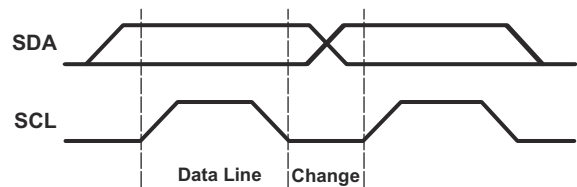
图 7-5. 位传输
