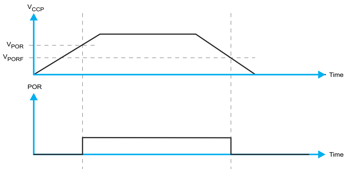
图 8-8. V_{POR}
