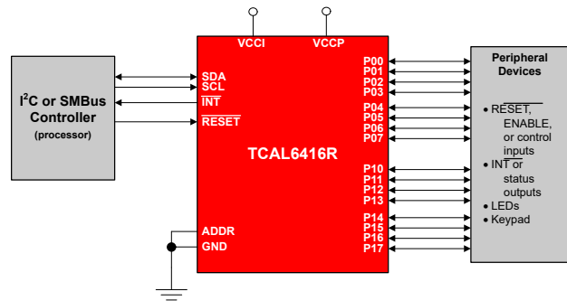
简化原理图
