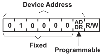
图 7-7. TCAL6416 地址
