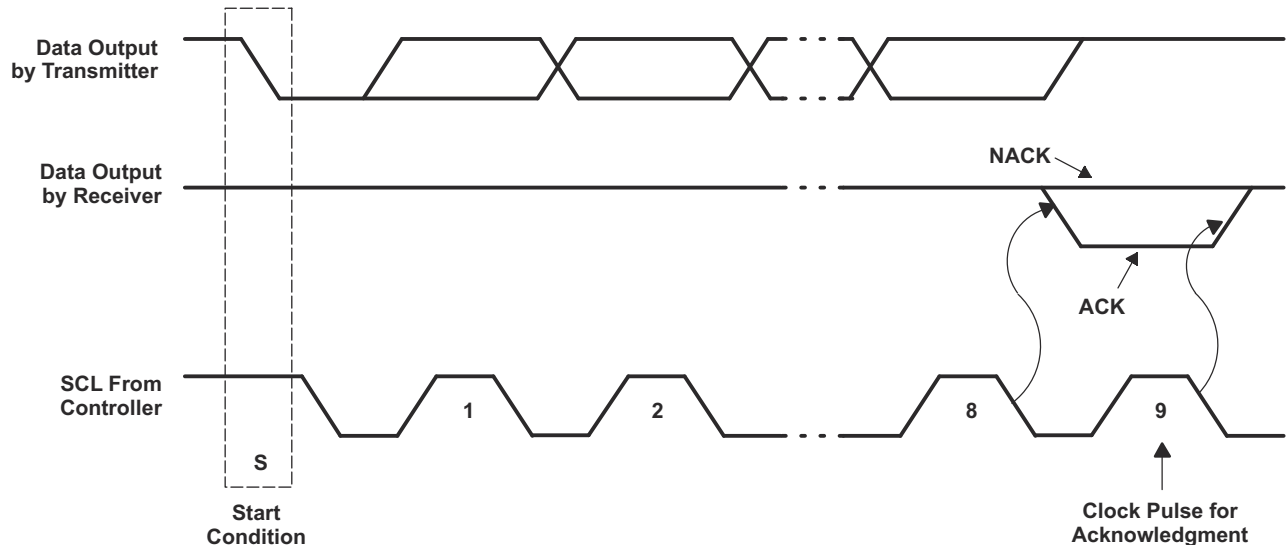
图 7-6. I²C 总线上的应答
