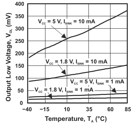
图 6-8. I/O Low Voltage vs Temperature
