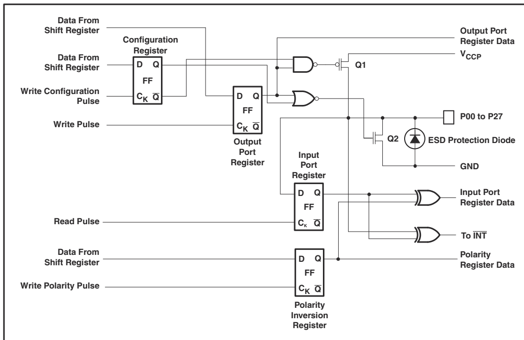
图 8-1. Positive Logic
