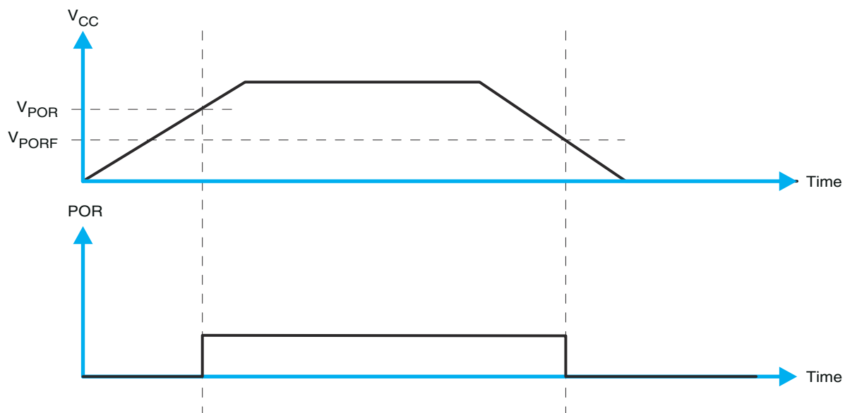
图 9-7. V_{POR}
