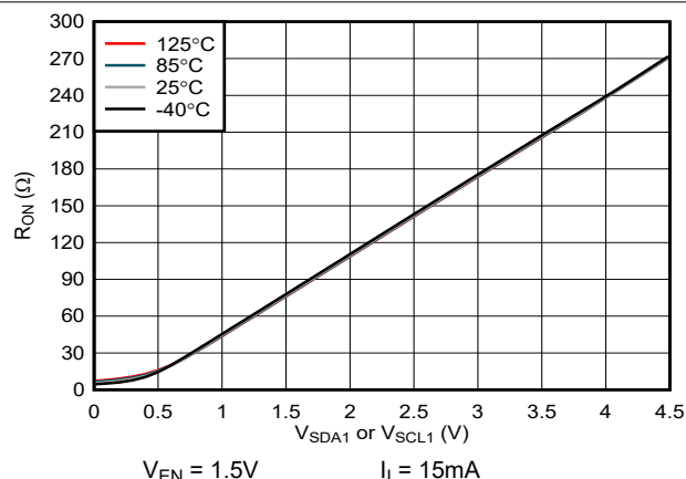
图 5-1. 导通电阻 ( R_{ON} ) 与输入电压间的关系 ( V_{SDA1} 或 V_{SCL1} )
