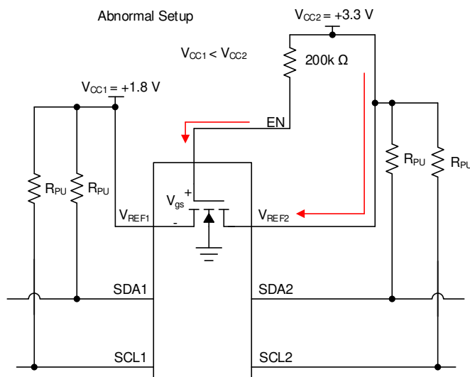
图 7-2. 异常设置
