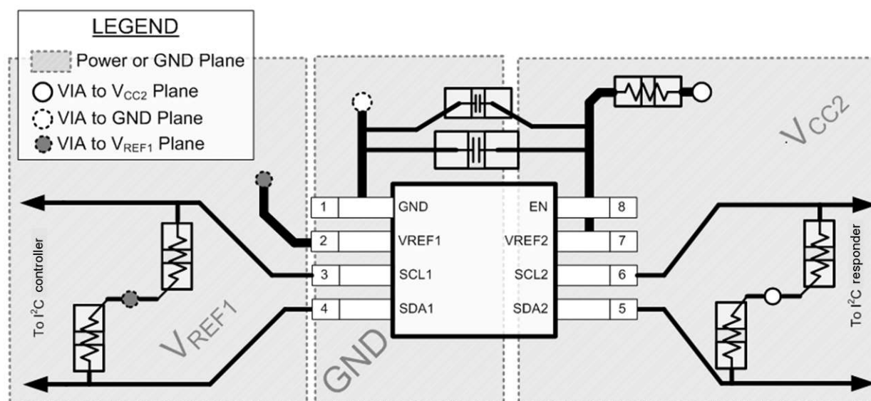
图 8-8. 布局示例
