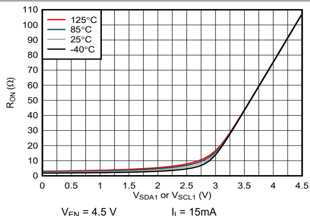
图 5-2. 导通电阻 ( R_{ON} ) 与输入电压间的关系 ( V_{SDA1} 或 V_{SCL1} )
