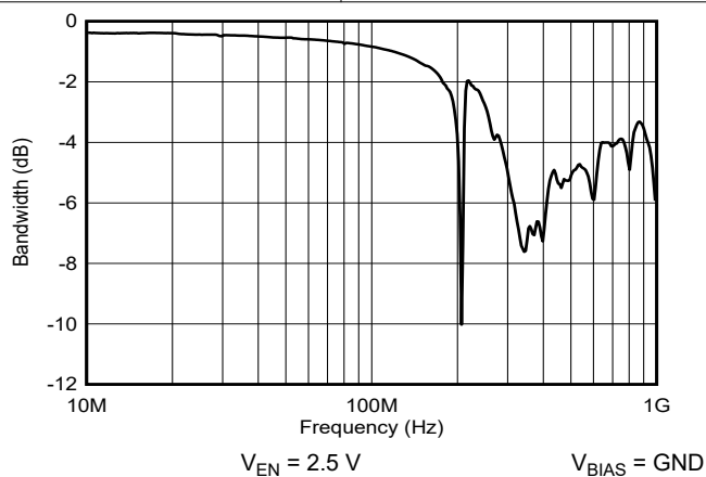
图 5-3. 典型带宽
