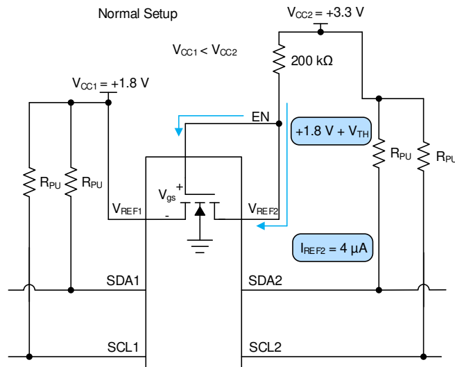
图 7-1. 正常设置
