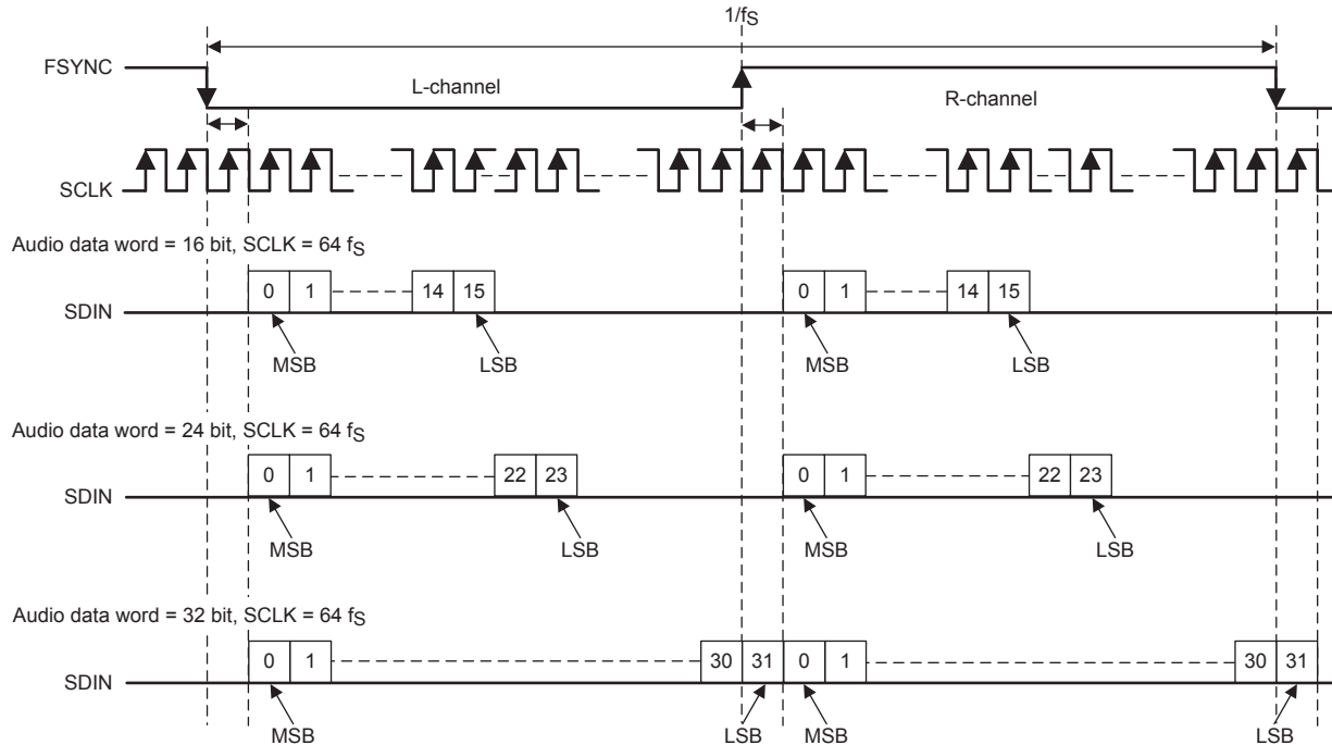
图 9-4. I²S Audio Data Format
