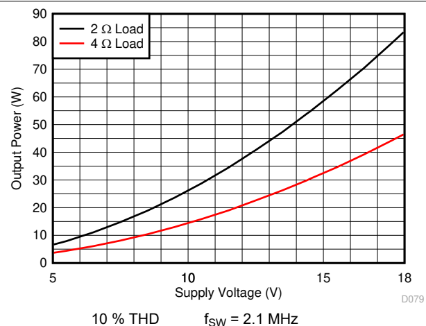
图 7-23. PBTL Output Power vs Voltage
