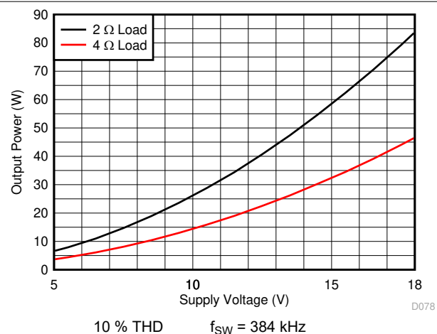
图 7-22. PBTL Output Power vs Voltage
