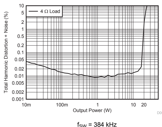
图 7-6. THD+N vs Power
