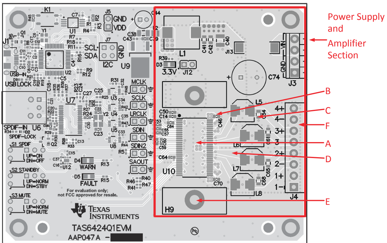
图 12-1. EVM Layout
