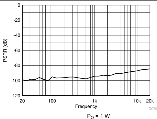
图 7-3. VBAT PSRR vs Frequency
