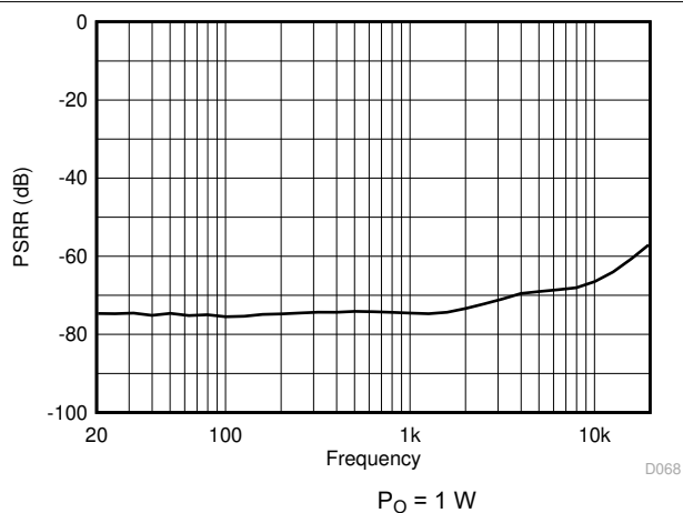
图 7-2. PVDD PSRR vs Frequency
