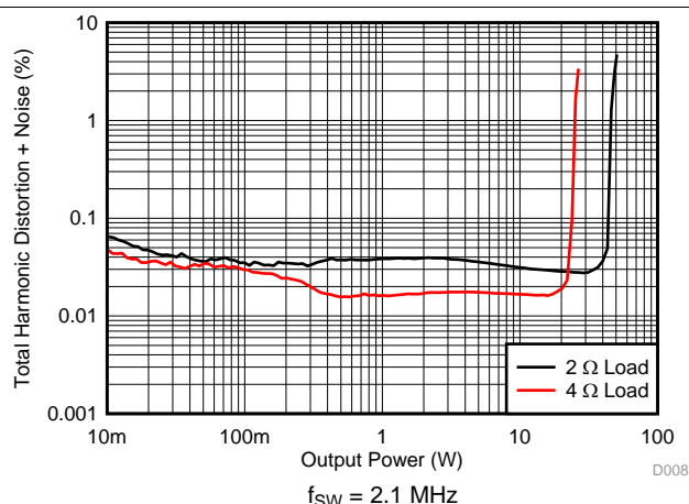
图 24. PBTL THD+N vs Power
