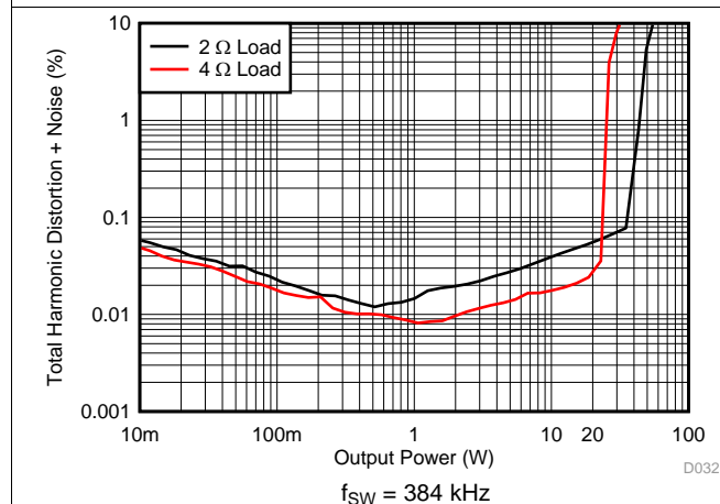
图 23. PBTL THD+N vs Power
