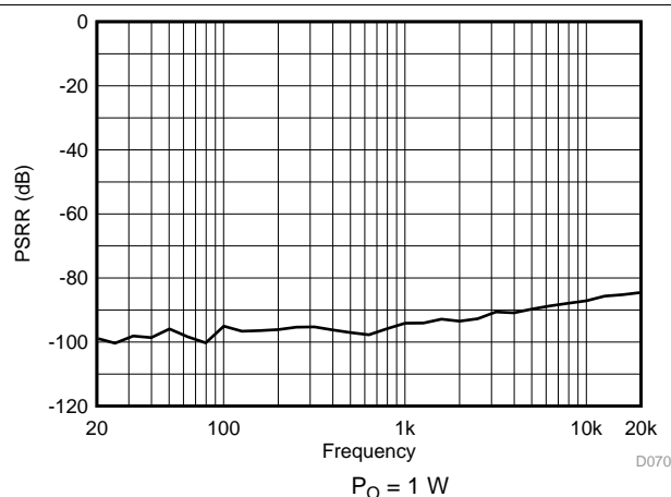
图 3. VBAT PSRR vs Frequency
