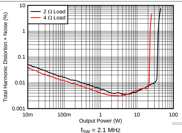
图 9. THD+N vs Power
