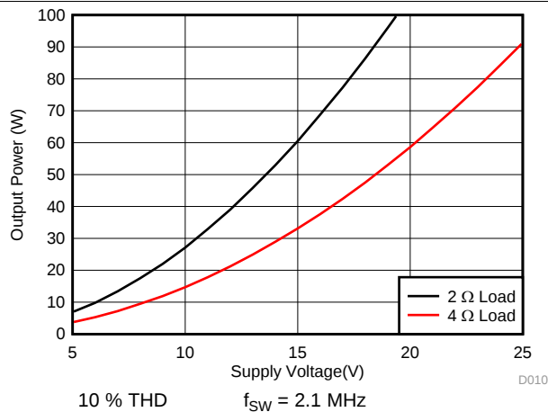
图 31. PBTl Output Power vs Voltage
