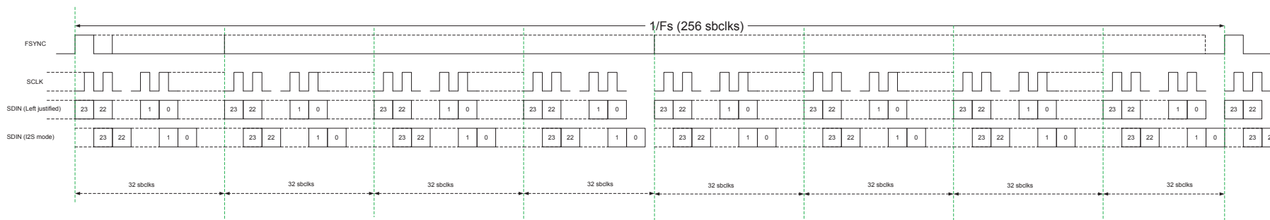
图 38. TDM8 Audio Data Format
