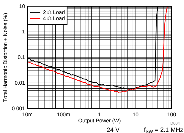
图 11. THD+N vs Power
