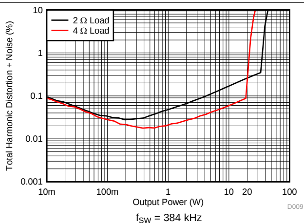
图 8. THD+N vs Power
