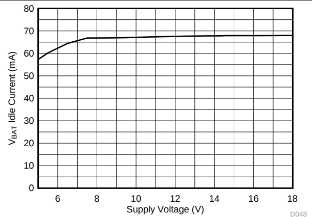
图 20. VBAT Idle Current vs Voltage
