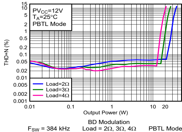
图 6-45. THD+N vs Output Power-PBTL
