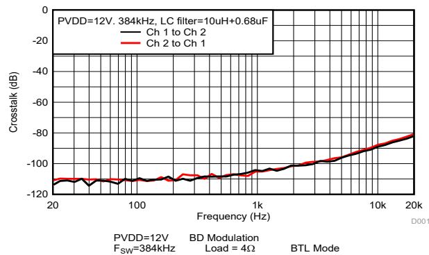
图 6-15. Crosstalk
