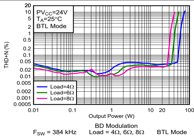
图 6-9. THD+N vs Output Power-BTL
