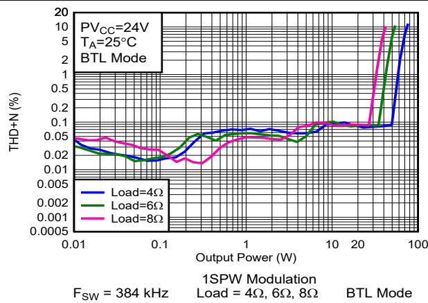
图 6-28. THD+N vs Output Power-BTL
