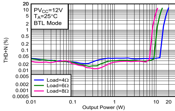
图 6-7. THD+N vs Output Power-BTL
