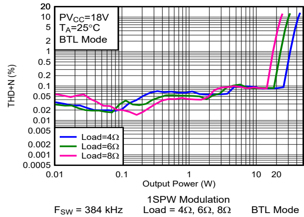
图 6-27. THD+N vs Output Power-BTL
