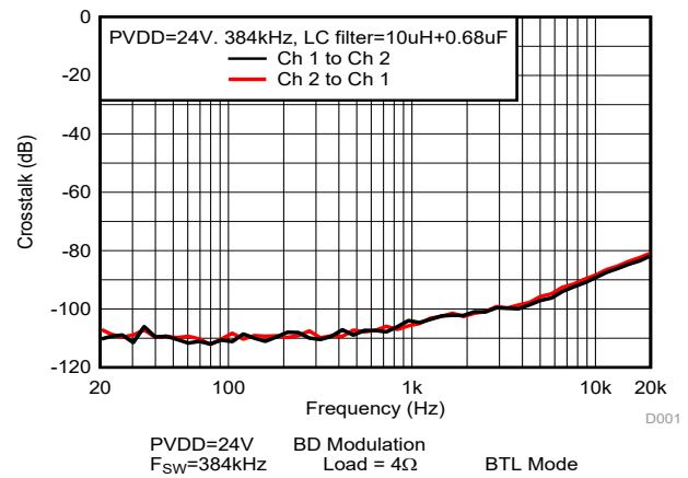
图 6-16. Crosstalk
