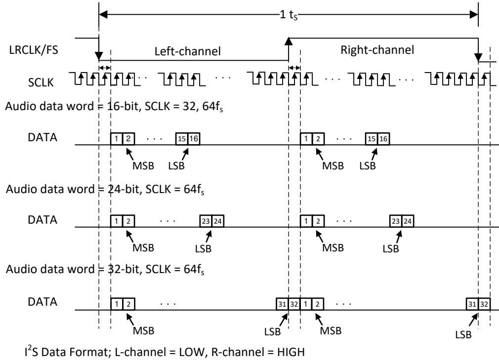
图 8-3. I²S Audio Data Format
