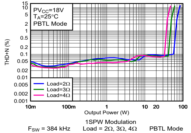
图 6-63. THD+N vs Output Power-PBTL
