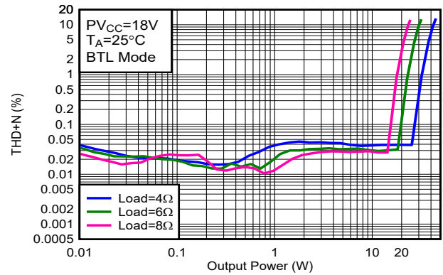
图 6-8. THD+N vs Output Power-BTL
