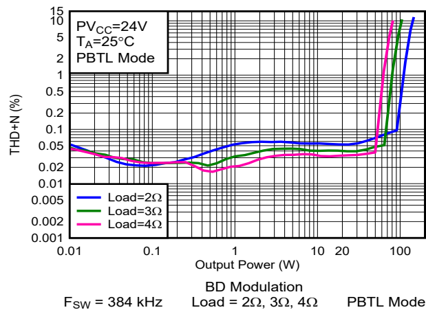
图 6-47. THD+N vs Output Power-PBTL
