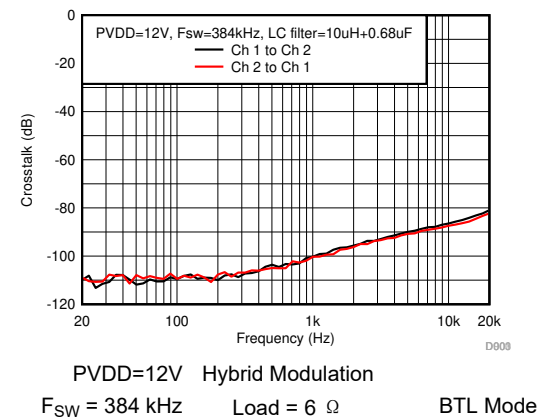
图 7-18. Crosstalk
