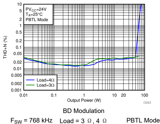
图 7-72. THD+N vs Output Power-PBTL
