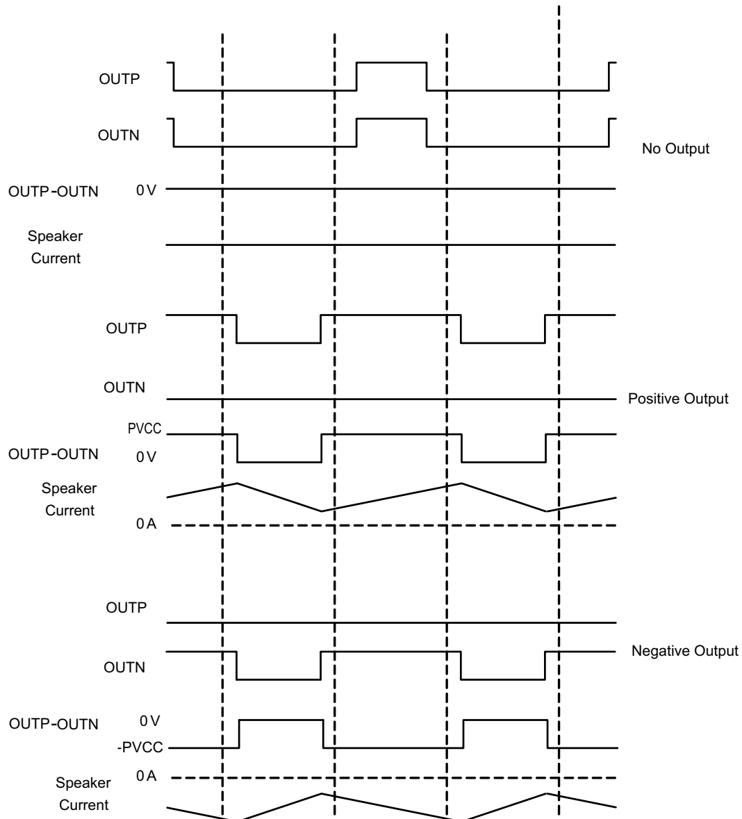
图 9-9. 1SPW Mode Modulation
