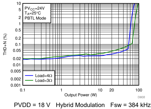
图 10-10. THD+N vs Output Power
