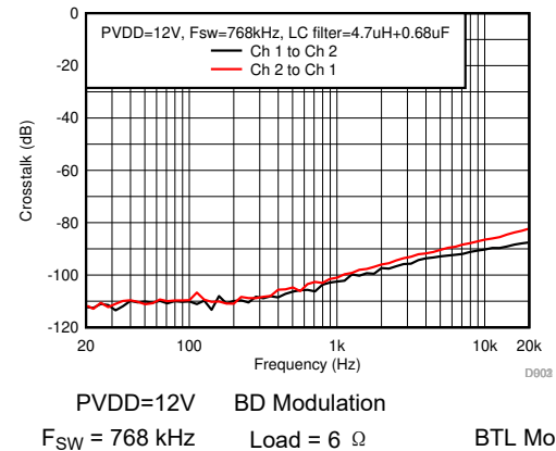
图 7-59. Crosstalk
