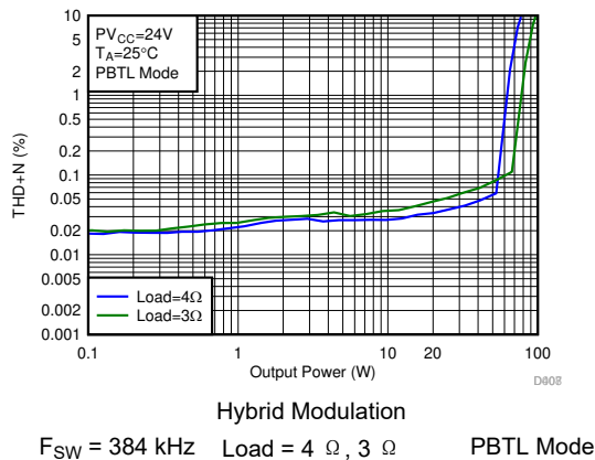
图 7-31. THD+N vs Output Power-PBTL
