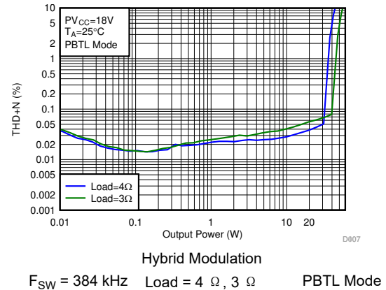
图 7-30. THD+N vs Output Power-PBTL
