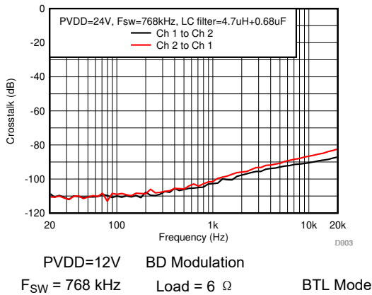
图 7-60. Crosstalk
