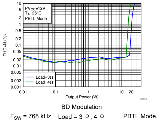
图 7-70. THD+N vs Output Power-PBTL
