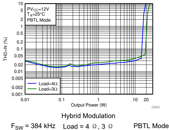
图 7-29. THD+N vs Output Power-PBTL
