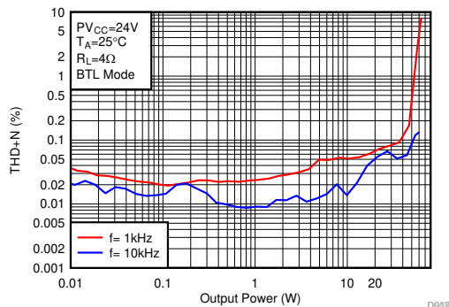
图 6-9. THD+N vs Output Power-BTL
