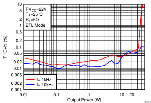
图 6-11. THD+N vs Output Power-BTL
