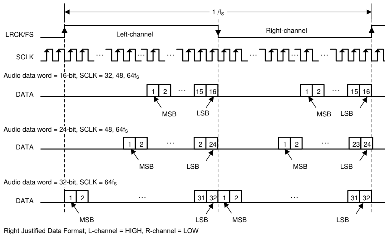
图 7-4. Right Justified Audio Data Format
