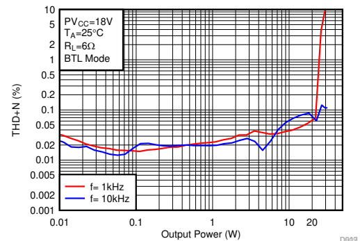
图 6-10. THD+N vs Output Power-BTL
