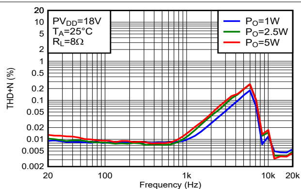
图 6-8. THD+N 与频率间的关系
