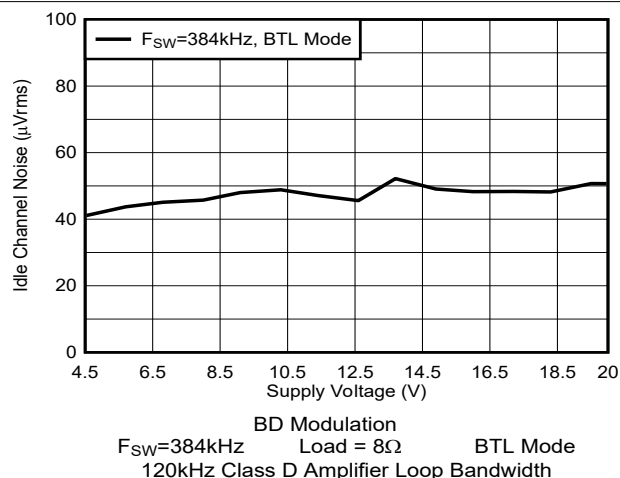
图 6-34. 空闲声道噪声与电源电压间的关系
