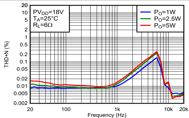
图 6-6. THD+N 与频率间的关系
