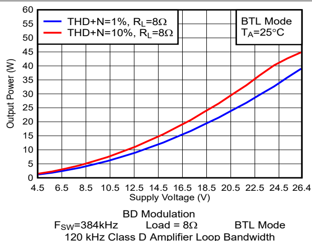
图 6-32. 输出功率与电源电压间的关系
