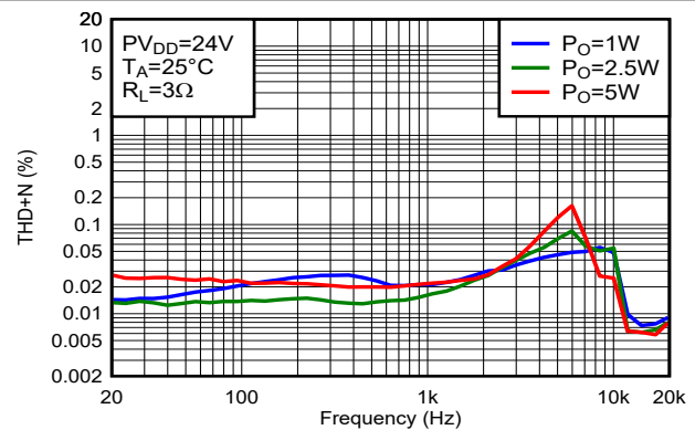
图 6-86. THD+N 与频率间的关系
