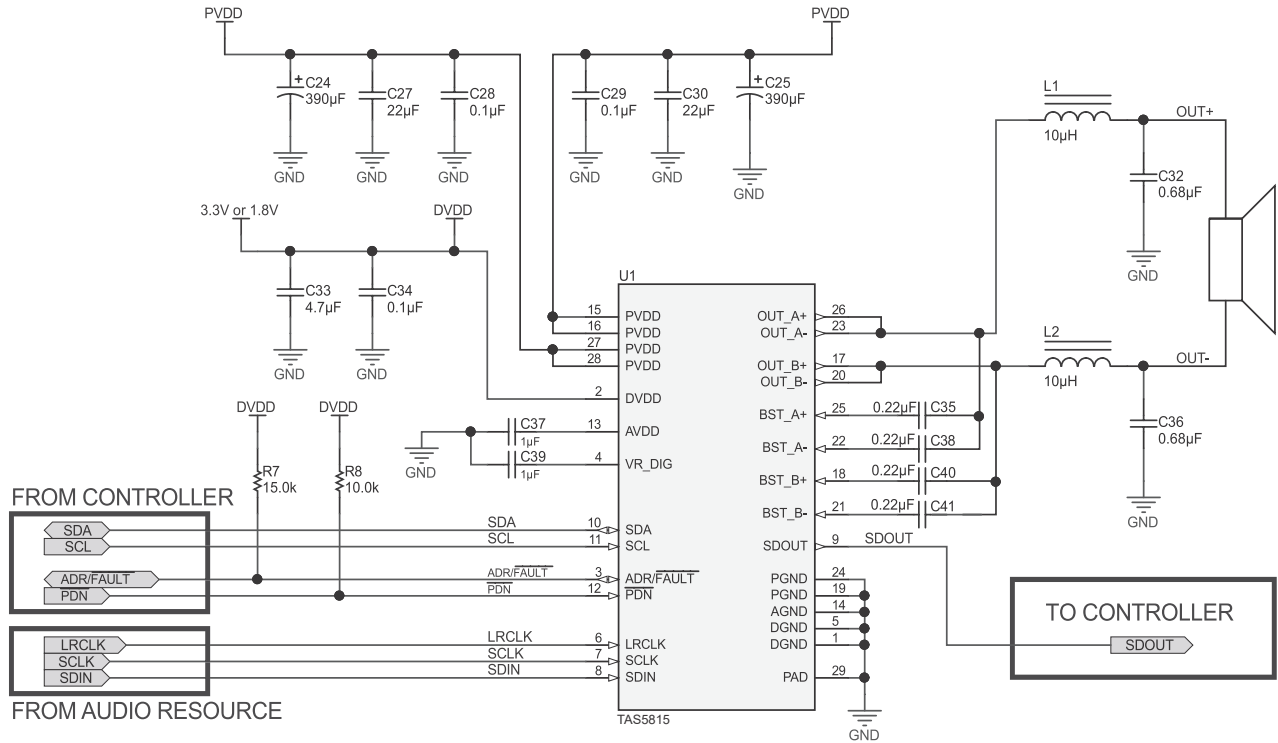
图 9-3. 单声道 (PBTL) 系统应用原理图
