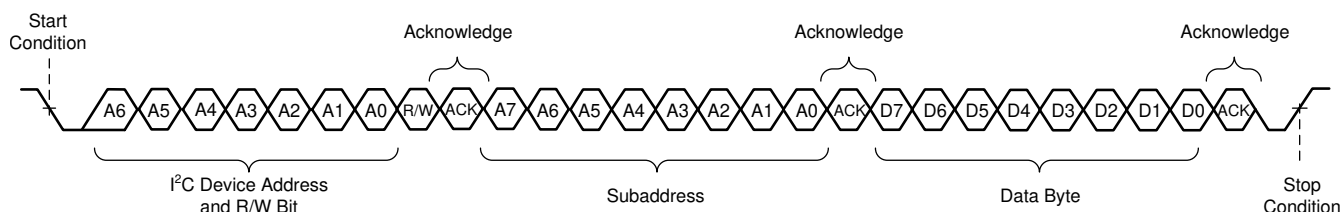
图 7-10. 随机写入传输
