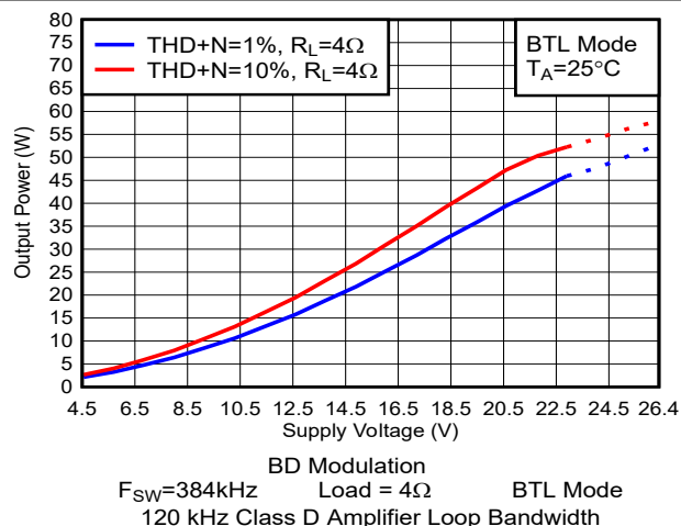
图 6-30. 输出功率与电源电压间的关系
