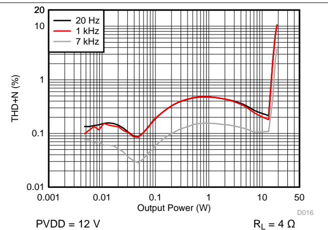
图 20. THD+N vs Output Power - PBTL
