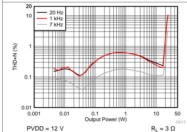
图 21. THD+N vs Output Power - PBTL
