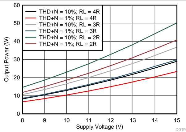
图 23. Output Power vs PVDD - PBTL
