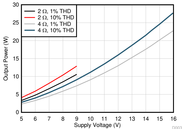
图 6-3. Output Power vs PVDD
