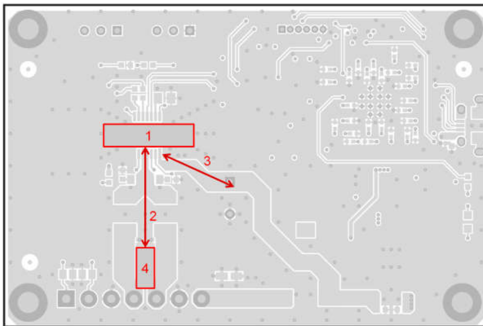
图 9-1. Top layer
