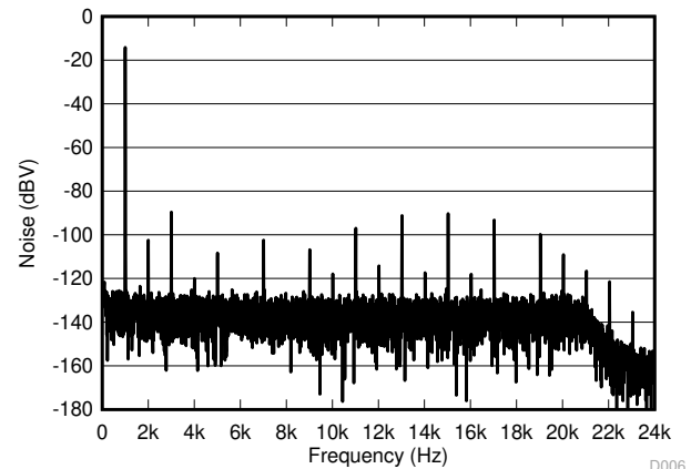
图 6-6. Noise FFT With 1-W Output
