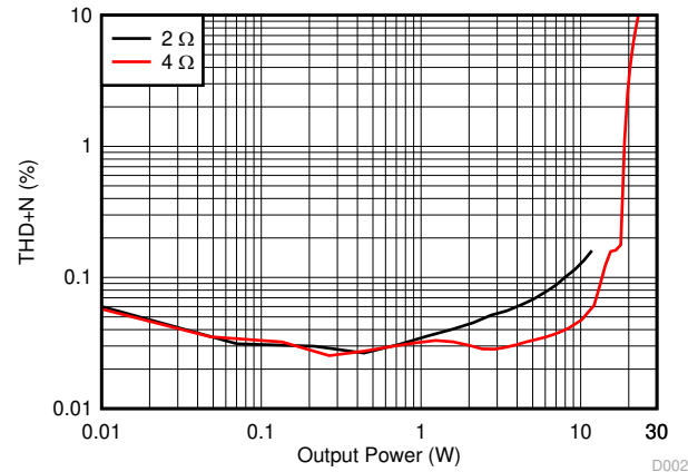
图 6-2. THD+N vs Output Power
