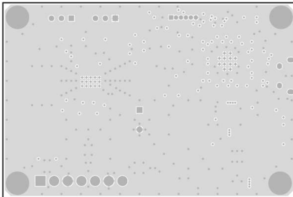
图 9-2. Signal Layer
