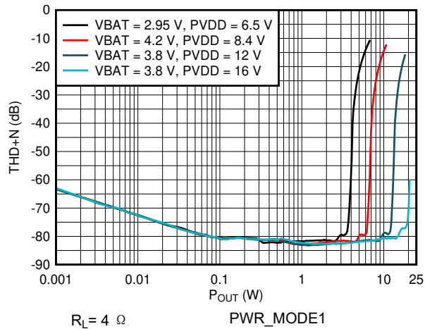
图 6-3. THD+N vs Output Power
