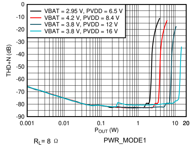
图 6-4. THD+N vs Output Power
