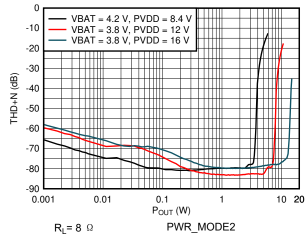
图 6-6. THD+N vs Output Power
