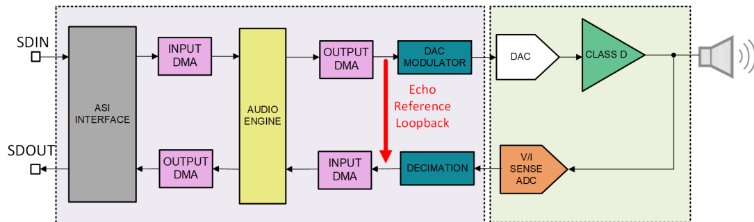
图 8-11. Echo Reference Loopback
