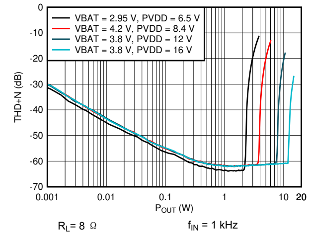
图 6-38. V Sense THDN vs Pout
