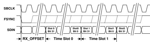
图 8-3. TDM RX Time Slots
