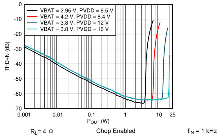
图 6-37. V Sense THDN vs Pout
