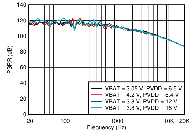
图 6-24. VBAT PSRR vs Frequency
