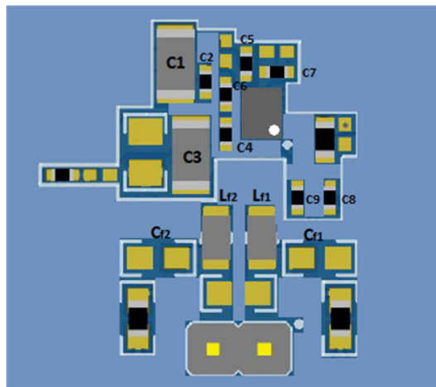
图 12-1. Component Placement
