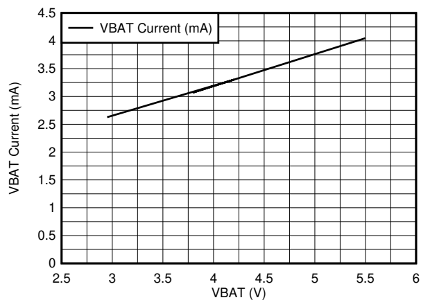
图 6-27. VBAT Idle Current vs VBAT
