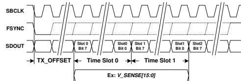
图 8-4. TDM Port TX Diagram
