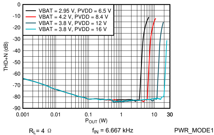
图 6-7. THDN vs Output Power
