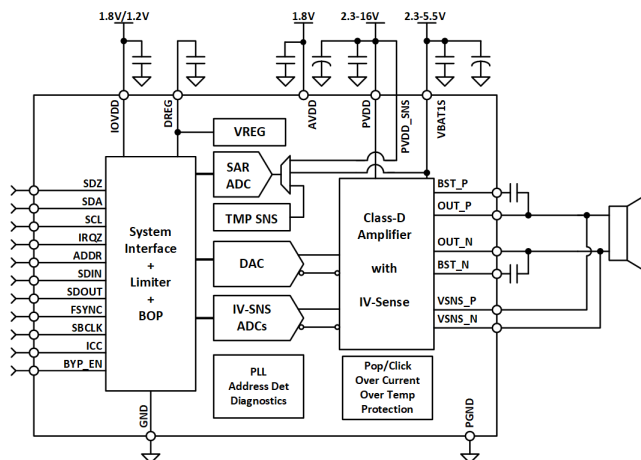
原理图
