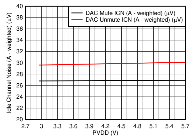
图 6-16. ICN (A-Weighted) vs PVDD
