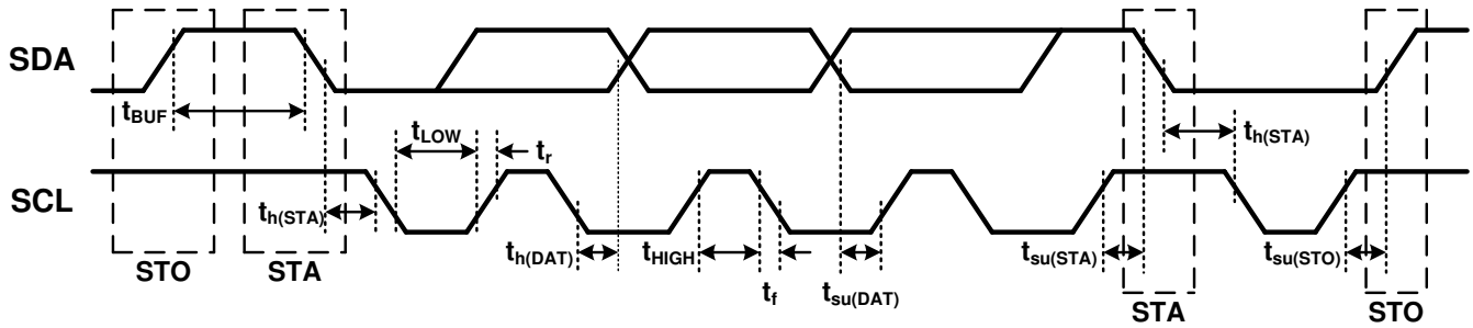
图 5-1. I²C Timing Diagram
