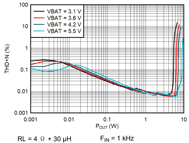
图 5-6. THD+N vs Output Power (QFN Package)
