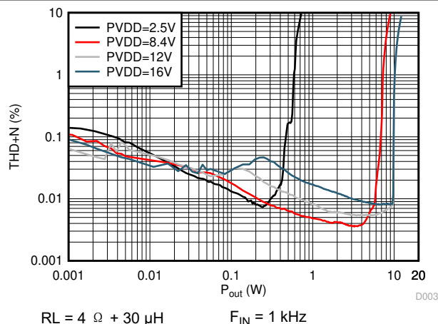
图 5-9. THD+N vs Output Power
