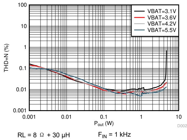
图 5-7. THD+N vs Output Power (DSBGA Package)
