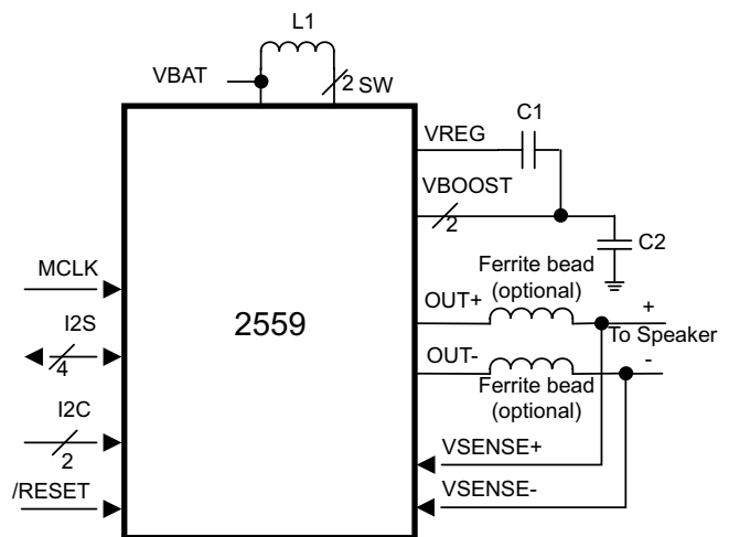
简化原理图
