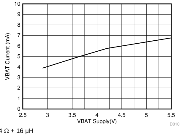
图 16. Quiescent Current vs VBAT
