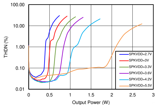
(增益 = 18dB) 图 9-3. 总谐波失真 + 噪声与 4 \Omega 扬声器功率间的关系
