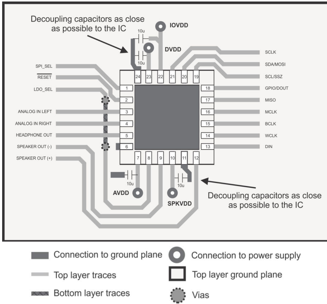
图 9-5. 布局图
