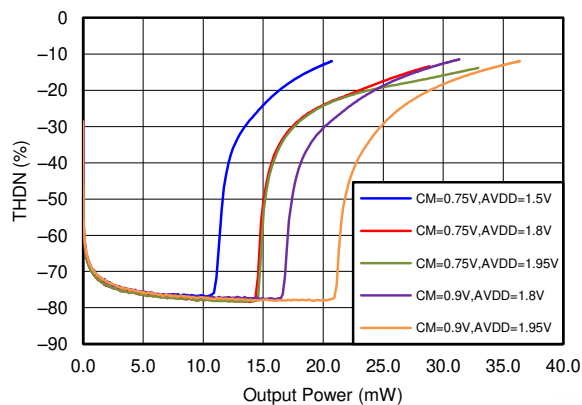
(增益 = 9dB) 图 9-4. 总谐波失真 + 噪声与 HP 功率间的关系
