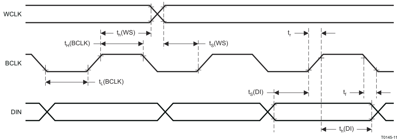
图 5-2. 从模式下的 I²S/LJF/RJF 时序
