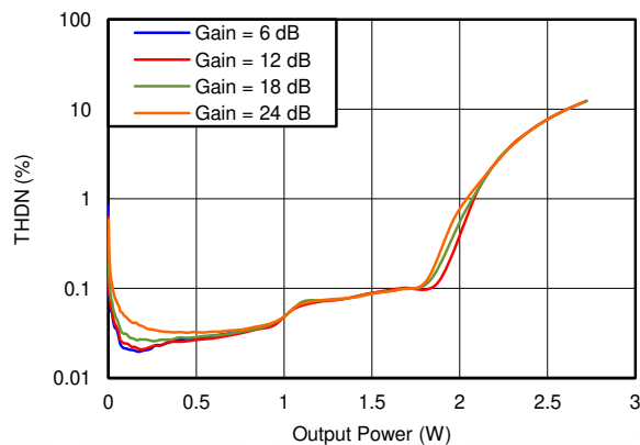
(SPKVDD = 5.5V) 图 9-2. 总谐波失真 + 噪声与 4 \Omega 扬声器功率间的关系
