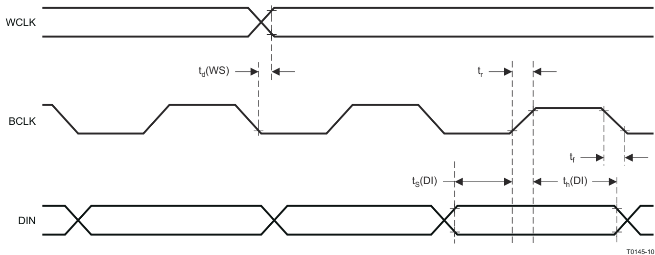
图 5-1. 主模式下的 I²S/LJF/RJF 时序
