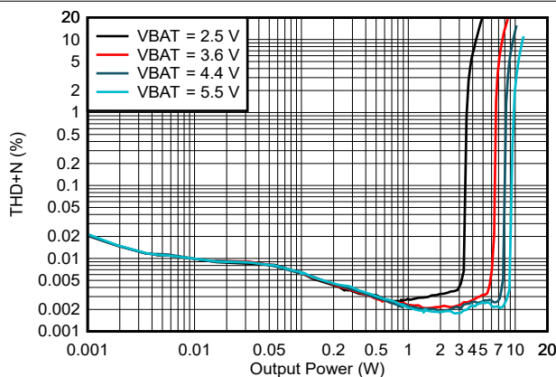
图 7-2. THDN 与输出功率间的关系
