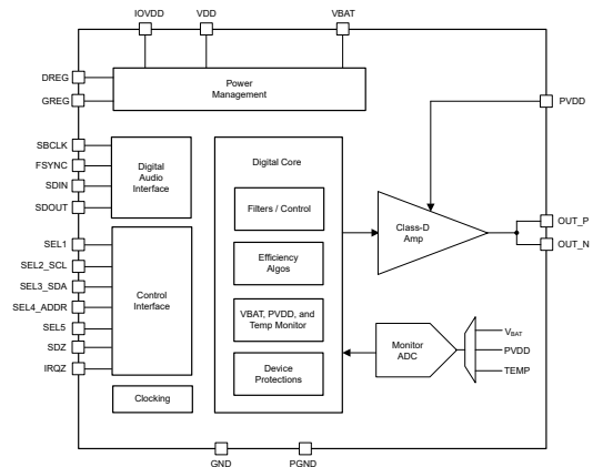
功能方框图
