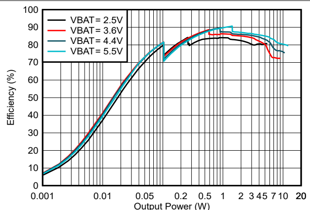
图 7-3. 效率与输出功率间的关系
