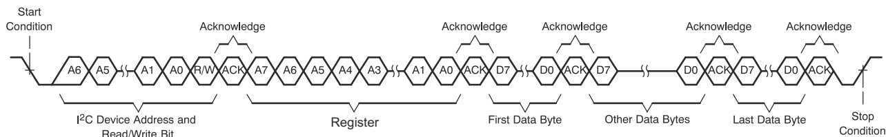
图 6-10. I 2 C 多字节写入传输
