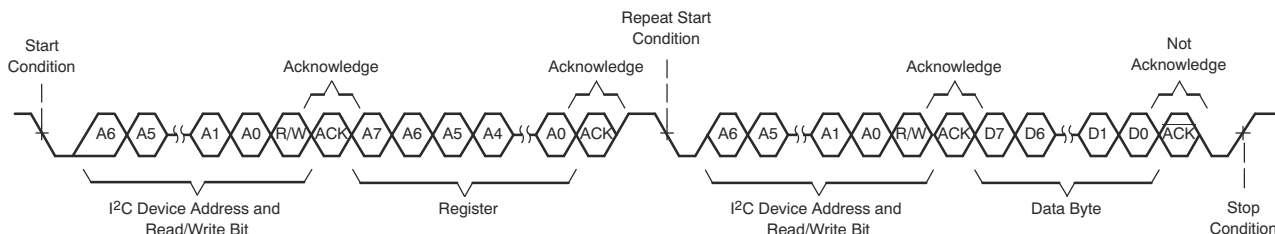
图 6-11. I 2 C 单字节读取传输
