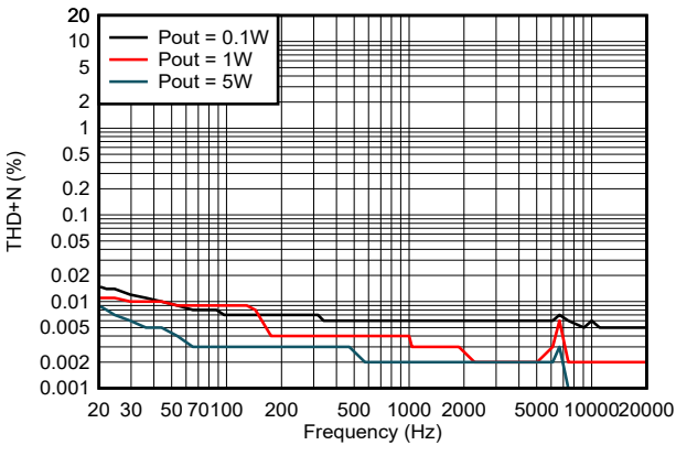
图 5-2. THD+N 与频率间的关系
