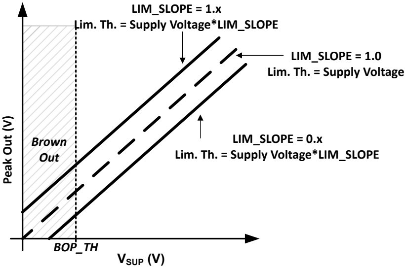
图 6-4. 具有动态电源余量的限制器
