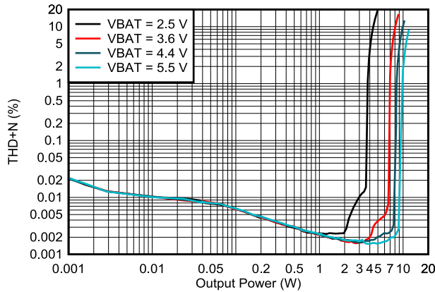
R_L = 8\Omega 1S 升压模式 HW 引脚控制
