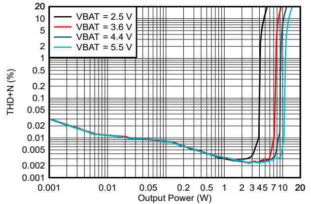
R_L = 4\Omega 1S 升压模式 HW 引脚控制
