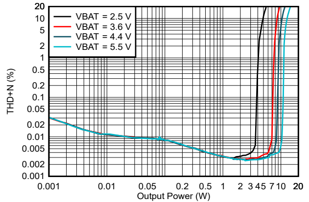
R_L = 4\Omega 1S 升压模式
