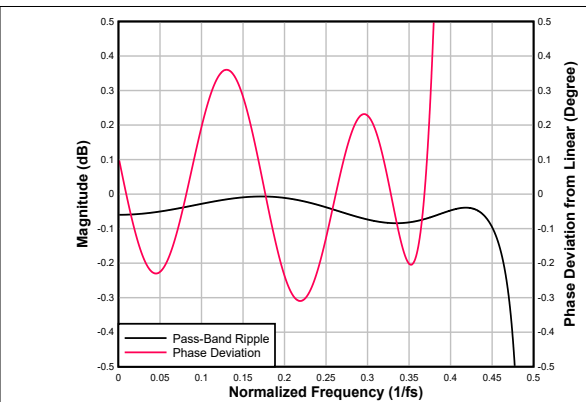
图 6-29. 低延迟内插滤波器通带纹波和相位偏差
