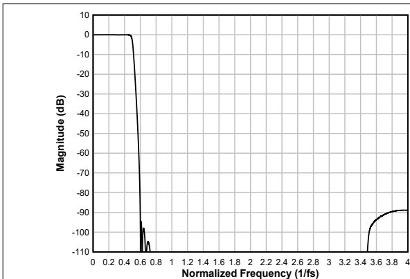
图 6-30. 低延迟内插滤波器幅度响应
