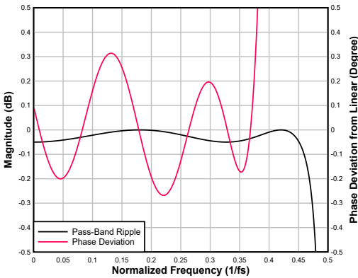
图 6-47. 低延迟内插滤波器通带纹波和相位偏差
