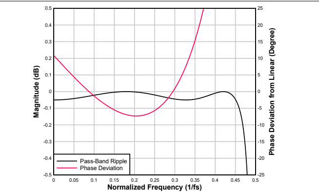
图 6-57. 超低延迟内插滤波器通带纹波和相位偏差
