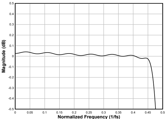
图 6-65. 线性相位抽取滤波器通带纹波
