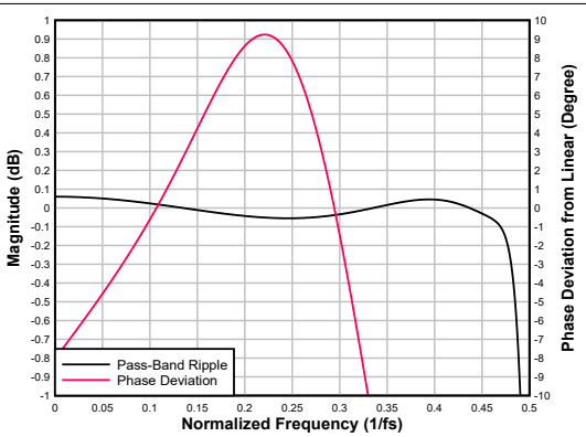
图 6-89. 低延迟抽取滤波器通带纹波和相位偏差
