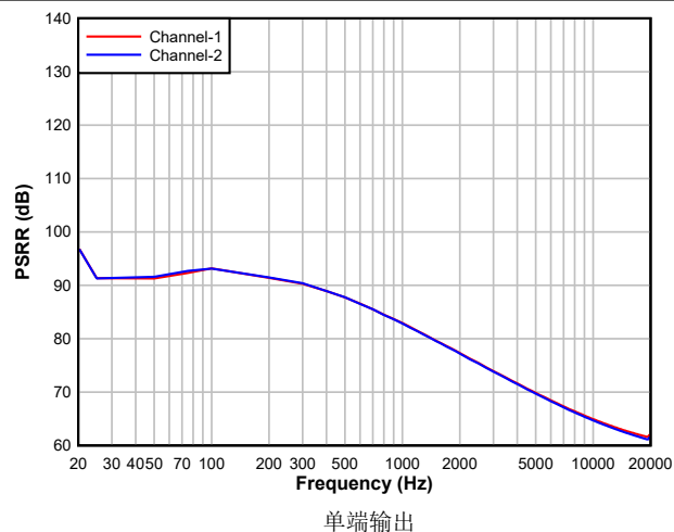
图 5-19. DAC PSRR 与频率间的关系
