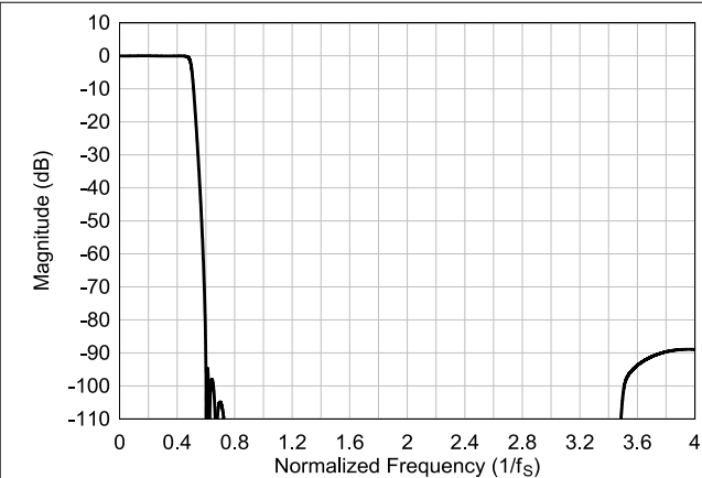
图 6-50. 超低延迟内插滤波器幅度响应
