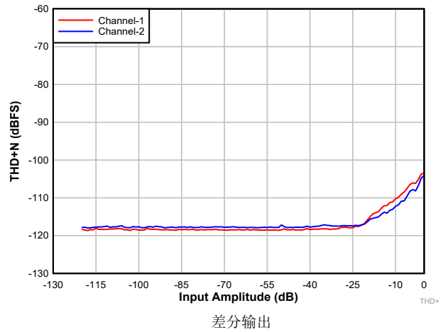
图 8-3. DAC THD+N 级别与输入间的关系
