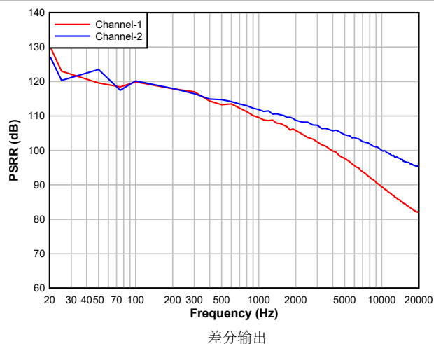
图 5-18. DAC PSRR 与频率间的关系
