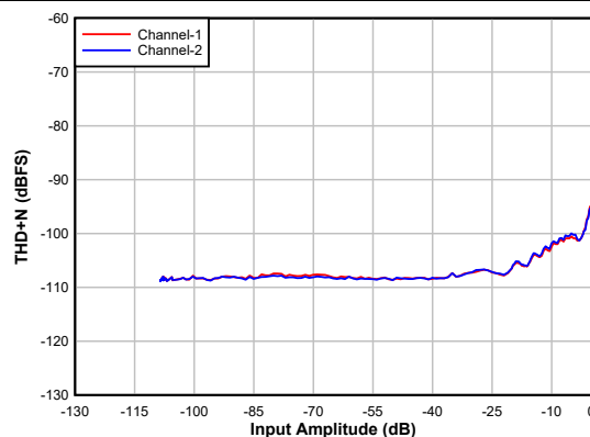
单端输出
