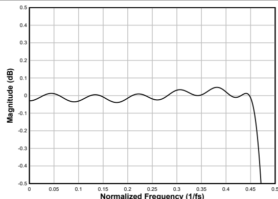
图 6-69. 线性相位抽取滤波器通带纹波
