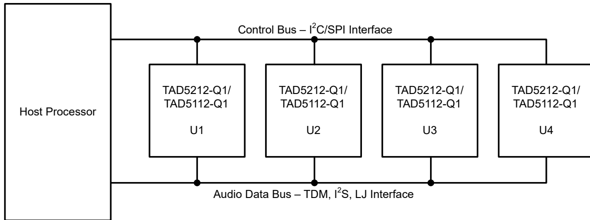
图 6-13. 多个 TAD5212-Q1 器件具有共享控制和音频数据总线
