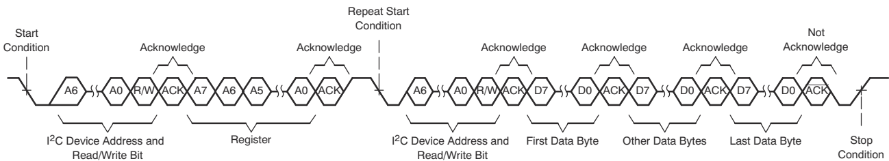
图 6-105. I 2 C 多字节读取传输
