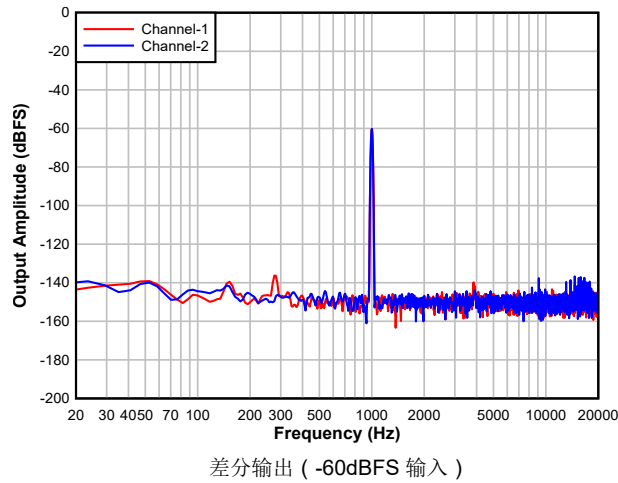
图 8-2. 具有-60dBFS 输入的 DAC FFT
