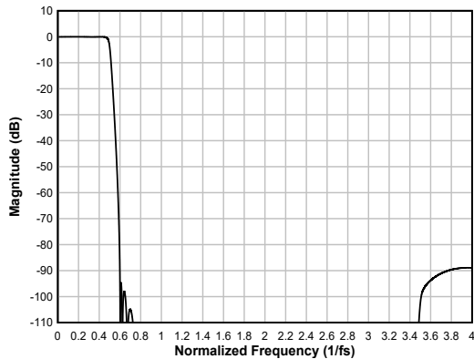
图 6-40. 低延迟内插滤波器幅度响应
