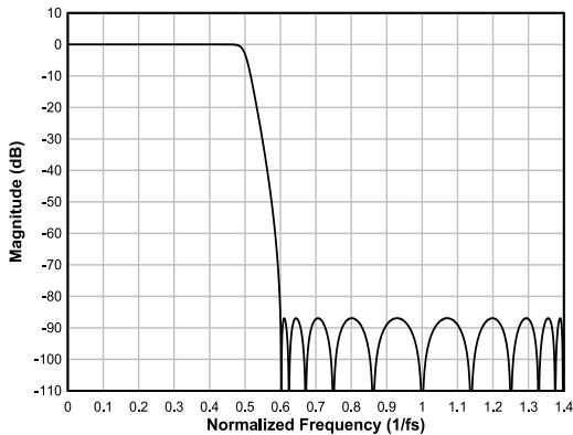
图 6-48. 低延迟内插滤波器幅度响应
