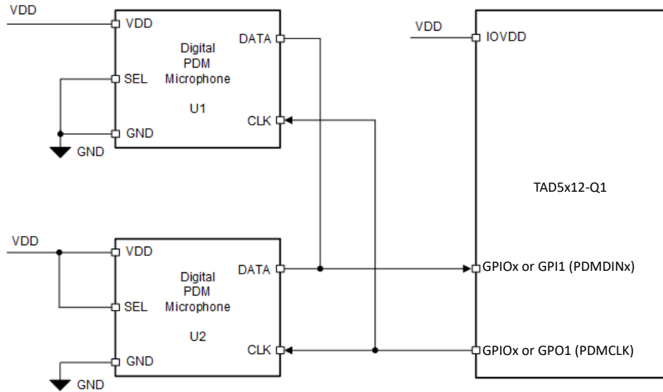
图 6-18. TAD5212-Q1 的数字 PDM 麦克风连接图
