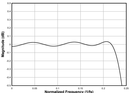
图 6-75. 线性相位抽取滤波器通带纹波
