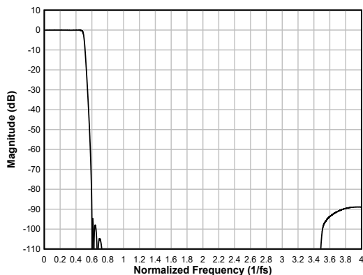
图 6-42. 低延迟内插滤波器幅度响应
