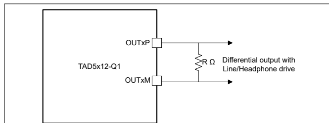
图 6-14. 差分输出连接 (OUT1x_CFG[2:0] = 3'b000)
