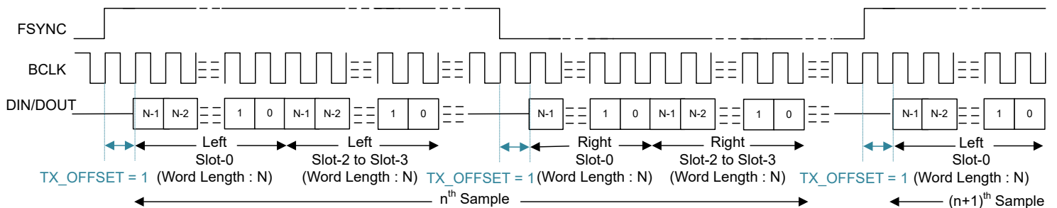
图 6-12. LJ 协议时序 (TX_OFFSET = 1 且 BCLK_POL = 1)
