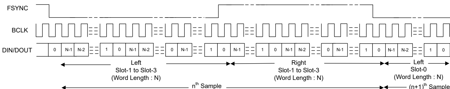
图 6-7. I²S 协议时序 (无空闲 BCLK 周期, PASI_TX_OFFSET = 0)
