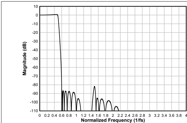
图 6-80. 低延迟抽取滤波器幅度响应
