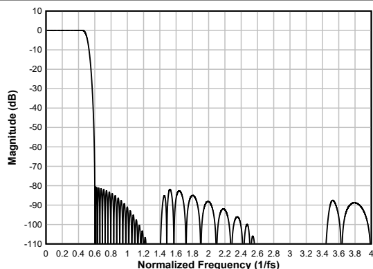
图 6-68. 线性相位抽取滤波器幅度响应
