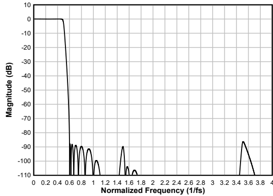
图 6-94. 超低延迟抽取滤波器幅度响应
