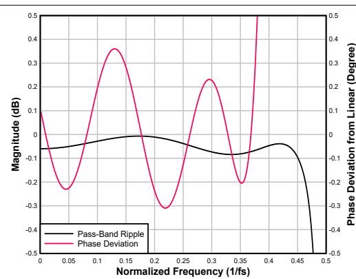
图 6-45. 低延迟内插滤波器通带纹波和相位偏差
