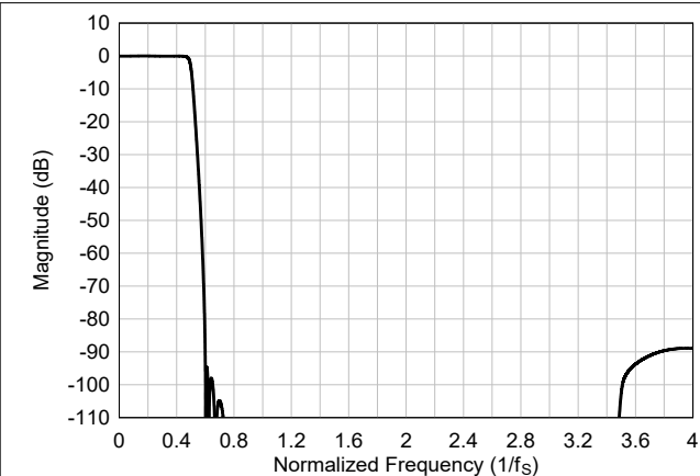
图 6-52. 超低延迟内插滤波器幅度响应
