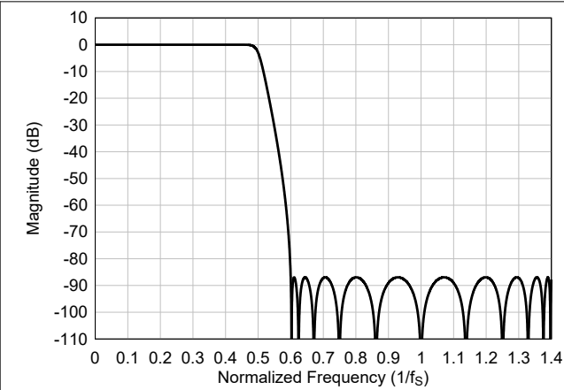
图 6-58. 超低延迟内插滤波器幅度响应
