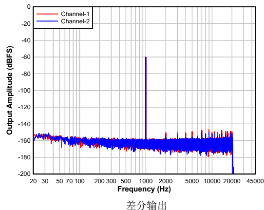
图 5-16. 具有-60dBFS 输入的 DAC FFT
