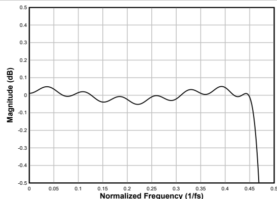
图 6-71. 线性相位抽取滤波器通带纹波
