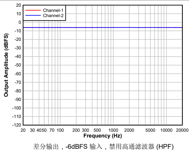
图 5-20. DAC 频率响应
