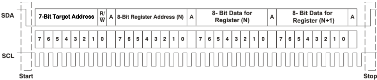
图 6-101. 典型的 I²C 序列
