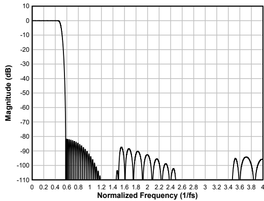
图 6-26. 线性相位内插滤波器幅度响应
