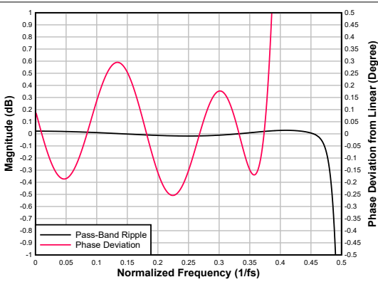
图 6-87. 低延迟抽取滤波器通带纹波和相位偏差
