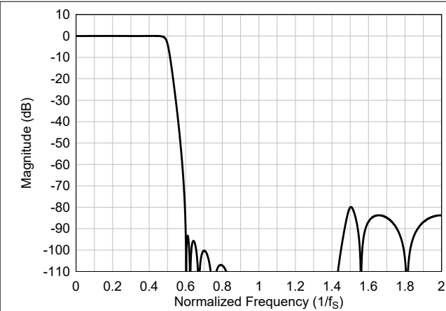
图 6-56. 超低延迟内插滤波器幅度响应
