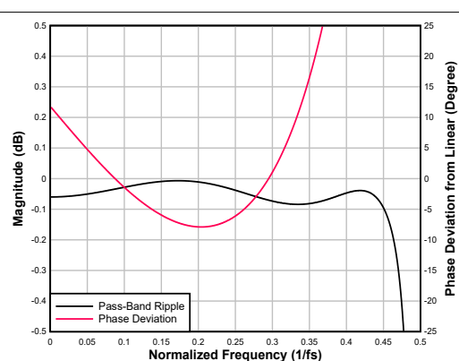
图 6-55. 超低延迟内插滤波器通带纹波和相位偏差
