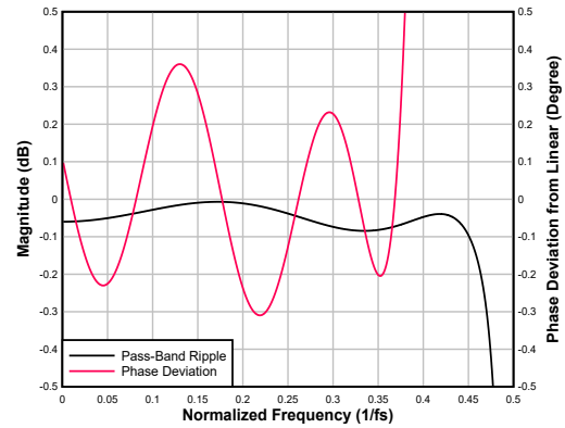
图 6-41. 低延迟内插滤波器通带纹波和相位偏差
