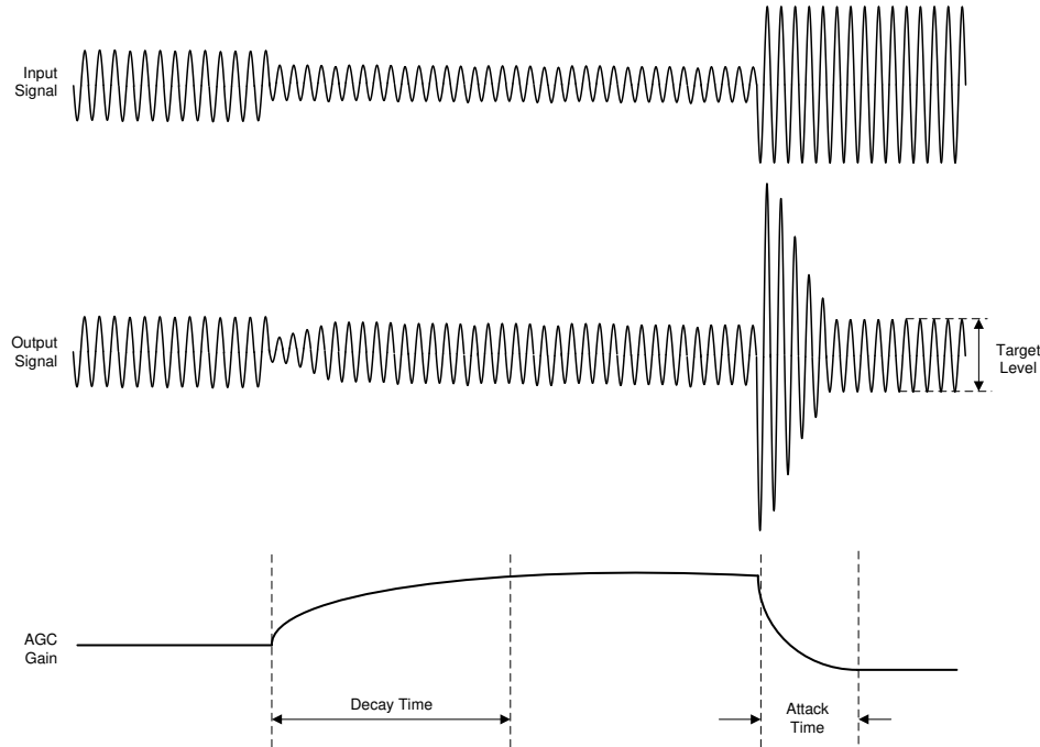
图 6-100. AGC 特性
