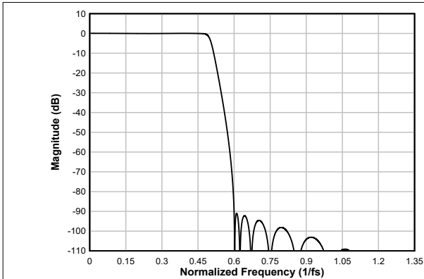
图 6-88. 低延迟抽取滤波器幅度响应
