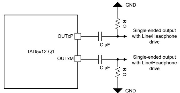
图 6-17. 立体声单端输出连接 (OUT1x_CFG[2:0] = 3'b001)
