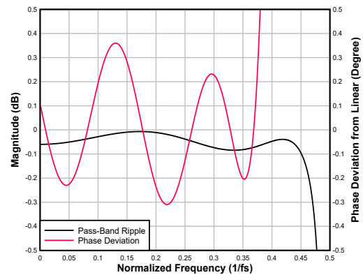
图 6-43. 低延迟内插滤波器通带纹波和相位偏差
