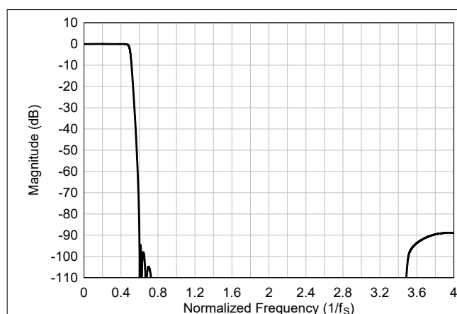
图 6-54. 超低延迟内插滤波器幅度响应
