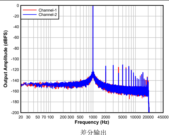
图 5-17. 具有-1dBFS 输入的 DAC FFT
