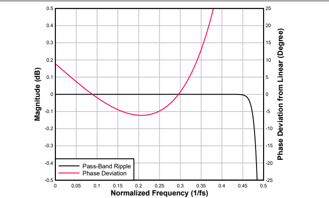
图 6-59. 超低延迟内插滤波器通带纹波和相位偏差
