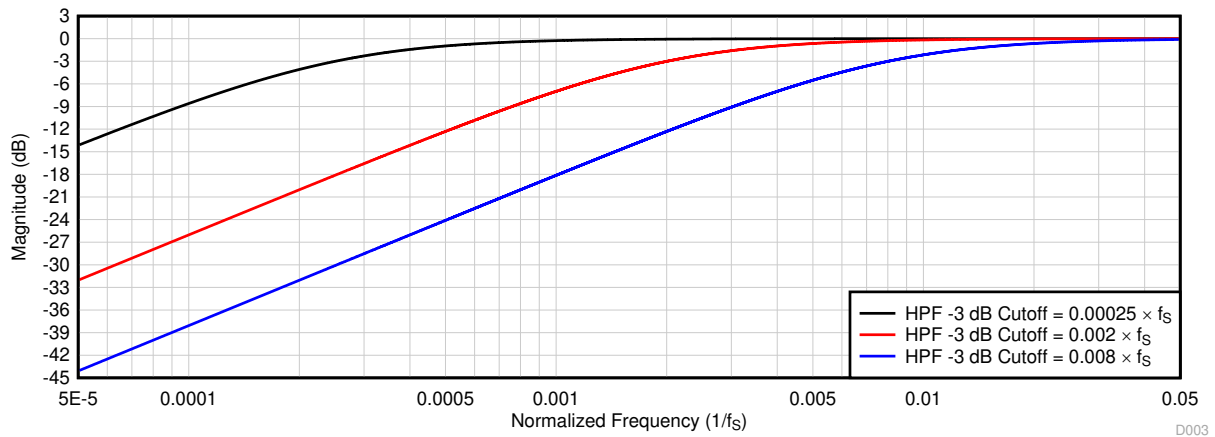
图 6-21. HPF 滤波器频率响应图
