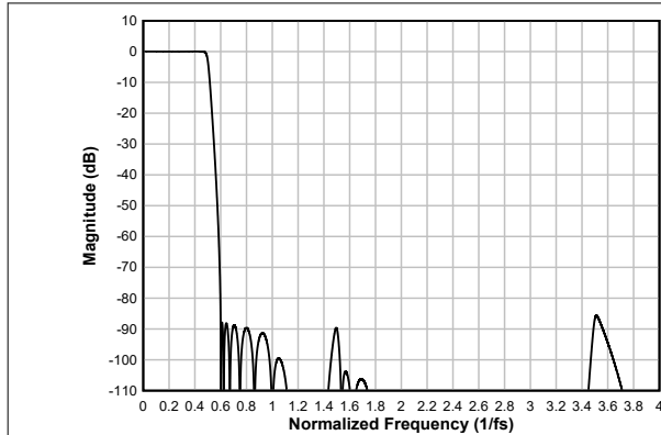
图 6-96. 超低延迟抽取滤波器幅度响应
