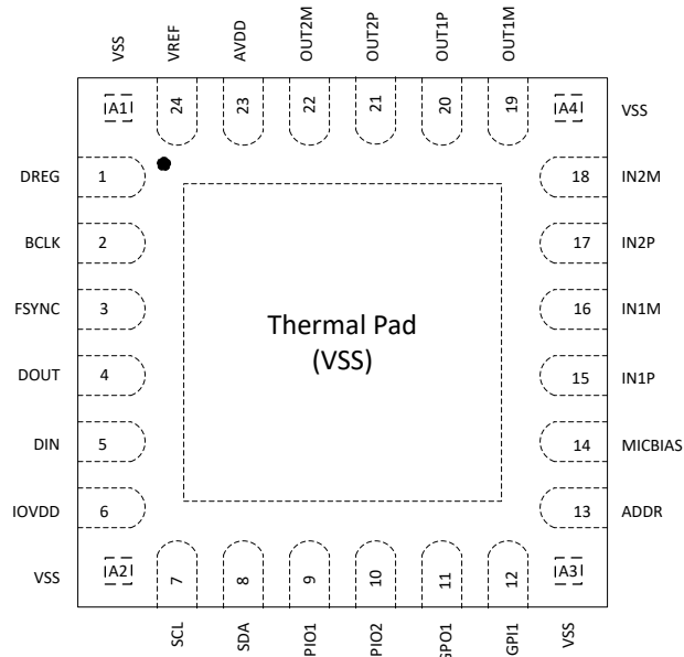
图 4-1. 带有外露散热焊盘和转角引脚的 24 引脚 QFN 封装，顶视图
