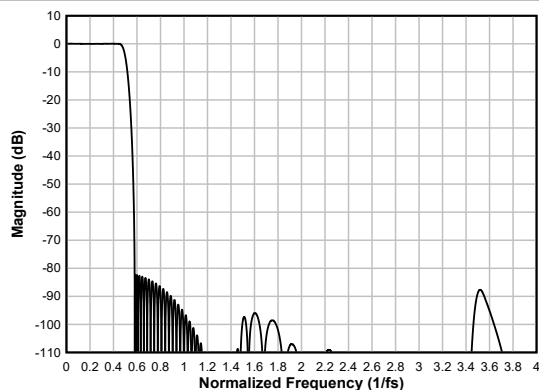
图 6-70. 线性相位抽取滤波器幅度响应
