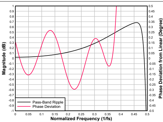
图 6-81. 低延迟抽取滤波器通带纹波和相位偏差
