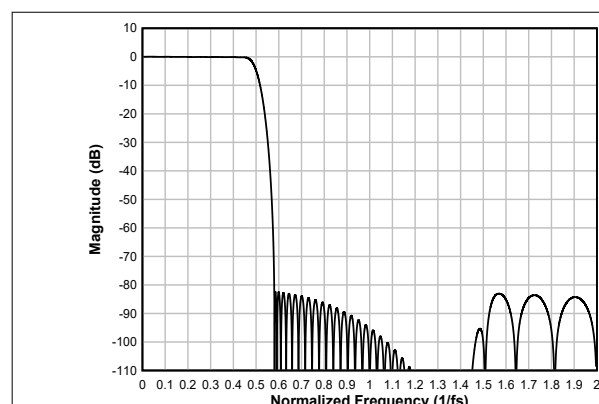
图 6-32. 线性相位内插滤波器幅度响应
