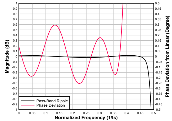
图 6-85. 低延迟抽取滤波器通带纹波和相位偏差
