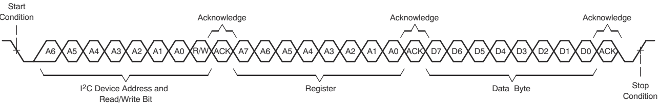
图 6-102. I²C 单字节写入传输
