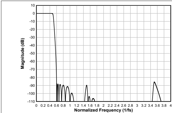
图 6-86. 低延迟抽取滤波器幅度响应
