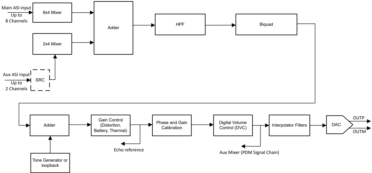
图 6-20. DAC 信号链处理流程图
