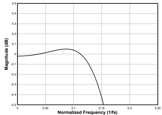
图 6-79. 线性相位抽取滤波器通带纹波
