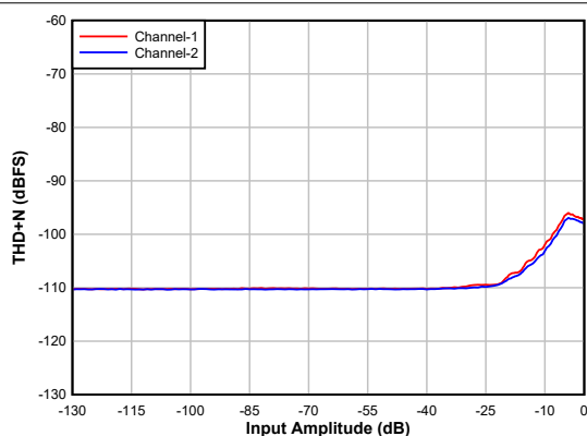
伪差分输出
