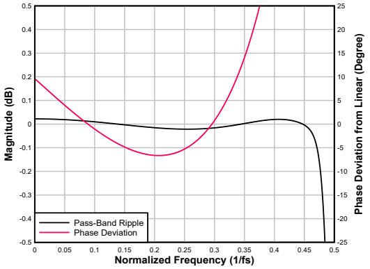
图 6-95. 超低延迟抽取滤波器通带纹波和相位偏差
