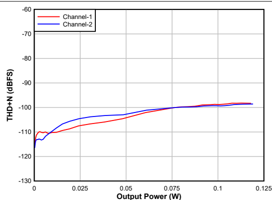
差分接收器输出，32 \Omega 负载
