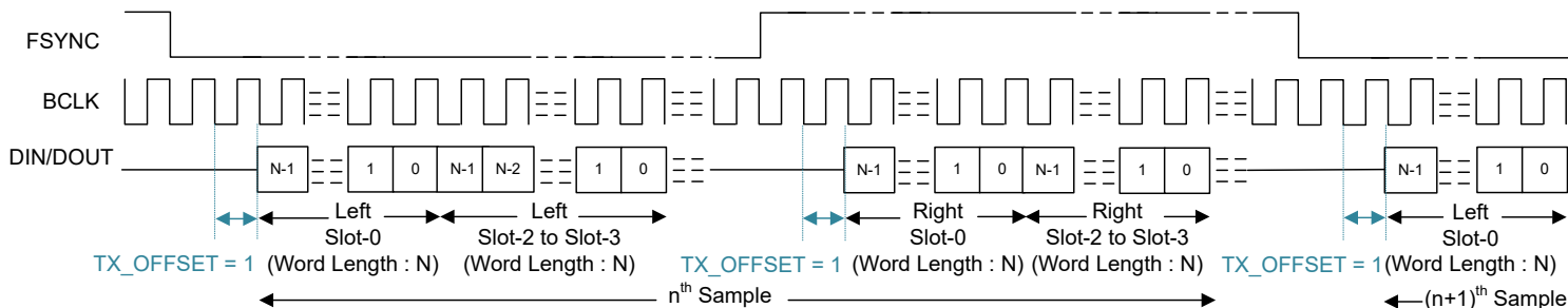
图 6-6. I²S 协议时序 (PASI_TX_OFFSET = 1)
