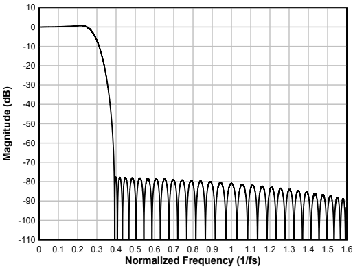
图 6-36. 线性相位内插滤波器幅度响应
