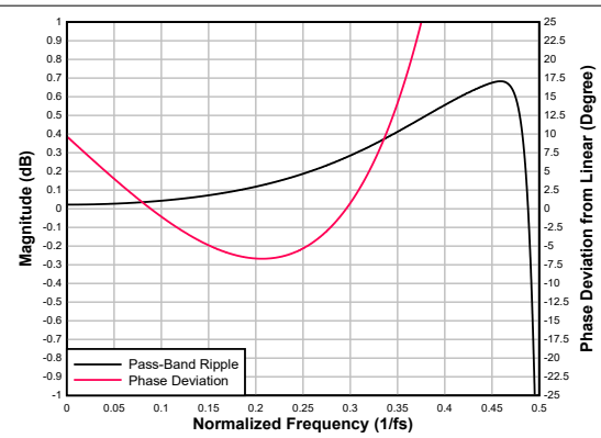
图 6-91. 超低延迟抽取滤波器通带纹波和相位偏差
