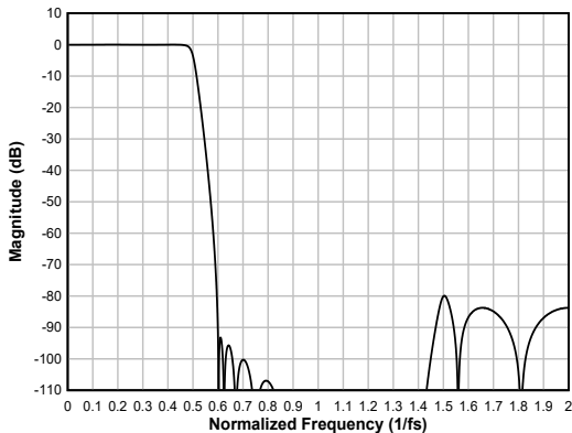
图 6-46. 低延迟内插滤波器幅度响应
