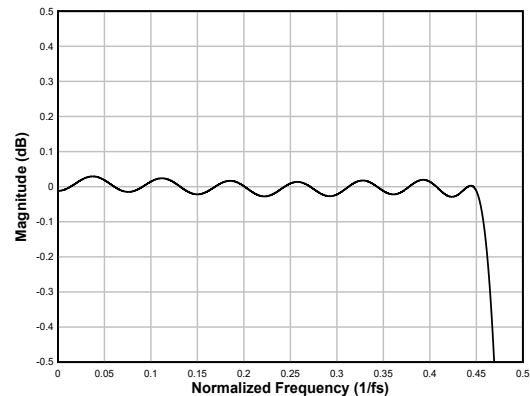
图 6-27. 线性相位内插滤波器通带纹波
