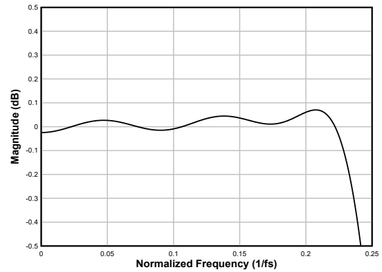
图 6-77. 线性相位抽取滤波器通带纹波
