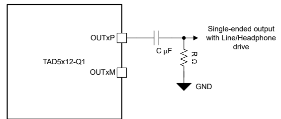
图 6-15. OUT1P 上的单声道单端输出连接 (OUT1x_CFG[2:0] = 3'b010)
