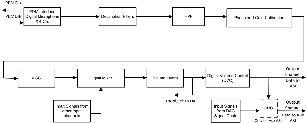
图 6-60. PDM 录音信号链处理流程图
