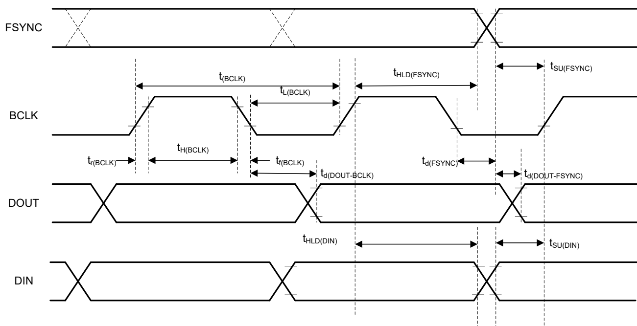
图 5-3. TDM (其中 BCLK_POL = 1)、I²S 和 LJ 接口时序图
