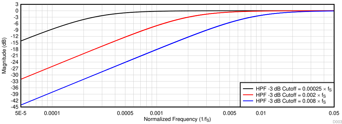
图 6-61. HPF 滤波器频率响应图
