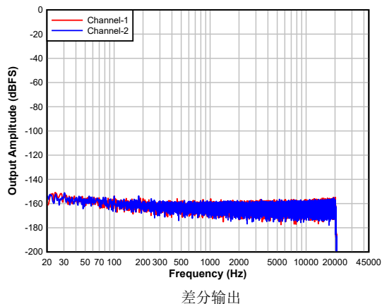
图 5-15. 具有空闲通道输入的 DAC FFT
