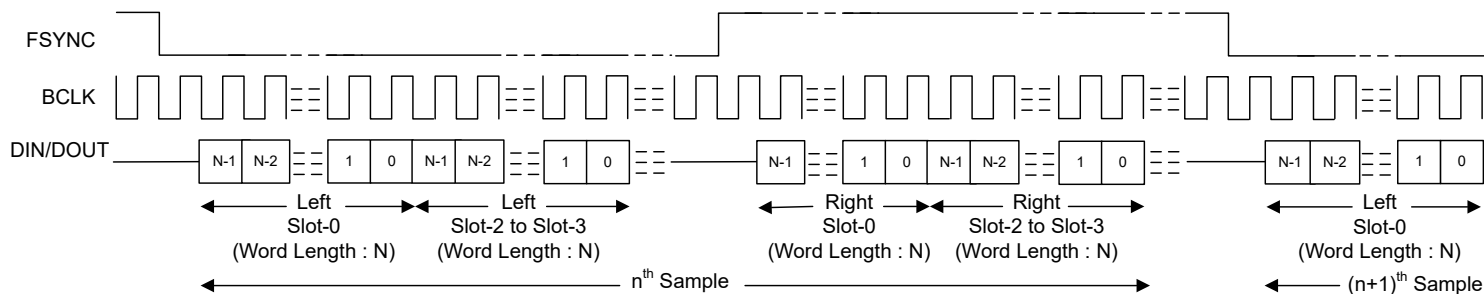
图 6-5. I²S 模式标准协议时序 (PASI_TX_OFFSET = 0)
