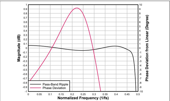
图 6-89. 低延迟抽取滤波器通带纹波和相位偏差
