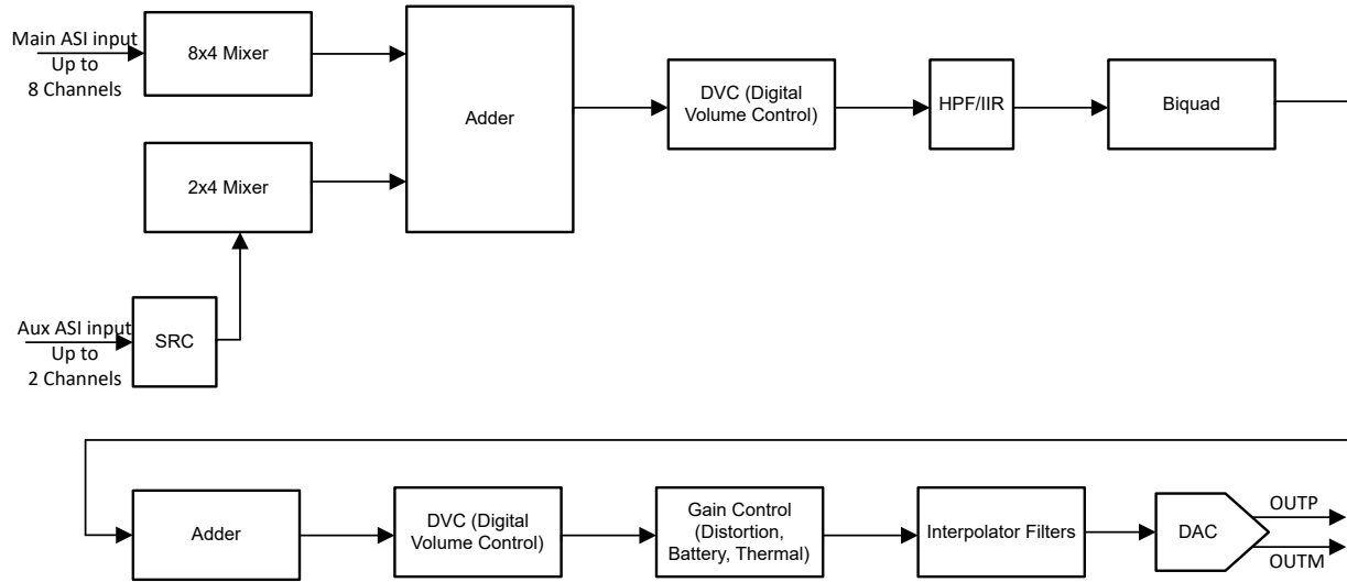
图 6-20. DAC 信号链处理流程图
