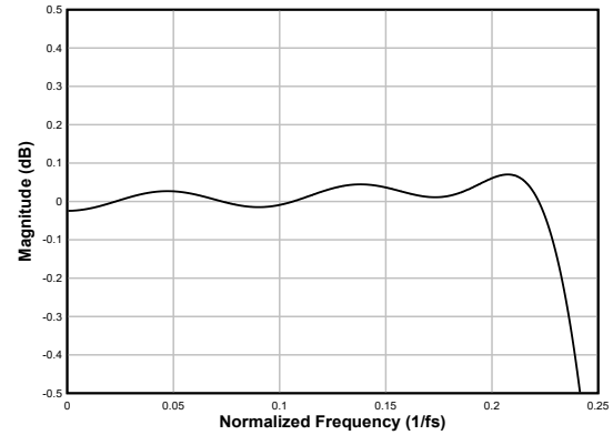
图 6-77. 线性相位抽取滤波器通带纹波
