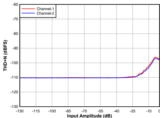
伪差分输出
