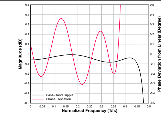
图 6-41. 低延迟内插滤波器通带纹波和相位偏差
