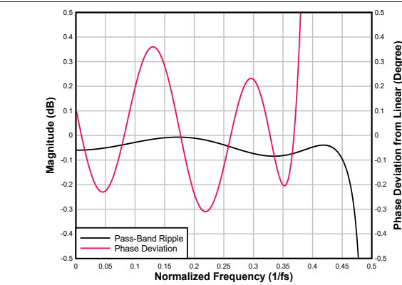
图 6-43. 低延迟内插滤波器通带纹波和相位偏差
