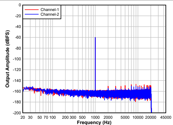
差分输出
