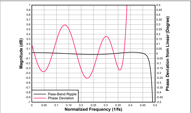
图 6-87. 低延迟抽取滤波器通带纹波和相位偏差
