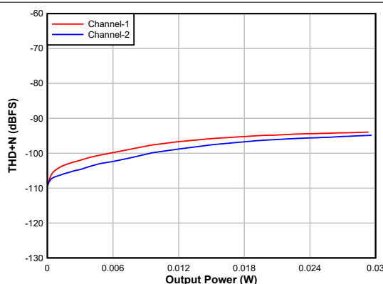
单端耳机输出，16 \Omega 负载
