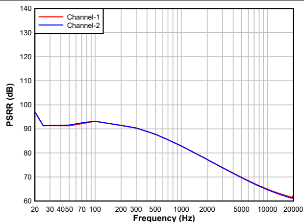
图 5-19. DAC PSRR 与频率间的关系
