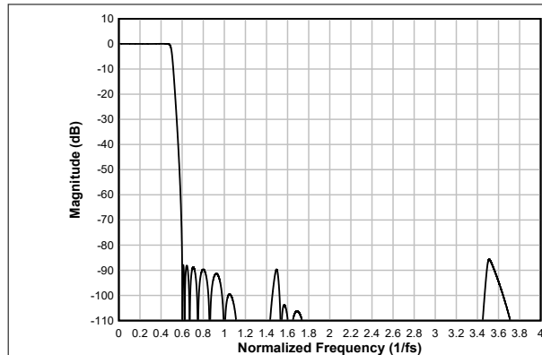
图 6-96. 超低延迟抽取滤波器幅度响应
