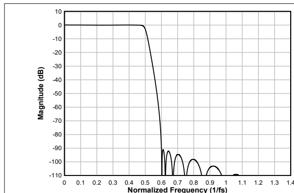
图 6-98. 超低延迟抽取滤波器幅度响应
