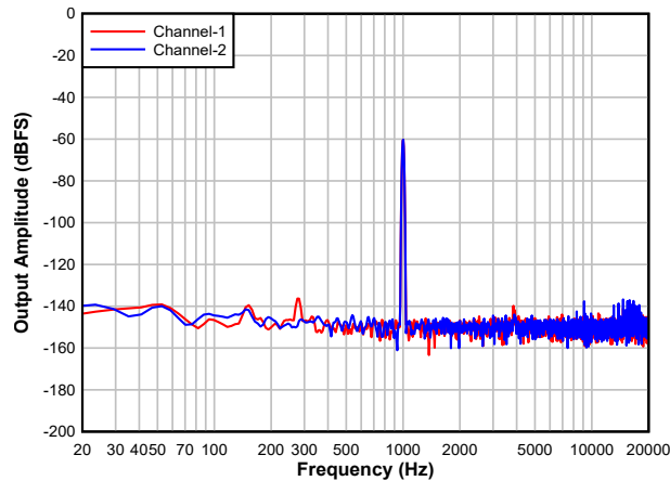
图 8-2. 具有 -60dBFS 输入的 DAC FFT
