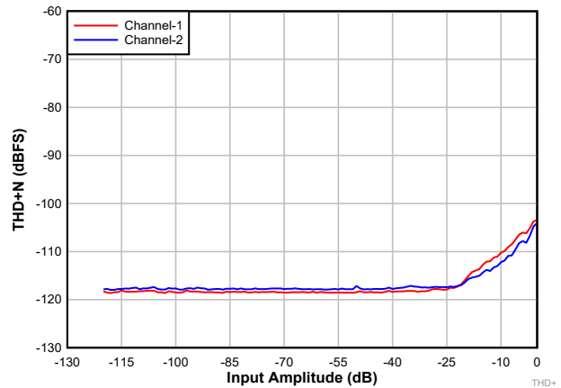
图 8-3. DAC THD+N 级别与输入间的关系
