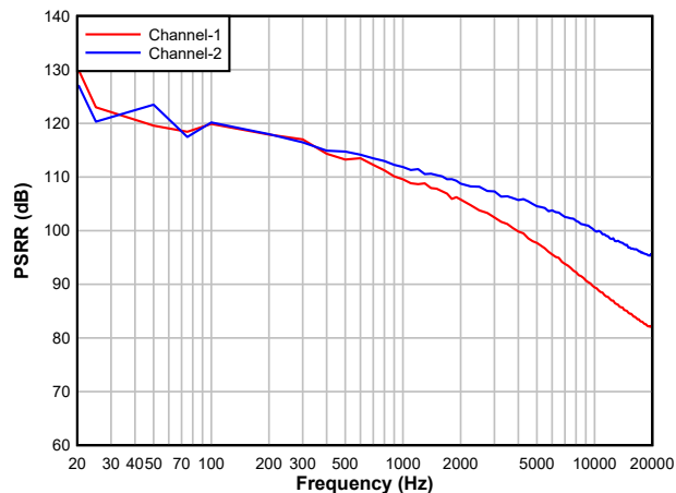
图 5-18. DAC PSRR 与频率间的关系
