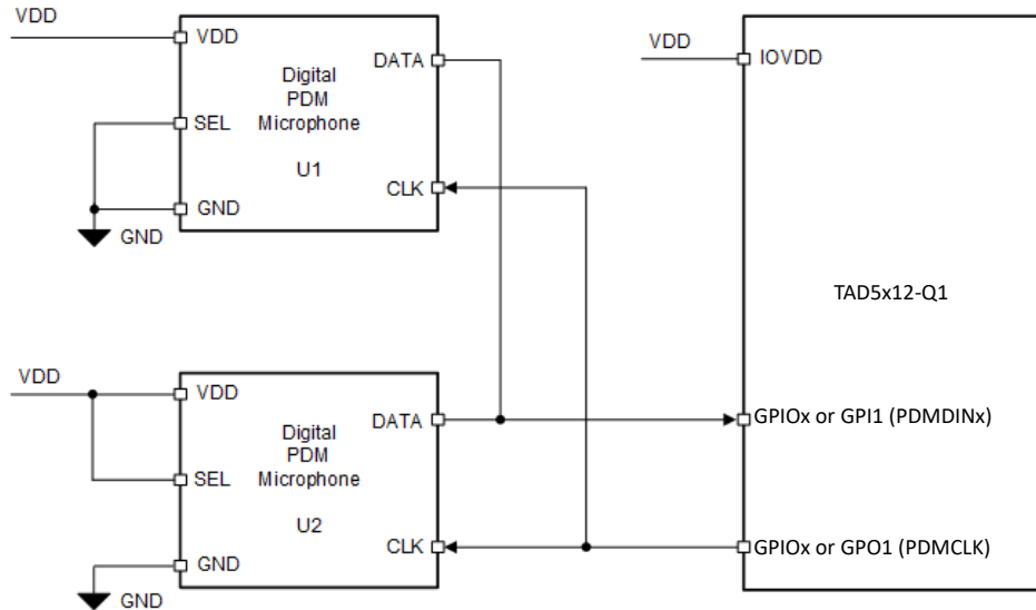
图 6-18. TAD5112-Q1 的数字 PDM 麦克风连接图
