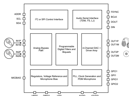
简化版方框图
