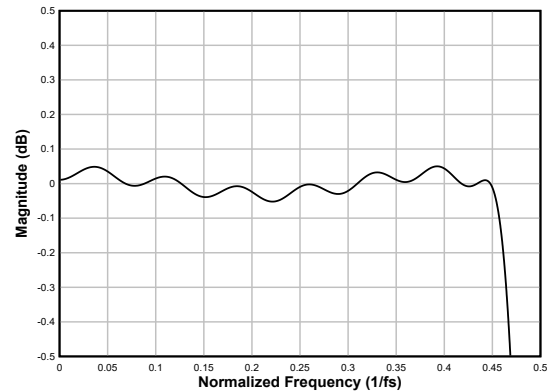
图 6-71. 线性相位抽取滤波器通带纹波
