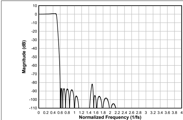
图 6-80. 低延迟抽取滤波器幅度响应
