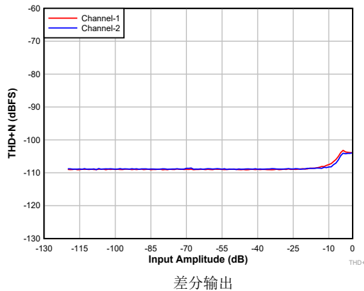
图 8-2. DAC THD + N 级别与输入间的关系
