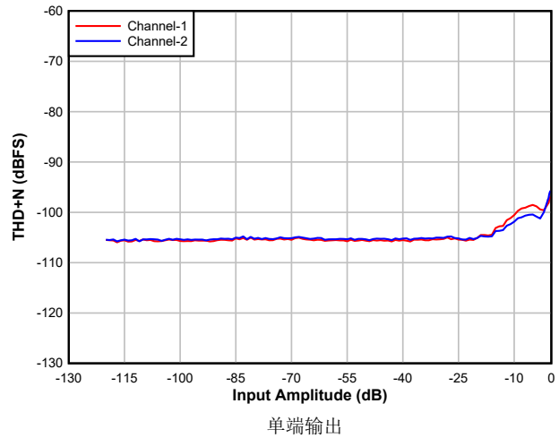
图 5-6. DAC THD+N 级别与输入间的关系
