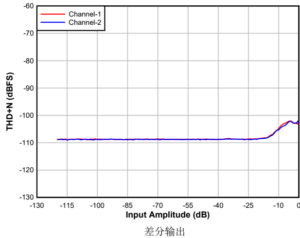
图 5-5. DAC THD + N 级别与输入间的关系
