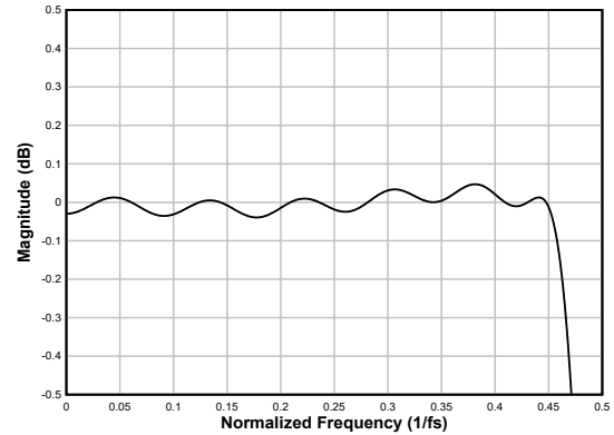
图 6-69. 线性相位抽取滤波器通带纹波
