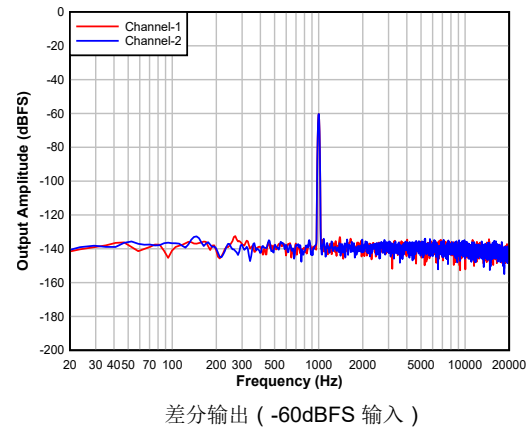
图 8-3. 具有 -60dBFS 输入的 DAC FFT
