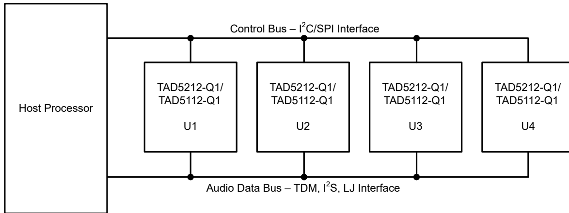
图 6-13. 多个 TAD5112-Q1 器件具有共享控制和音频数据总线
