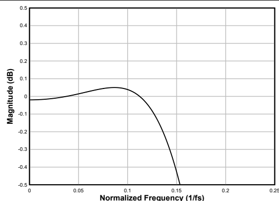
图 6-79. 线性相位抽取滤波器通带纹波
