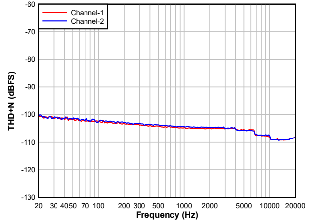
图 5-10. DAC THD+N 级别与频率间的关系
