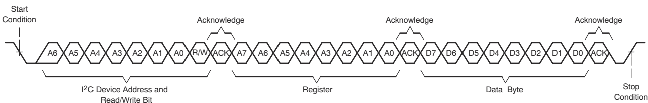
图 6-102. I²C 单字节写入传输
