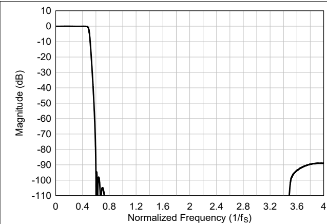
图 6-52. 超低延迟内插滤波器幅度响应
