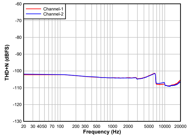
图 5-10. DAC THD+N 级别与频率间的关系
