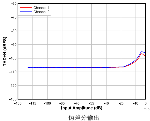
图 5-7. DAC THD+N 级别与输入间的关系
