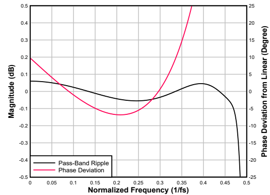
图 6-100. 超低延迟抽取滤波器通带纹波和相位偏差
