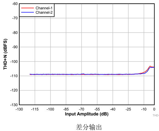
图 8-2. DAC THD + N 级别与输入间的关系
