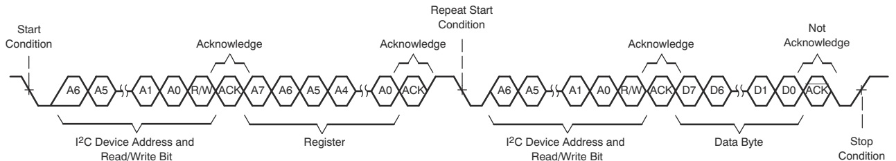
图 6-105. I 2 C 单字节读取传输
