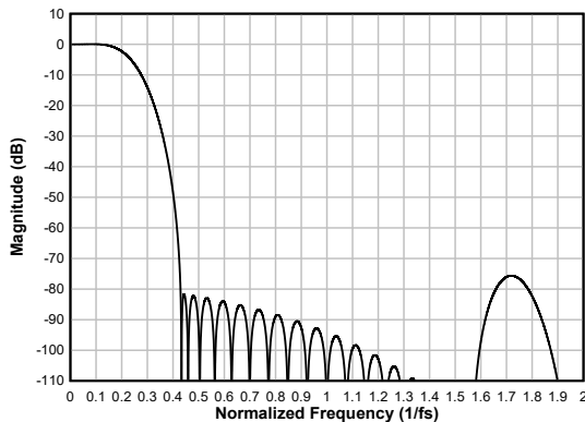
图 6-79. 线性相位抽取滤波器幅度响应
