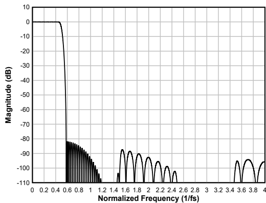
图 6-27. 线性相位内插滤波器幅度响应
