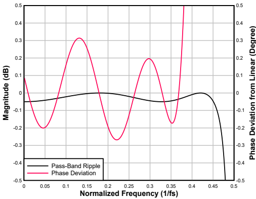
图 6-48. 低延迟内插滤波器通带纹波和相位偏差
