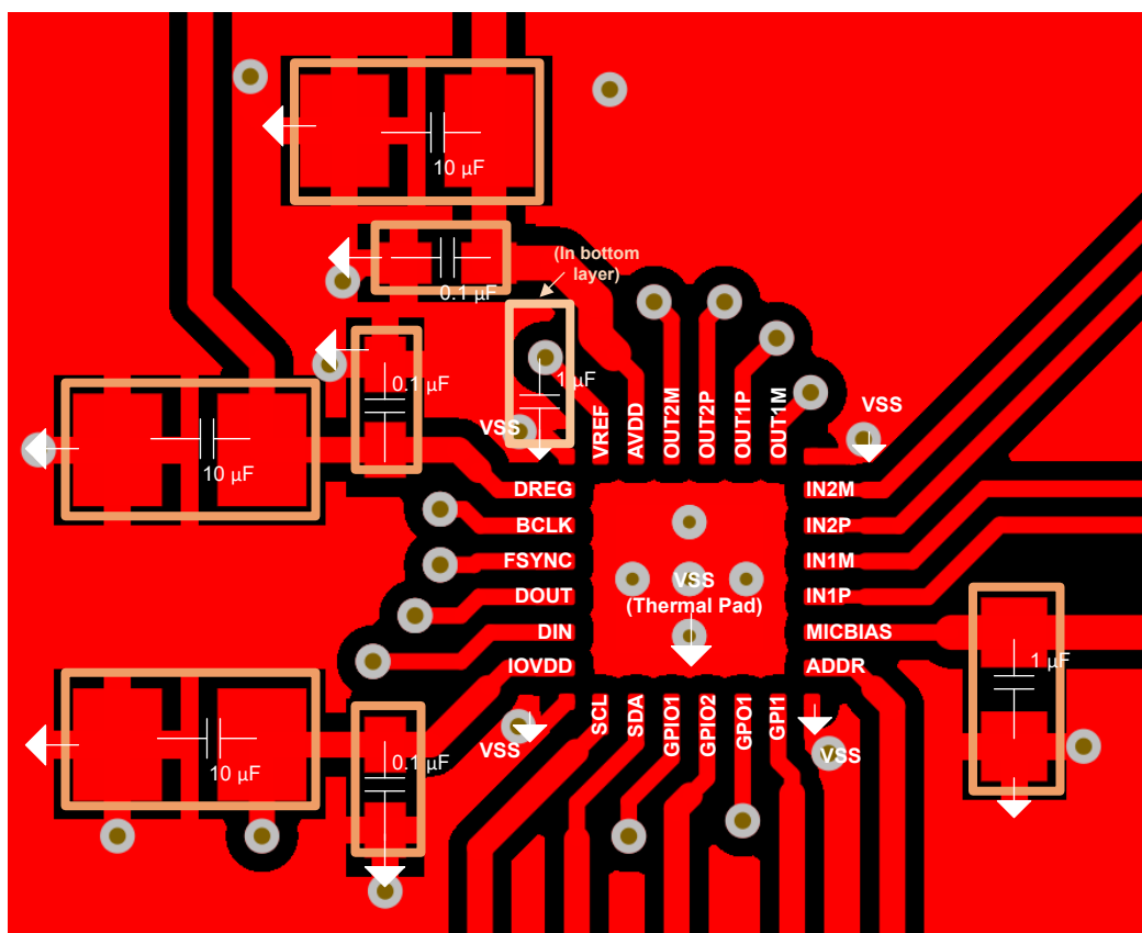
图 8-5. 示例布局
