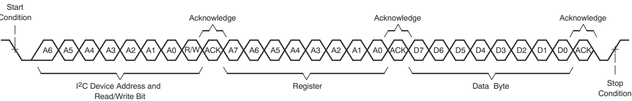
图 6-103. I²C 单字节写入传输
