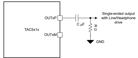
图 6-16. OUT1P 上的单声道单端输出连接 (OUT1x_CFG[2:0] = 3'b010)
