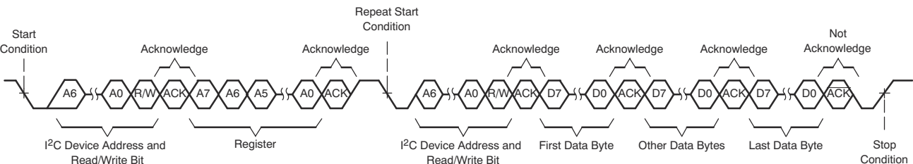
图 6-106. I 2 C 多字节读取传输
