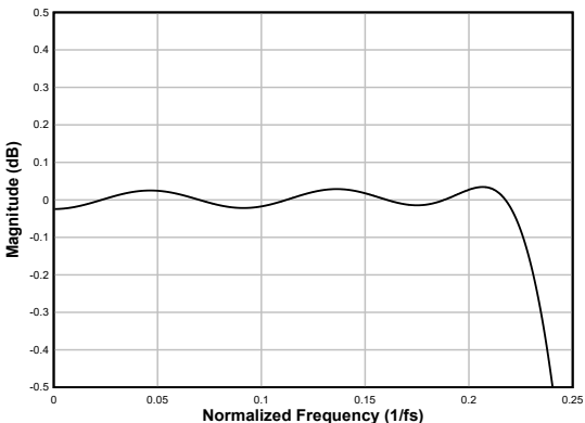
图 6-76. 线性相位抽取滤波器通带纹波
