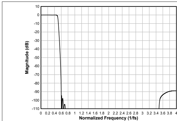
图 6-45. 低延迟内插滤波器幅度响应
