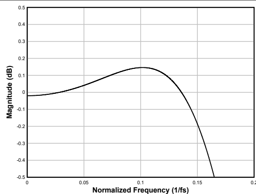
图 6-40. 线性相位内插滤波器通带纹波
