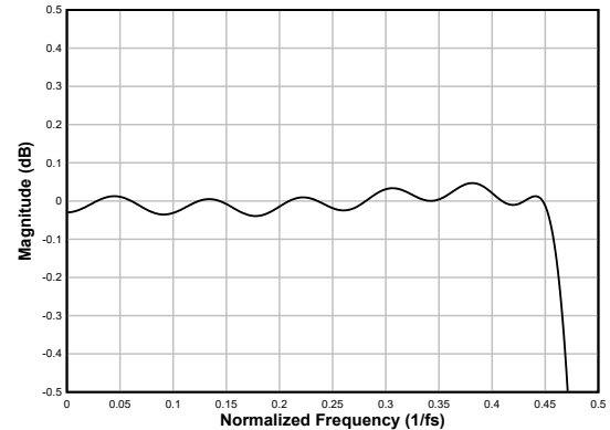
图 6-70. 线性相位抽取滤波器通带纹波
