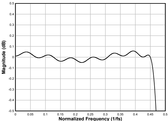
图 6-74. 线性相位抽取滤波器通带纹波
