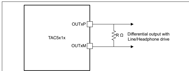
图 6-15. 差分输出连接 (OUT1x_CFG[2:0] = 3'b000)
