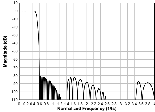
图 6-69. 线性相位抽取滤波器幅度响应
