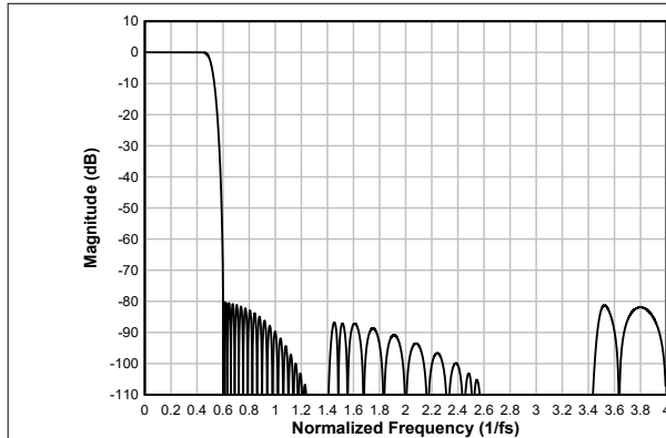
图 6-63. 线性相位抽取滤波器幅度响应
