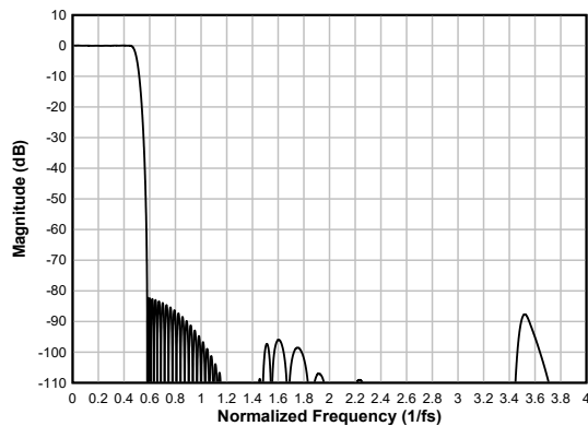
图 6-71. 线性相位抽取滤波器幅度响应
