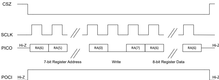
图 6-107. SPI 单字节写入传输
