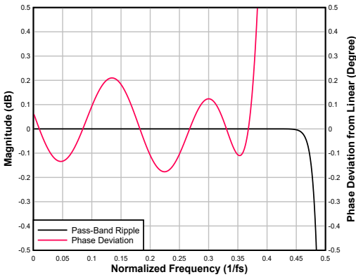
图 6-50. 低延迟内插滤波器通带纹波和相位偏差
