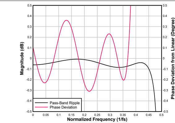
图 6-44. 低延迟内插滤波器通带纹波和相位偏差
