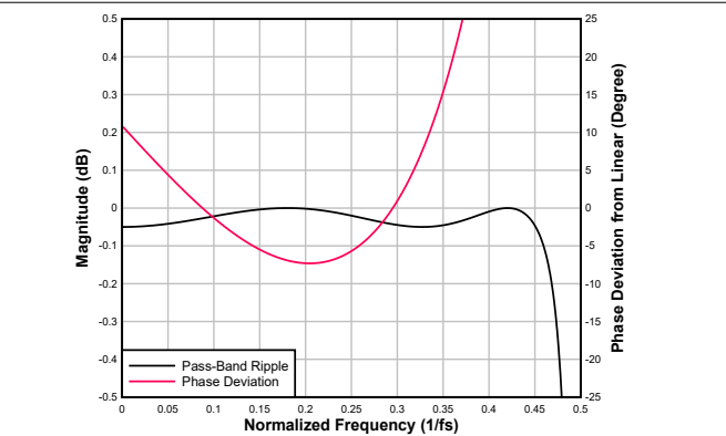
图 6-58. 超低延迟内插滤波器通带纹波和相位偏差
