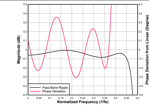
图 6-42. 低延迟内插滤波器通带纹波和相位偏差
