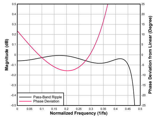
图 6-56. 超低延迟内插滤波器通带纹波和相位偏差
