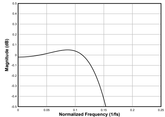
图 6-80. 线性相位抽取滤波器通带纹波
