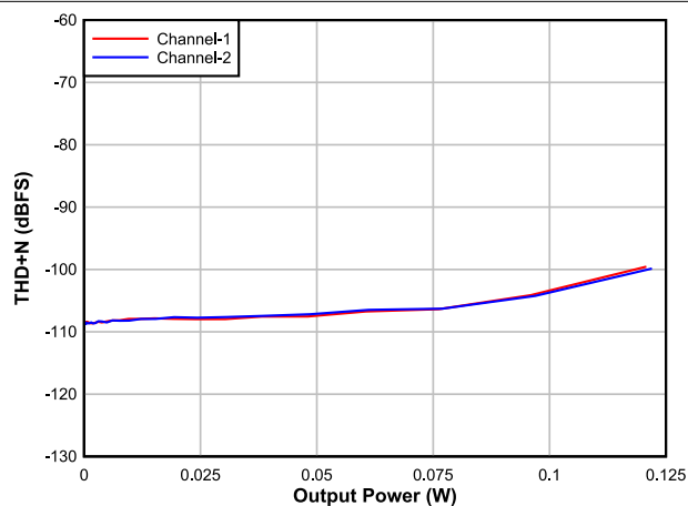
差分接收器输出，32 \Omega 负载
