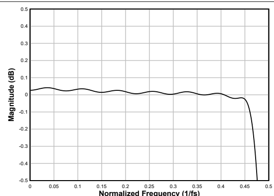
图 6-64. 线性相位抽取滤波器通带纹波
