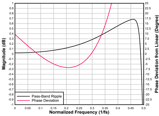
图 6-94. 超低延迟抽取滤波器通带纹波和相位偏差
