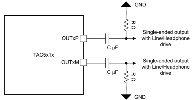
图 6-18. 立体声单端输出连接 (OUT1x_CFG[2:0] = 3'b001)
