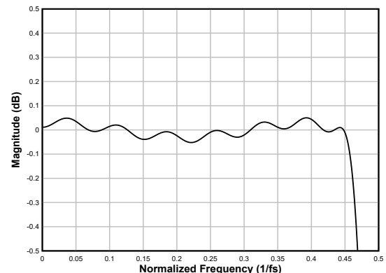
图 6-72. 线性相位抽取滤波器通带纹波
