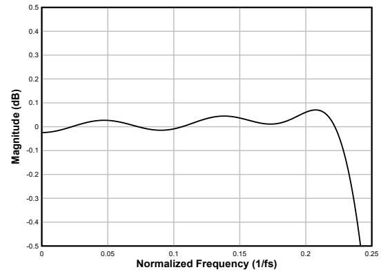
图 6-78. 线性相位抽取滤波器通带纹波
