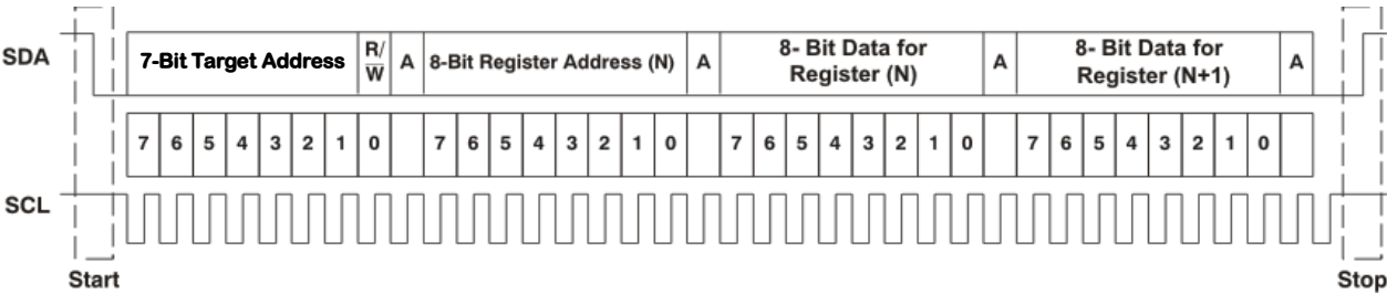
图 6-102. 典型的 I²C 序列
