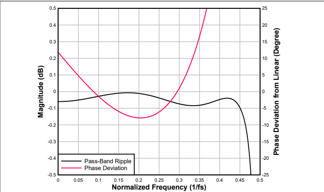
图 6-52. 超低延迟内插滤波器通带纹波和相位偏差
