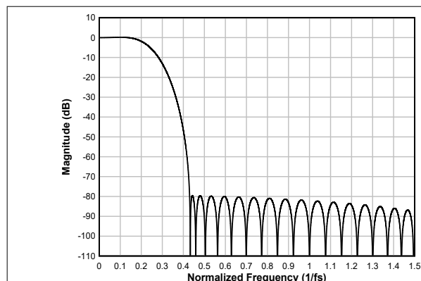
图 6-39. 线性相位内插滤波器幅度响应
