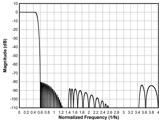
图 6-25. 线性相位内插滤波器幅度响应
