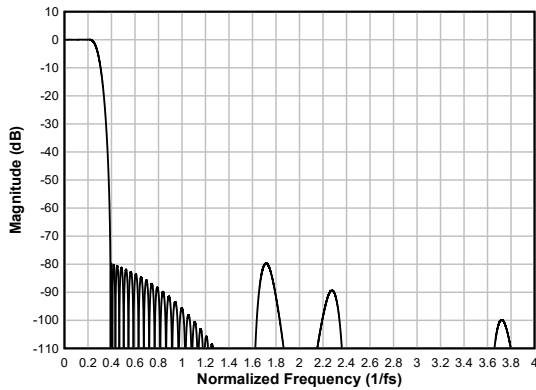
图 6-77. 线性相位抽取滤波器幅度响应
