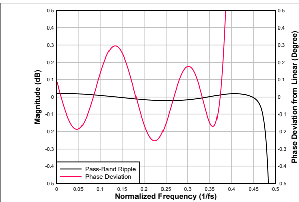
图 6-47. 低延迟抽取滤波器通带纹波和相位偏差
