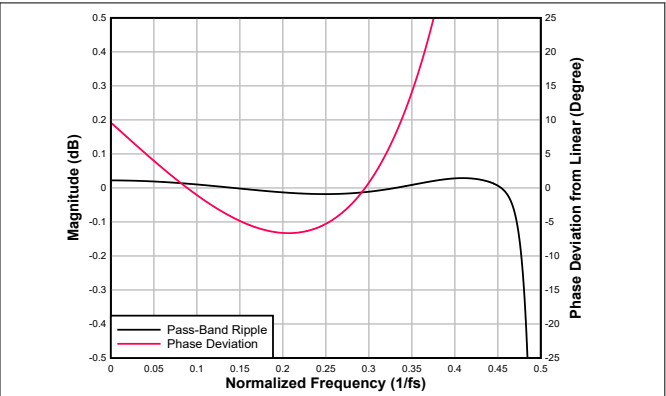
图 6-59. 超低延迟抽取滤波器通带纹波和相位偏差
