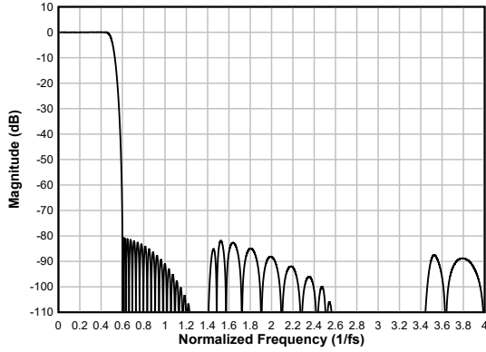
图 6-30. 线性相位抽取滤波器幅度响应
