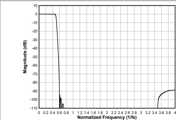
图 6-85. 低延迟内插滤波器幅度响应
