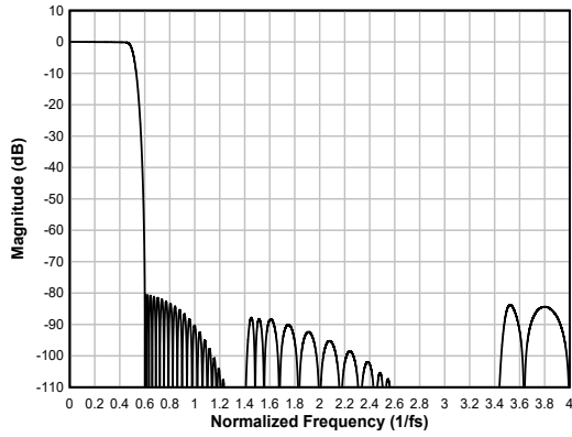
图 6-67. 线性相位内插滤波器幅度响应
