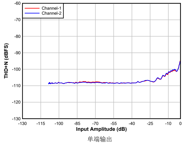
图 5-20. DAC THD+N 级别与输入间的关系
