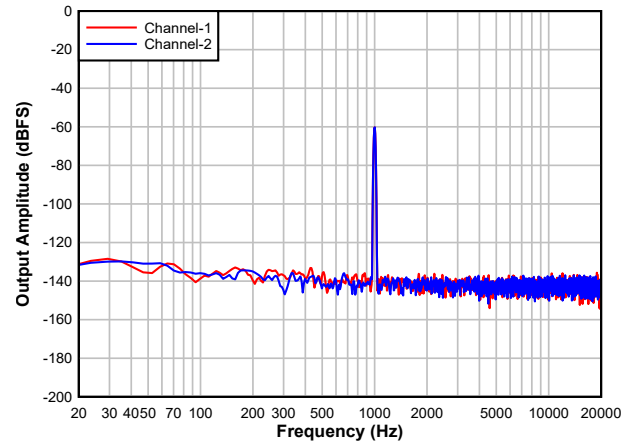
图 8-3. 具有-60dBFS 输入的 ADC FFT
