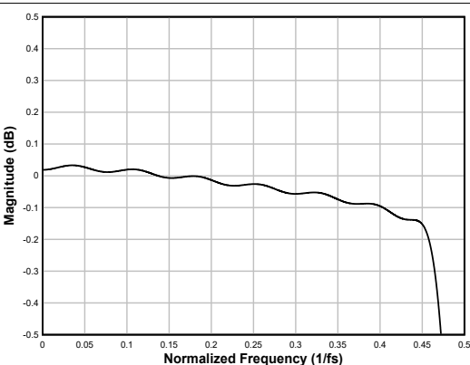
图 6-66. 线性相位内插滤波器通带纹波
