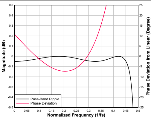
图 6-100. 超低延迟内插滤波器通带纹波和相位偏差
