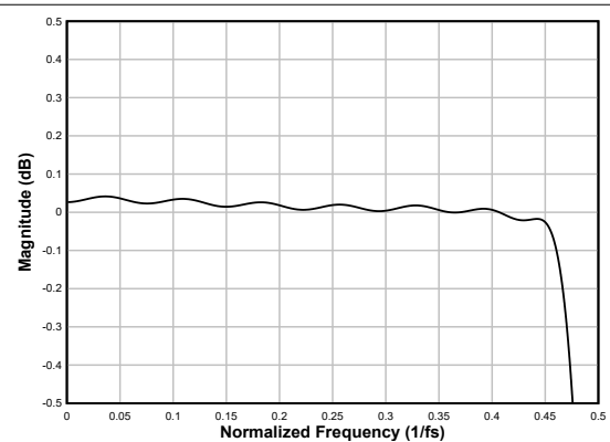
图 6-25. 线性相位抽取滤波器通带纹波
