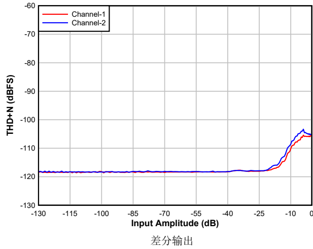
图 5-19. DAC THD+N 级别与输入间的关系
