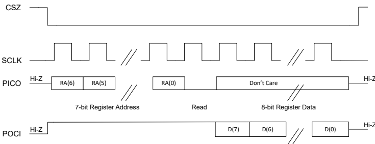
图 6-109. SPI 单字节读取传输
