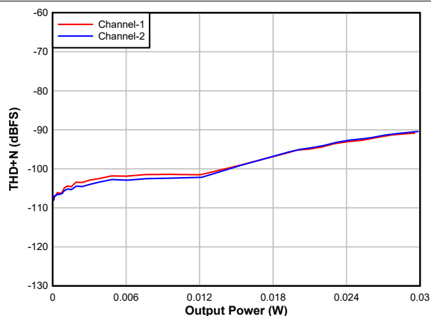
伪差分耳机输出, 16\Omega 负载
