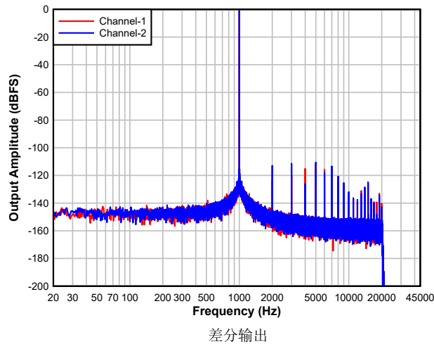
图 5-31. 具有 -1dBFS 输入的 DAC FFT
