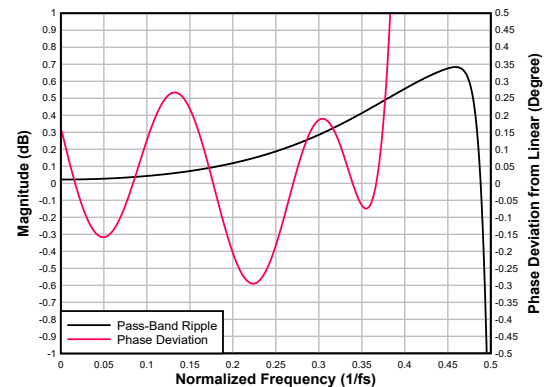
图 6-45. 低延迟抽取滤波器通带纹波和相位偏差
