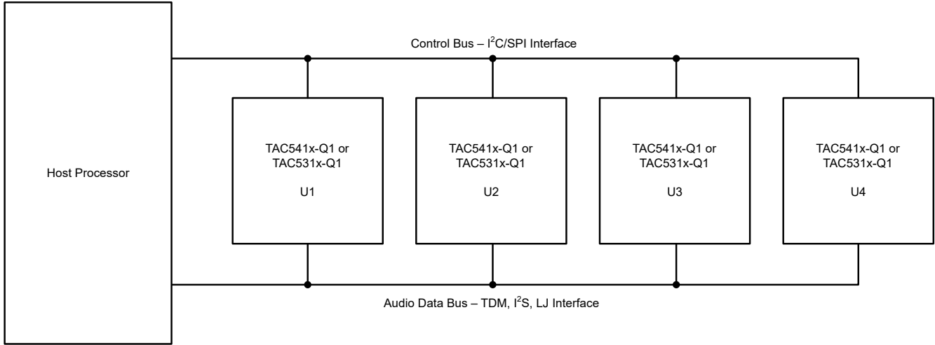
图 6-14. 多个 TAC5412-Q1 器件具有共享控制和音频数据总线
