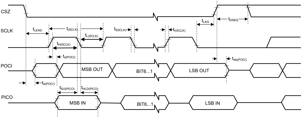
图 5-2. SPI 时序图
