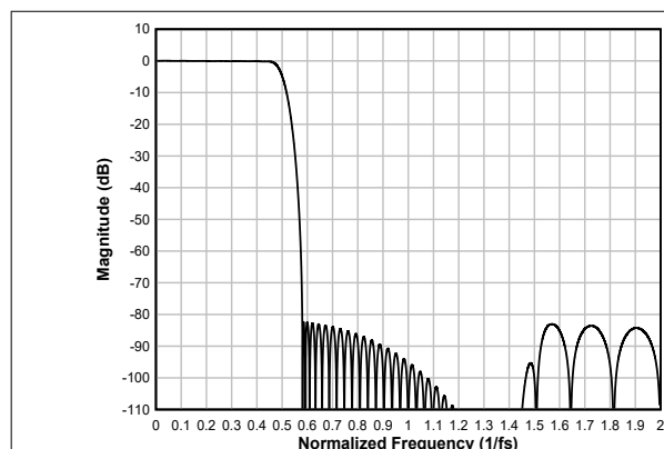
图 6-75. 线性相位内插滤波器幅度响应
