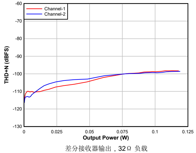
图 5-22. DAC THD+N 级别与输出功率间的关系
