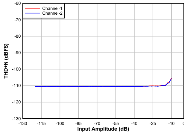
图 8-2. ADC THD+N 级别与输入间的关系
