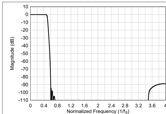
图 6-97. 超低延迟内插滤波器幅度响应
