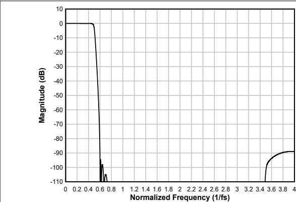
图 6-83. 低延迟内插滤波器幅度响应
