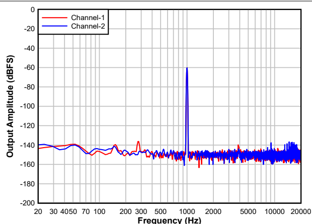
图 8-7. 具有-60dBFS 输入的 DAC FFT
