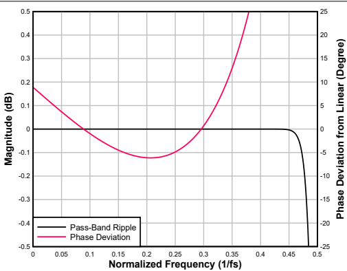
图 6-102. 超低延迟内插滤波器通带纹波和相位偏差
