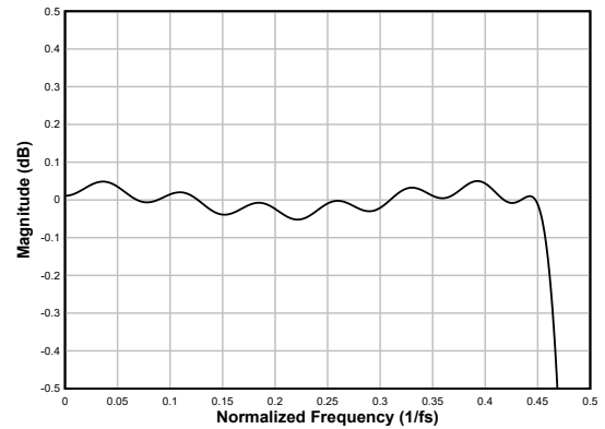
图 6-33. 线性相位抽取滤波器通带纹波
