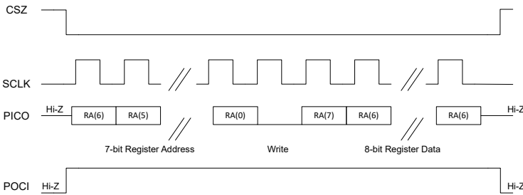
图 6-108. SPI 单字节写入传输
