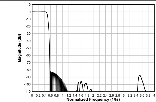
图 6-34. 线性相位抽取滤波器幅度响应
