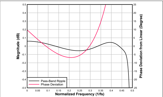
图 6-61. 超低延迟抽取滤波器通带纹波和相位偏差
