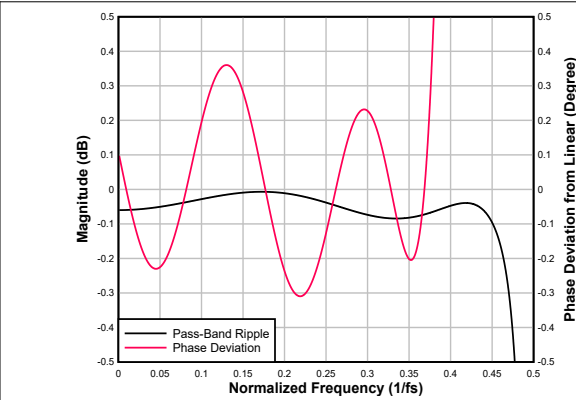
图 6-84. 低延迟内插滤波器通带纹波和相位偏差
