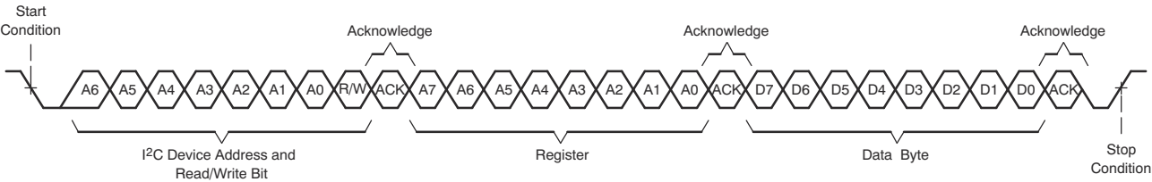
图 6-104. I²C 单字节写入传输
