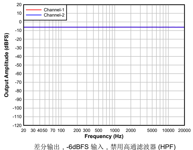
图 5-34. DAC 频率响应
