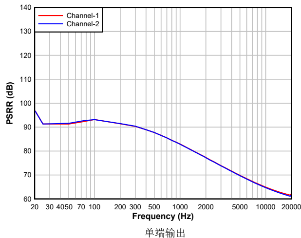
图 5-33. DAC PSRR 与频率间的关系
