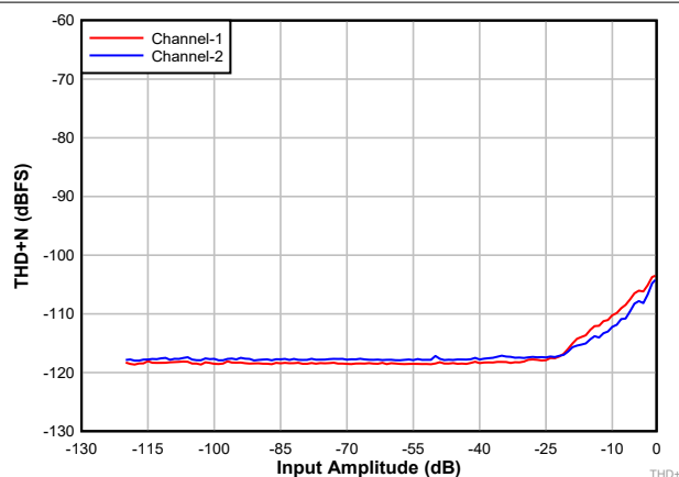
图 8-6. DAC THD+N 级别与输入间的关系
