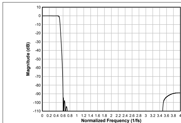
图 6-87. 低延迟内插滤波器幅度响应
