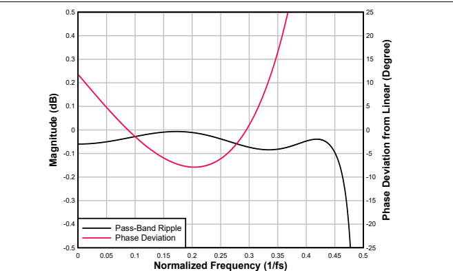
图 6-96. 超低延迟内插滤波器通带纹波和相位偏差
