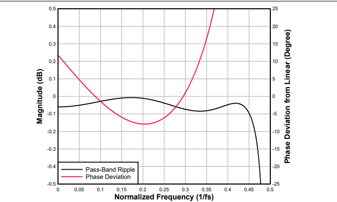
图 6-94. 超低延迟内插滤波器通带纹波和相位偏差
