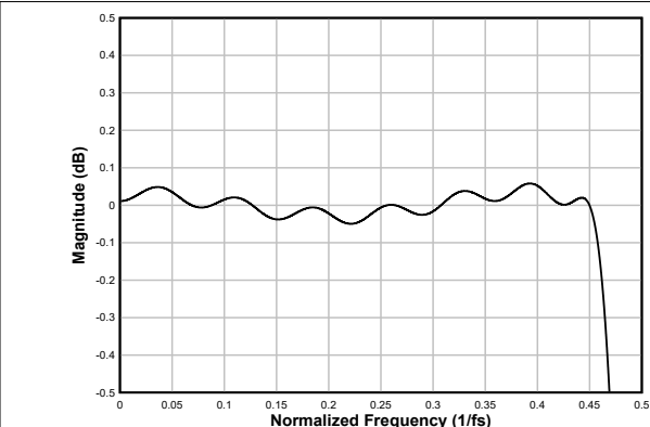
图 6-35. 线性相位抽取滤波器通带纹波
