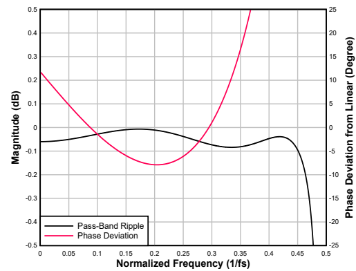
图 6-98. 超低延迟内插滤波器通带纹波和相位偏差
