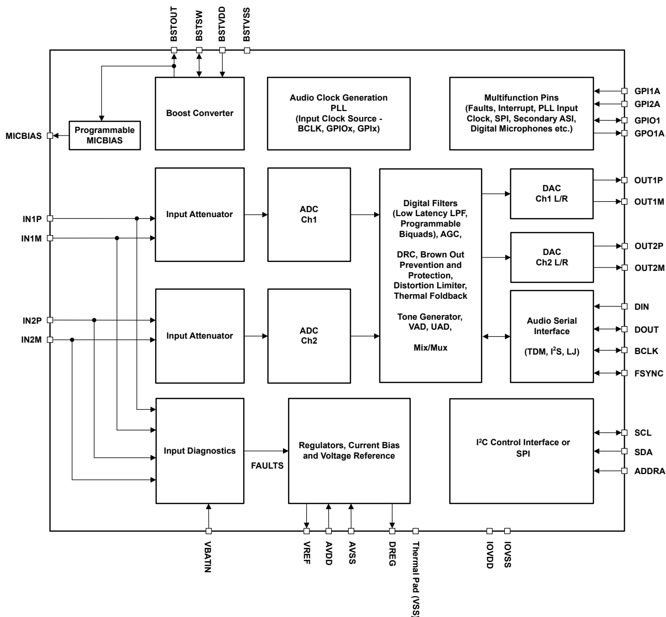
图 6-1. 功能方框图
