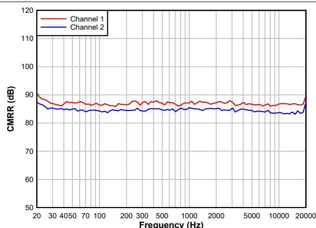
图 5-15. ADC CMRR 与频率间的关系
