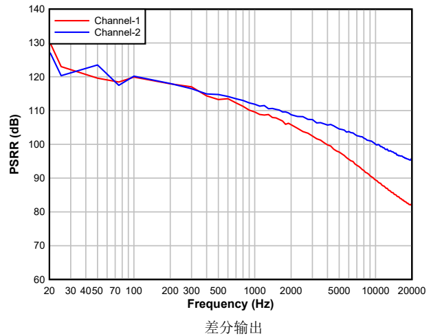
图 5-32. DAC PSRR 与频率间的关系
