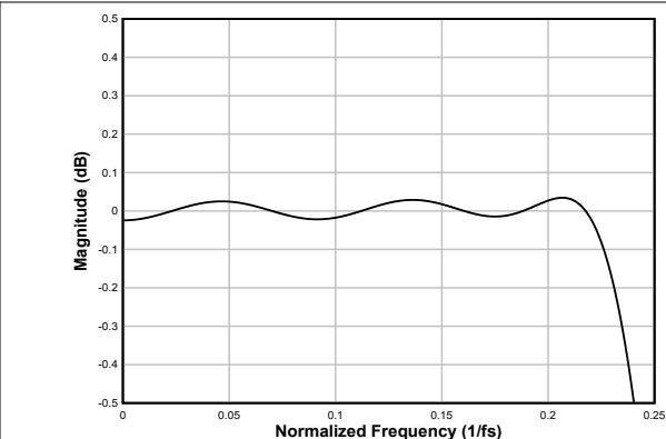
图 6-37. 线性相位抽取滤波器通带纹波
