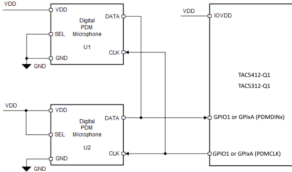
图 6-19. TAC5412-Q1 的数字 PDM 麦克风连接图
