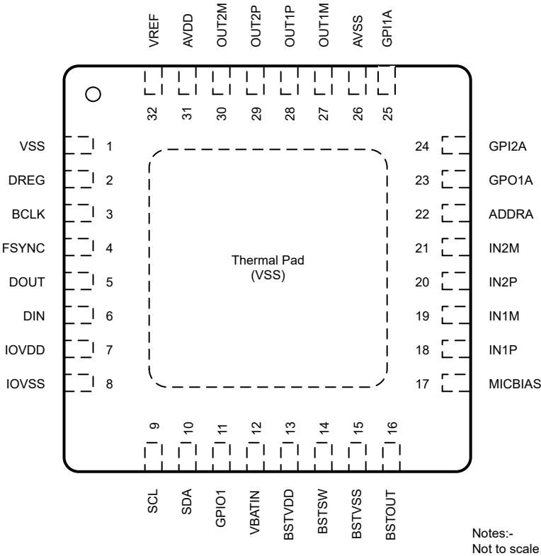
图 4-1. TAC5412-Q1 RTV 封装，32 引脚 WQFN（带有外露散热焊盘），顶视图
