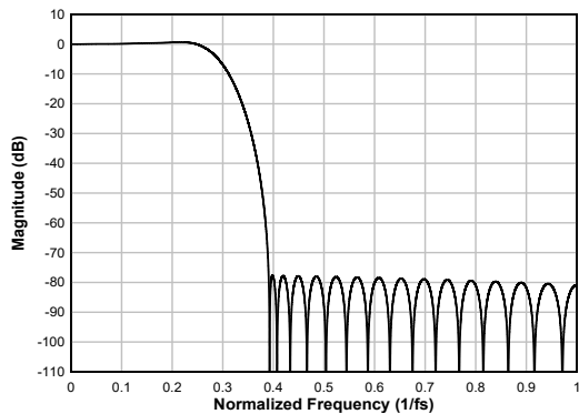
图 6-46. 线性相位内插滤波器幅度响应
