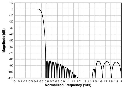
图 6-44. 线性相位内插滤波器幅度响应
