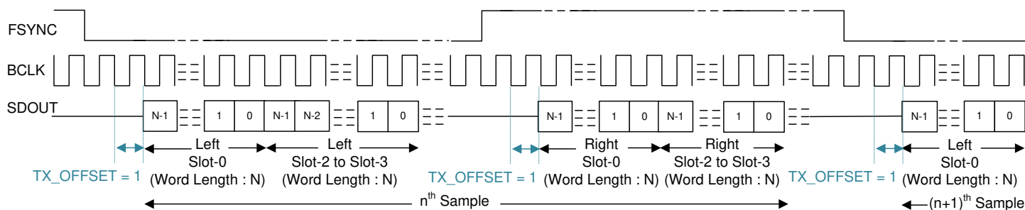
图 6-7. I²S 协议时序 (PASI_TX_OFFSET = 1)
