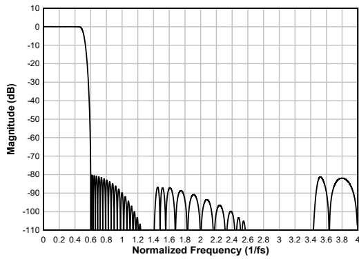
图 6-22. 线性相位抽取滤波器幅度响应
