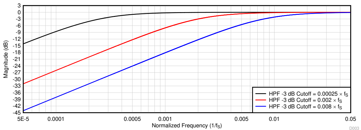
图 6-35. HPF 滤波器频率响应图
