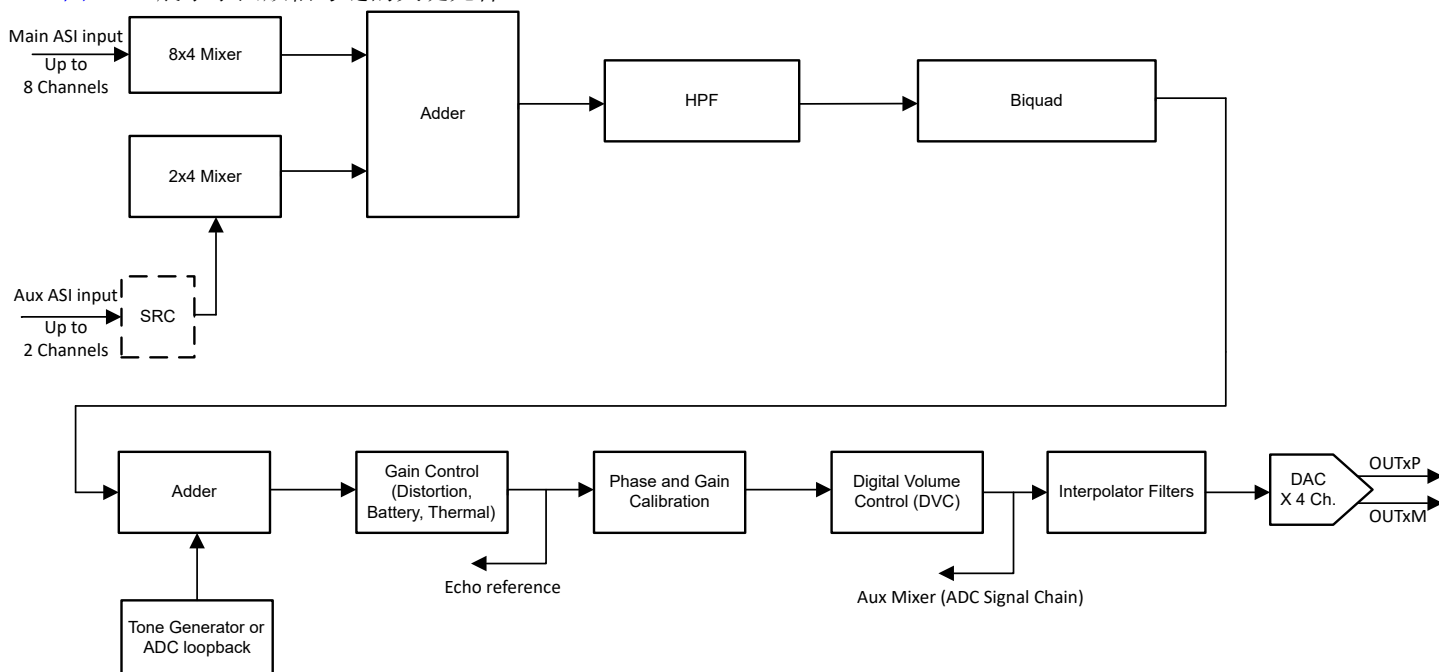
图 6-63. DAC 信号链处理流程图
