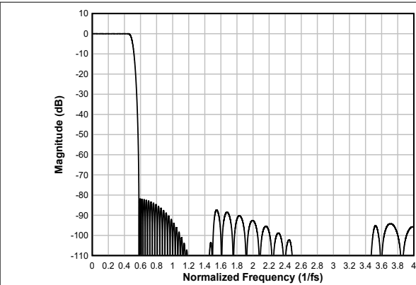
图 6-69. 线性相位内插滤波器幅度响应
