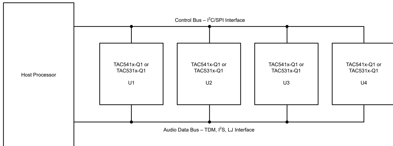
图 6-14. 多个 TAC5312-Q1 器件具有共享控制和音频数据总线
