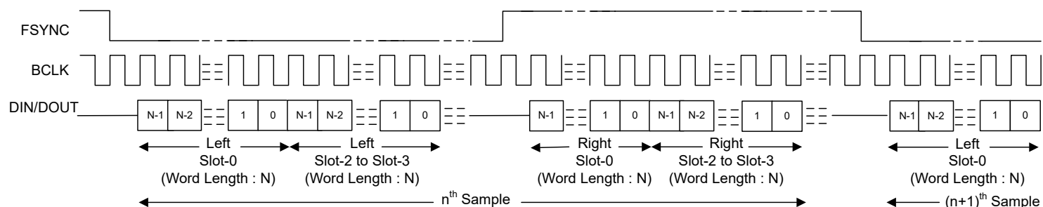
图 6-9. I²S 协议时序 (PASI_TX_OFFSET = 0 且 PASI_BCLK_POL = 1)
