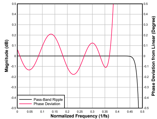
图 6-92. 低延迟内插滤波器通带纹波和相位偏差
