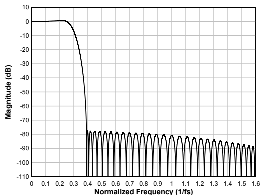
图 6-79. 线性相位内插滤波器幅度响应
