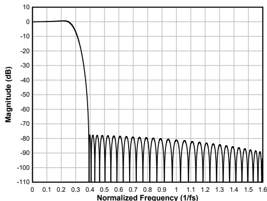
图 6-77. 线性相位内插滤波器幅度响应
