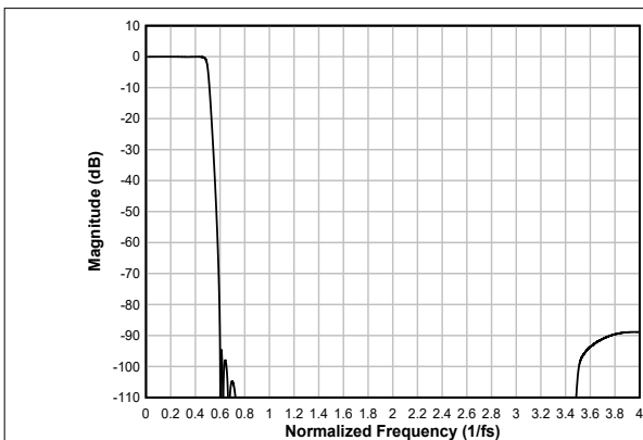
图 6-87. 低延迟内插滤波器幅度响应
