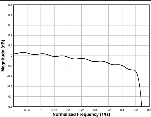
图 6-68. 线性相位内插滤波器通带纹波
