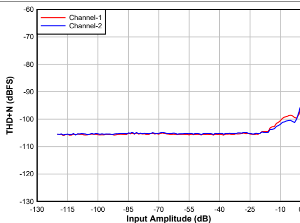
图 5-20. DAC THD+N 级别与输入间的关系
