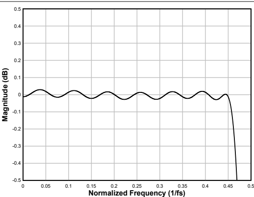
图 6-70. 线性相位内插滤波器通带纹波
