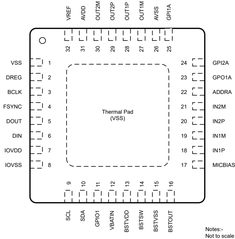
图 4-1. TAC5312-Q1 RTV 封装，32 引脚 WQFN (带有外露散热焊盘)，顶视图
