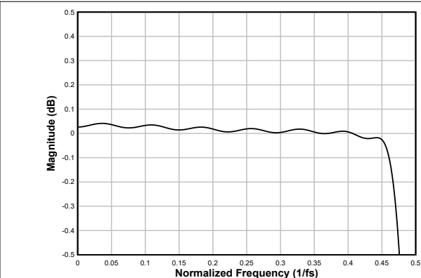
图 6-25. 线性相位抽取滤波器通带纹波
