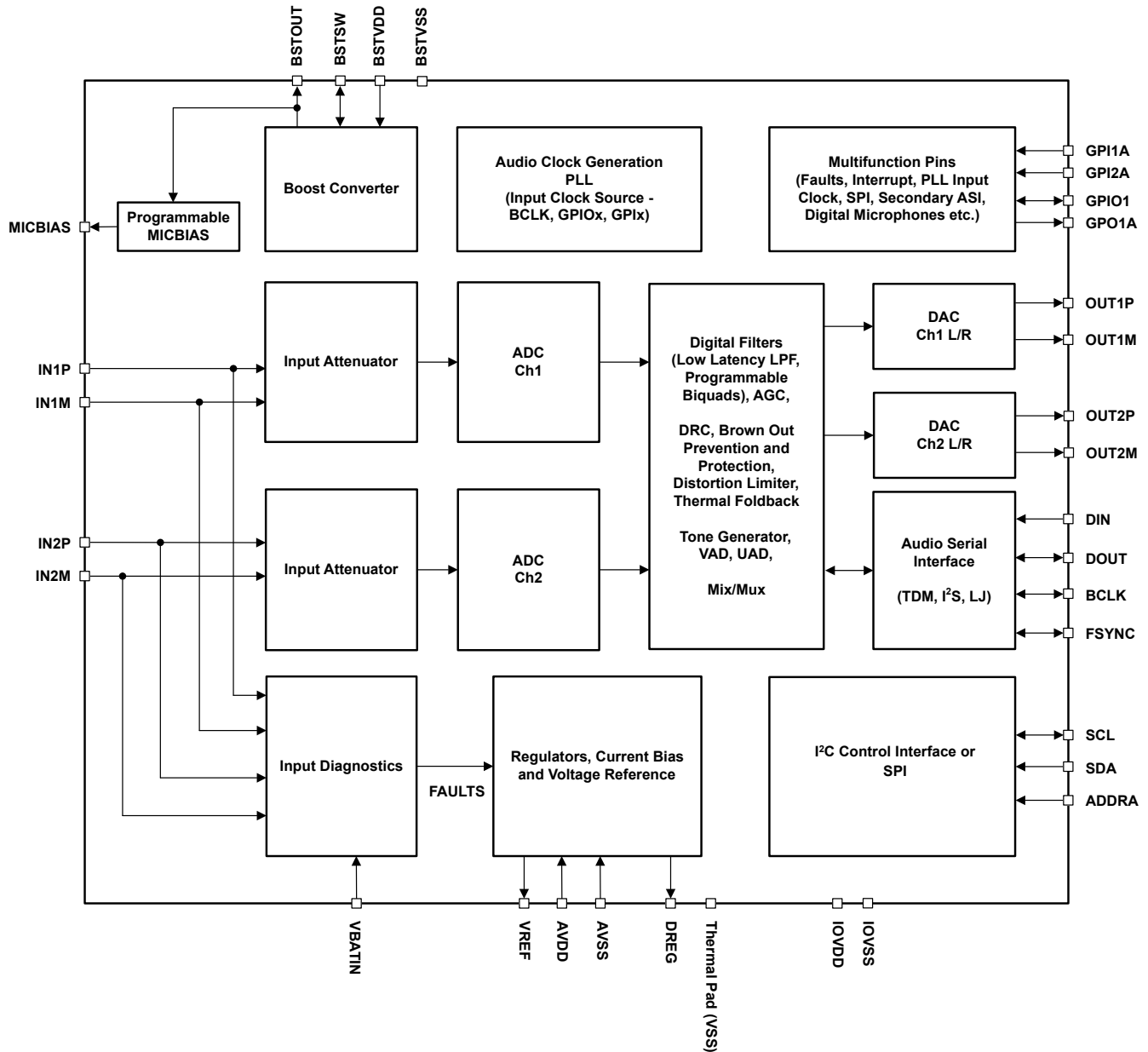
图 6-1. 功能方框图
