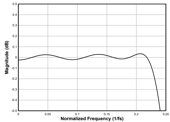
图 6-37. 线性相位抽取滤波器通带纹波
