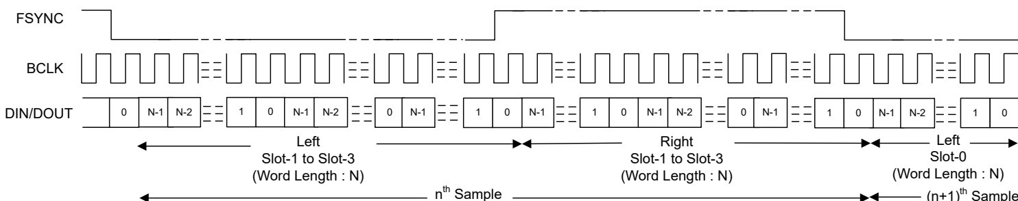
图 6-8. I²S 协议时序 (无空闲 BCLK 周期, PASI_TX_OFFSET = 0)
