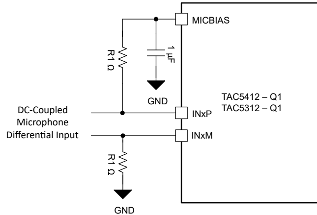
图 6-15. 直流耦合麦克风或线路差分输入连接
