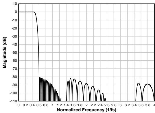
图 6-28. 线性相位抽取滤波器幅度响应
