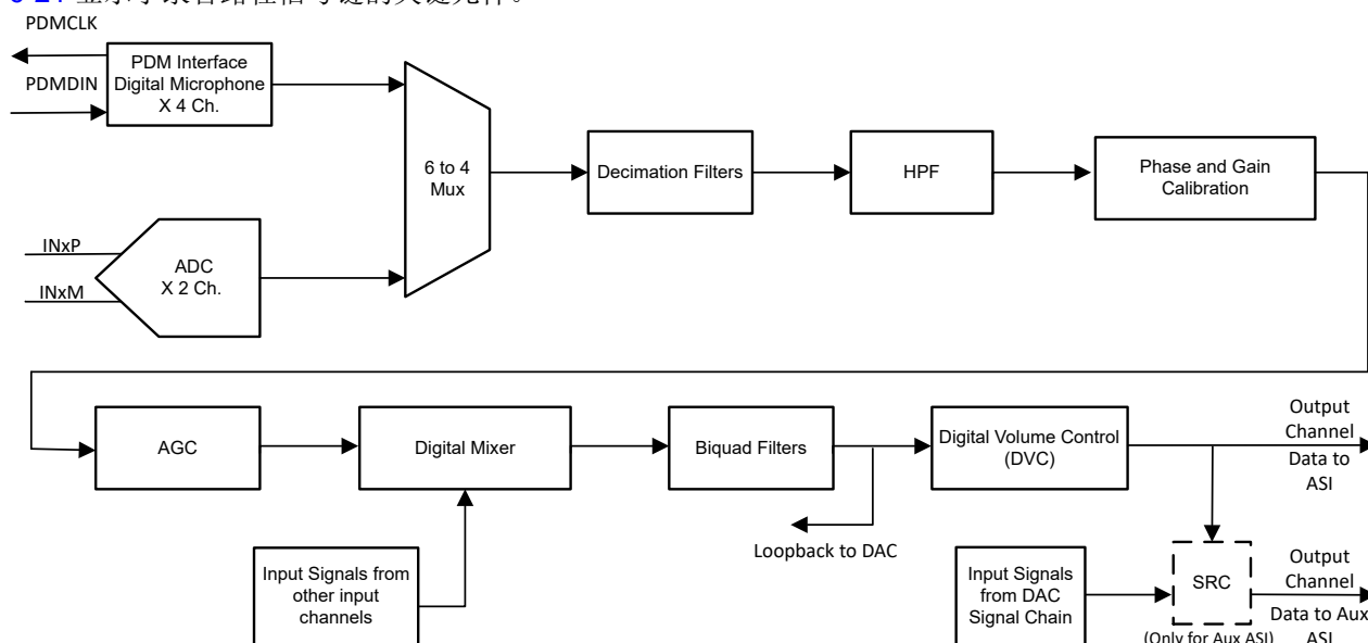
图 6-21. ADC 信号链处理流程图
