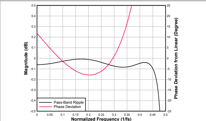
图 6-96. 超低延迟内插滤波器通带纹波和相位偏差
