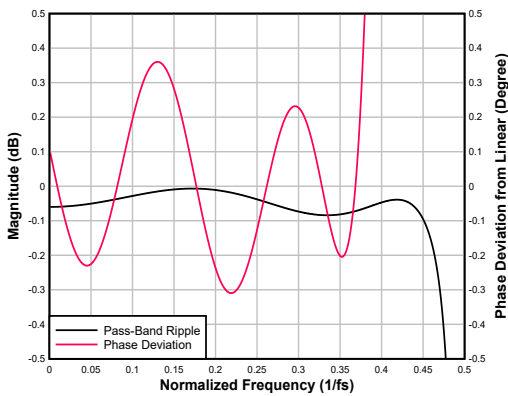
图 6-88. 低延迟内插滤波器通带纹波和相位偏差
