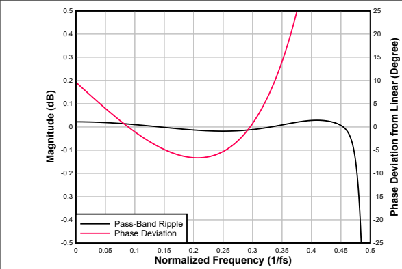
图 6-59. 超低延迟抽取滤波器通带纹波和相位偏差
