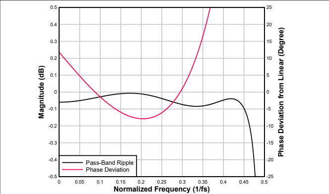
图 6-94. 超低延迟内插滤波器通带纹波和相位偏差
