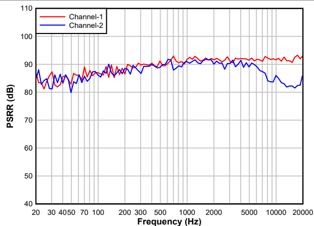
图 5-16. ADC PSRR 与频率间的关系
