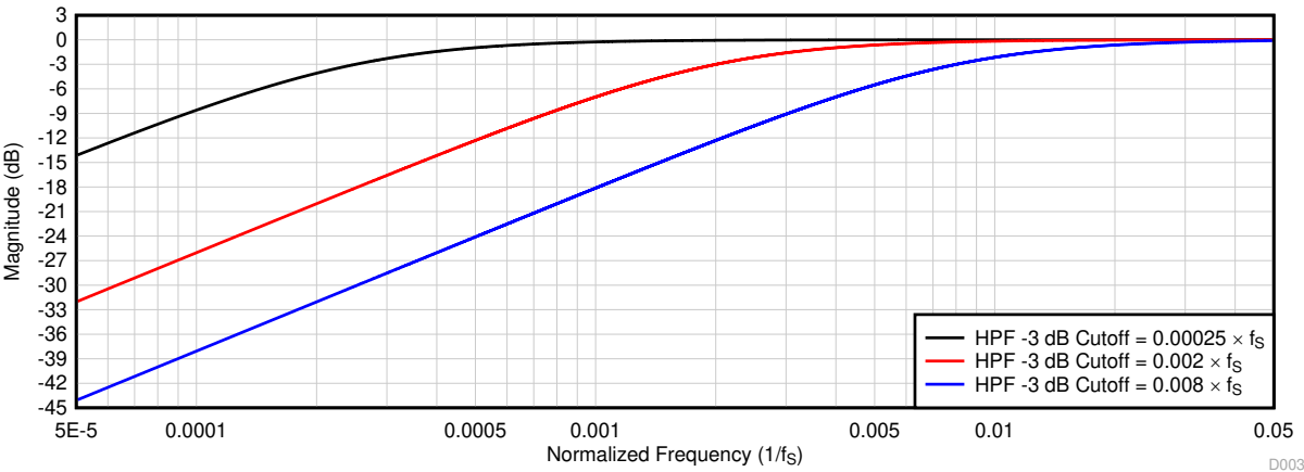
图 6-64. HPF 滤波器频率响应图
