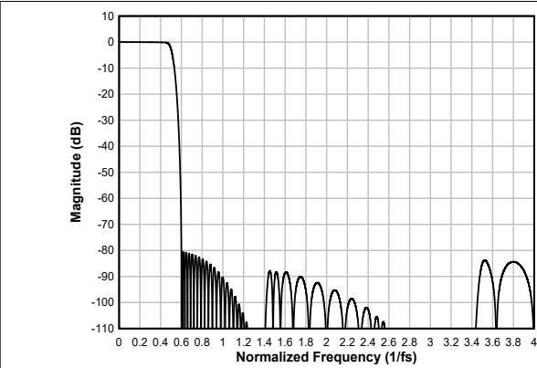
图 6-67. 线性相位内插滤波器幅度响应
