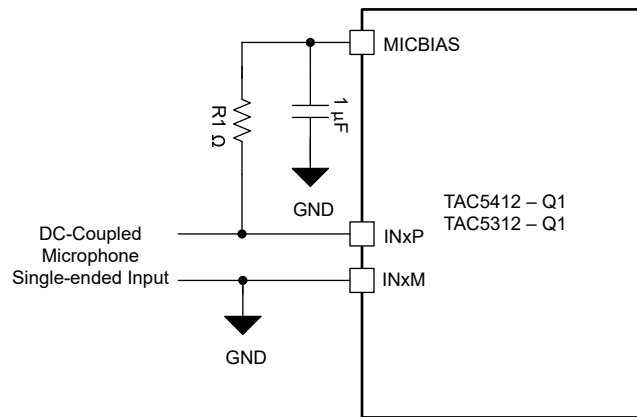
图 6-16. 直流耦合麦克风或线路单端输入连接
