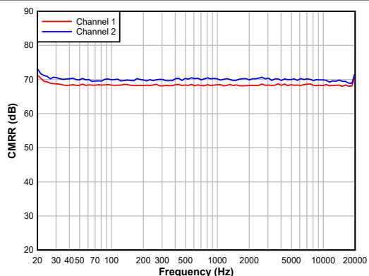
图 5-15. ADC CMRR 与频率间的关系
