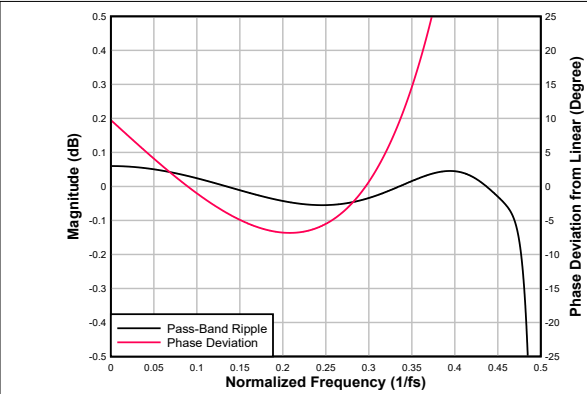
图 6-61. 超低延迟抽取滤波器通带纹波和相位偏差
