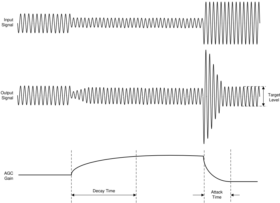
图 6-62. AGC 特性
