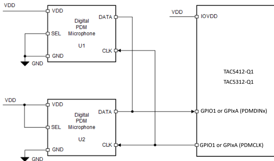
图 6-19. TAC5312-Q1 的数字 PDM 麦克风连接图
