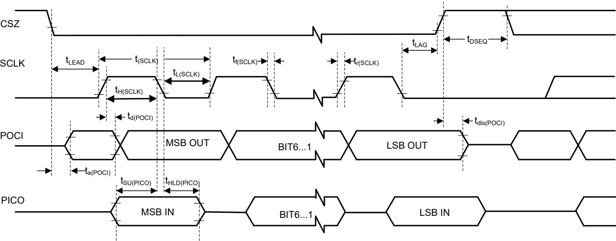
图 5-2. SPI 时序图
