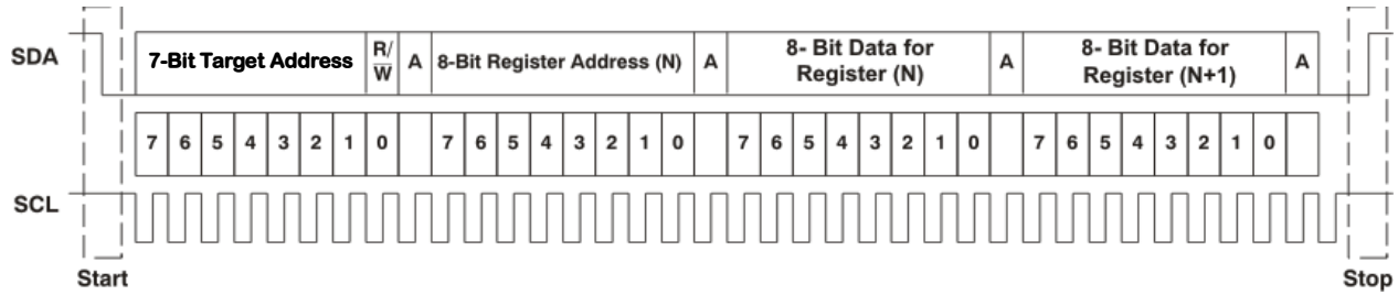
图 6-103. 典型的 I²C 序列
