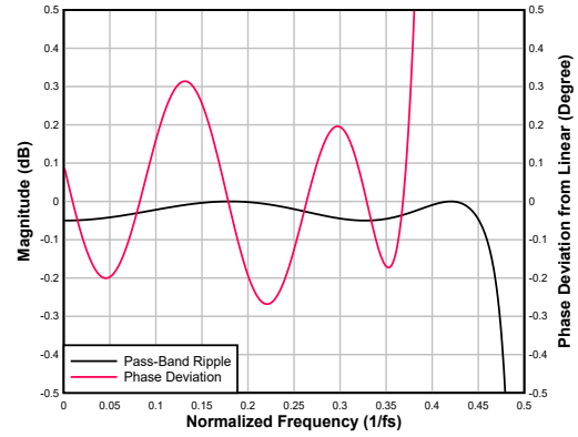
图 6-90. 低延迟内插滤波器通带纹波和相位偏差
